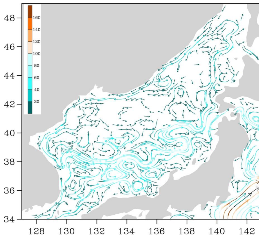
Рис. 3-1 Поверхностные течения Японского моря, 05 января 2014 г.
