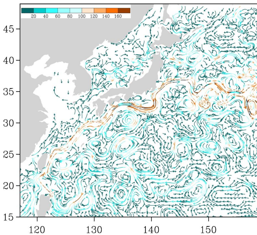
Рис. 3-4 Поверхностные течения западной части Тихого океана, 5 января 2014 г.
