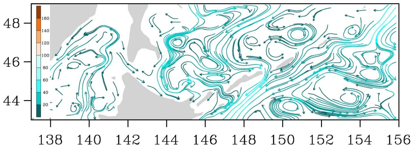
Рис. 3-7 Поверхностные течения, пролив Лаперуза, 5 января 2014 г.
