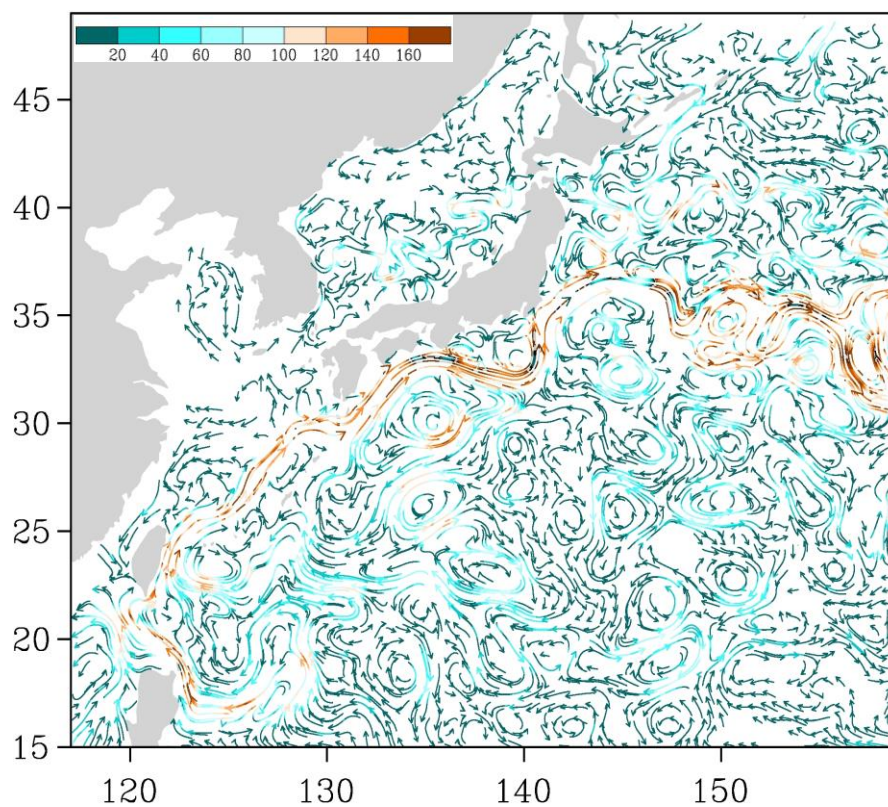
Рис. 3-5 Поверхностные течения западной части Тихого океана, 15 января 2014 г.
