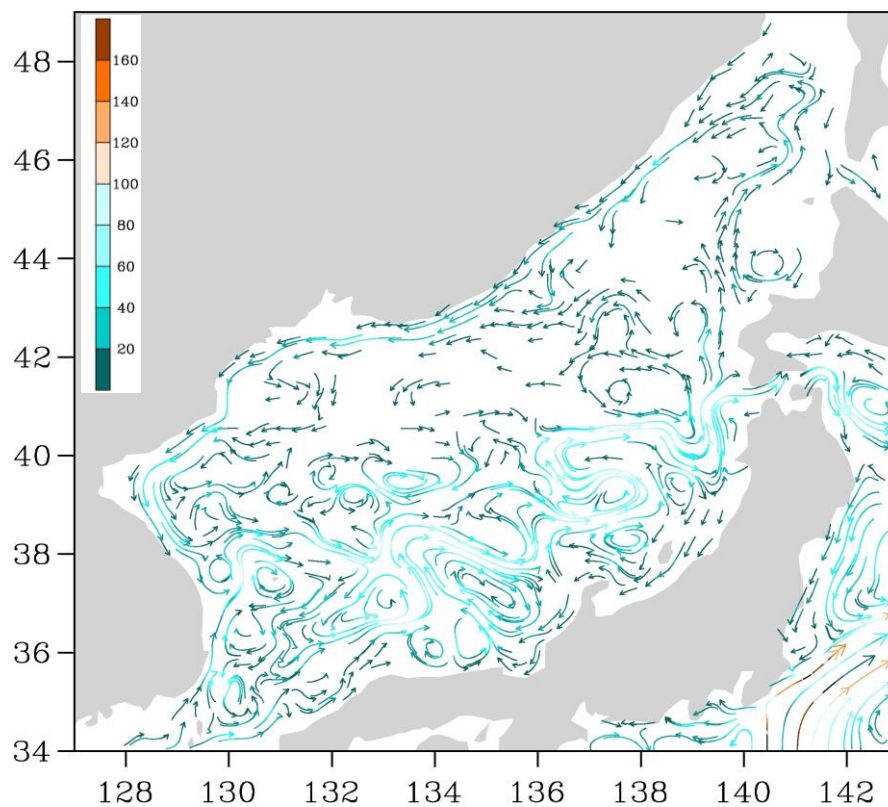
Рис. 3-2 Поверхностные течения Японского моря, 15 января 2014 г.
