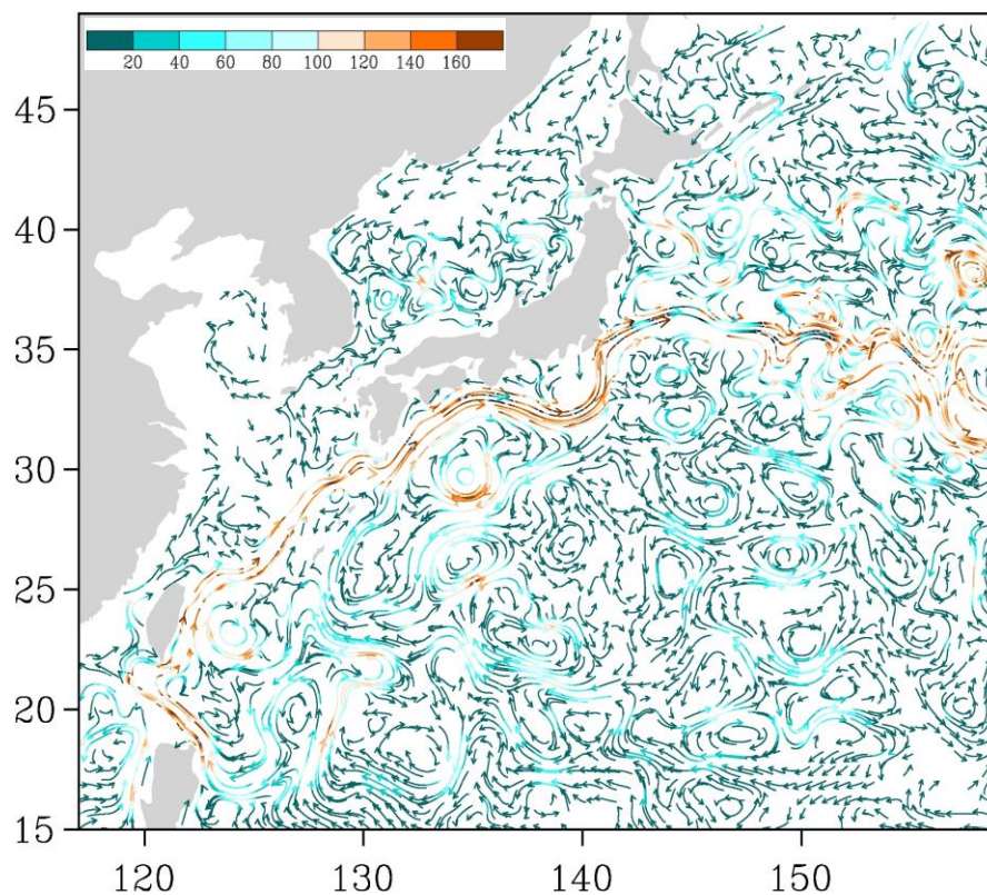
Рис. 3-6 Поверхностные течения западной части Тихого океана, 25 января 2014 г.
