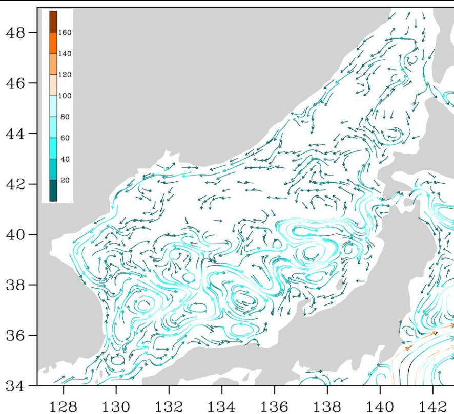
Рис. 3-3 Поверхностные течения Японского моря, 25 января 2014 г.
