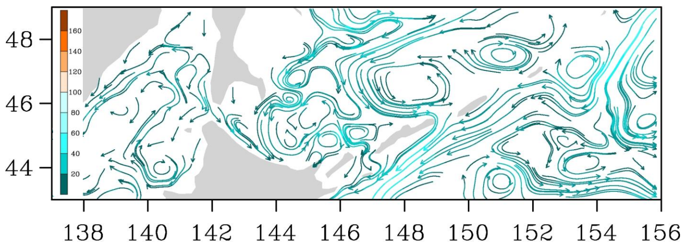
Рис. 3-9 Поверхностные течения, пролив Лаперуза, 25 января 2014 г.
