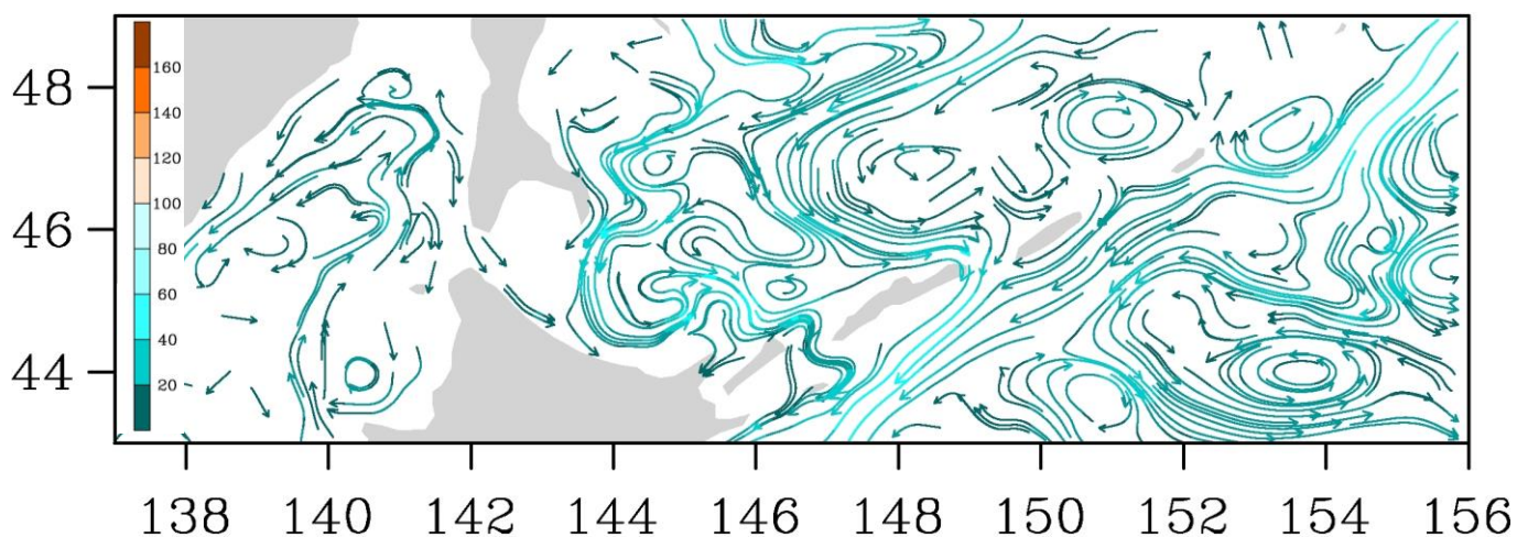
Рис. 3-8 Поверхностные течения, пролив Лаперуза, 15 января 2014 г.
