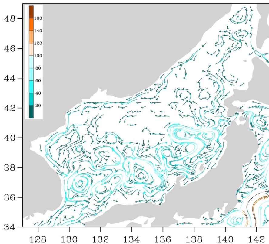
Рис. 3-2 Поверхностные течения Японского моря, 15 февраля 2014 г.
