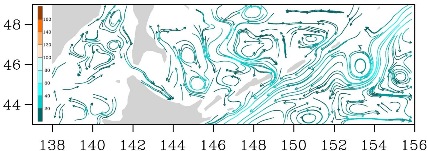
Рис. 3-9 Поверхностные течения, пролив Лаперуза, 25 февраля 2014 г.
