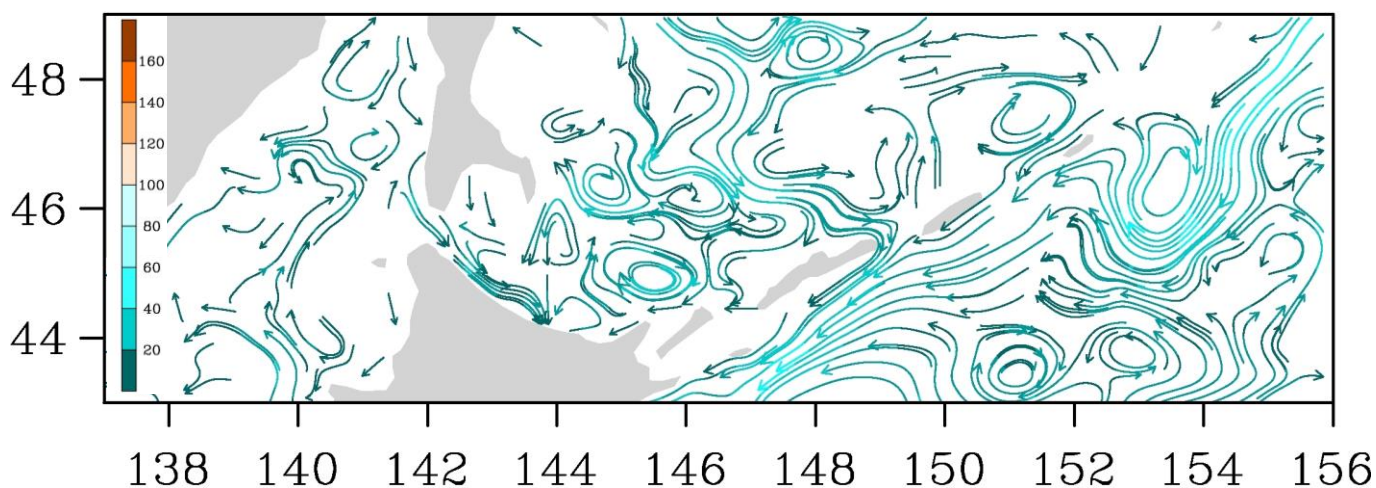
Рис. 3-8 Поверхностные течения, пролив Лаперуза, 15 февраля 2014 г.
