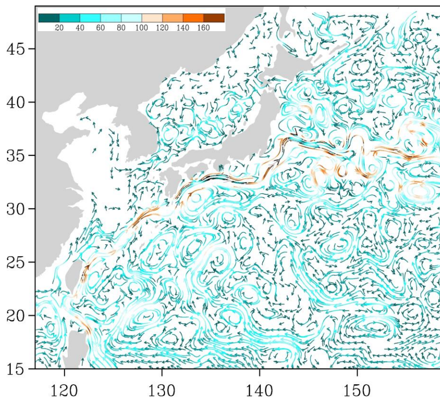
Рис. 3-6 Поверхностные течения западной части Тихого океана, 25 февраля 2014 г.
