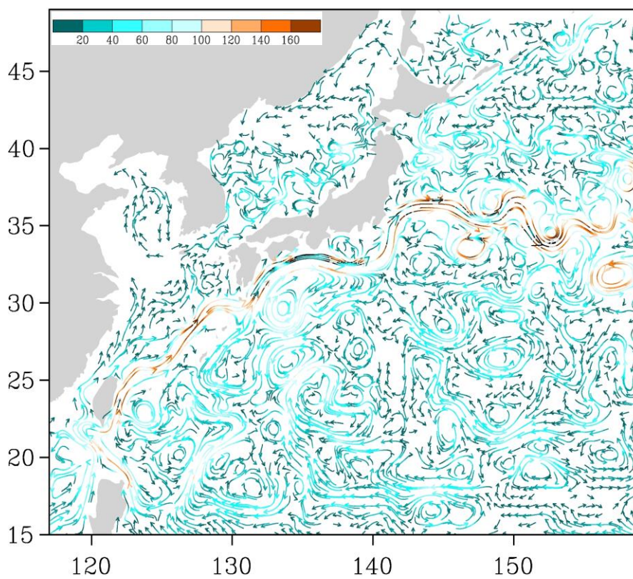
Рис. 3-4 Поверхностные течения западной части Тихого океана, 5 февраля 2014 г.
