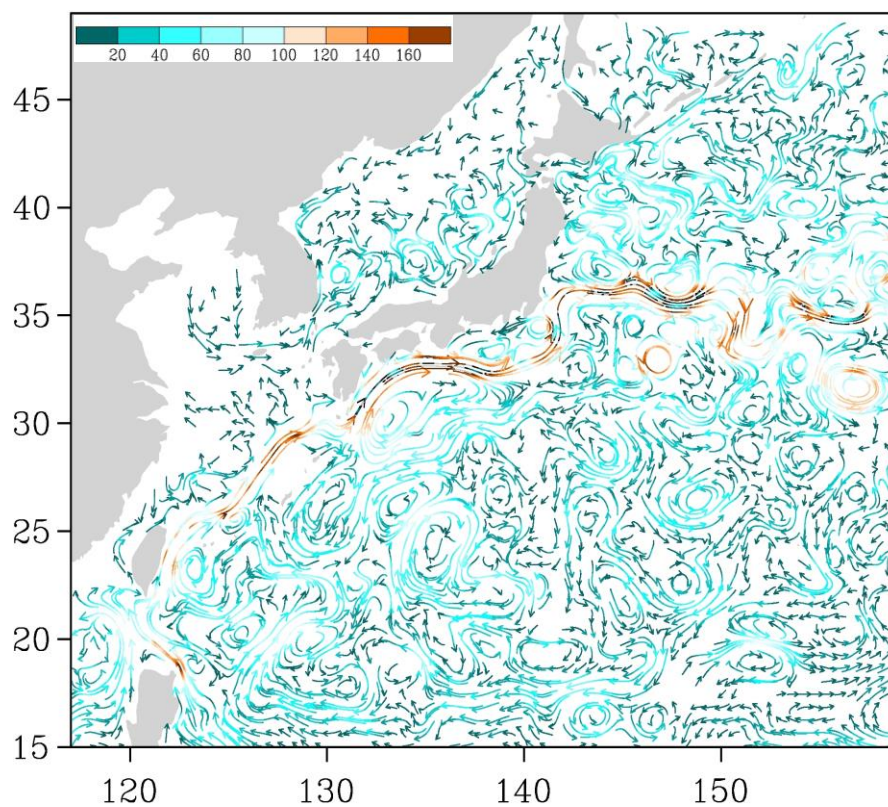
Рис. 3-5 Поверхностные течения западной части Тихого океана, 15 февраля 2014 г.
