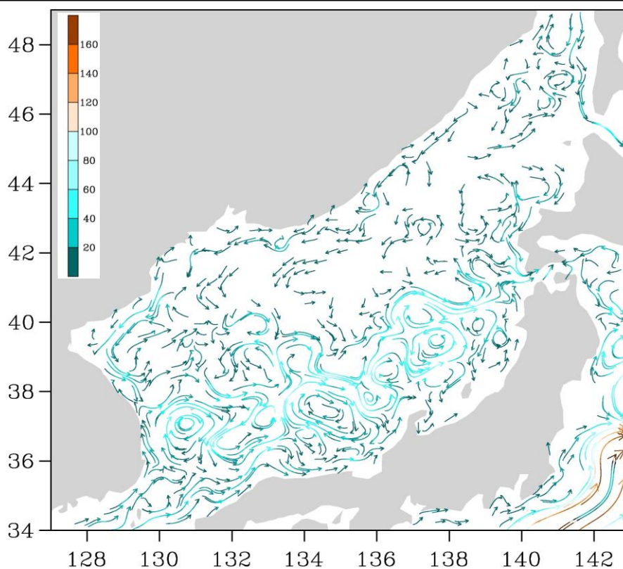
Рис. 3-3 Поверхностные течения Японского моря, 25 февраля 2014 г.
