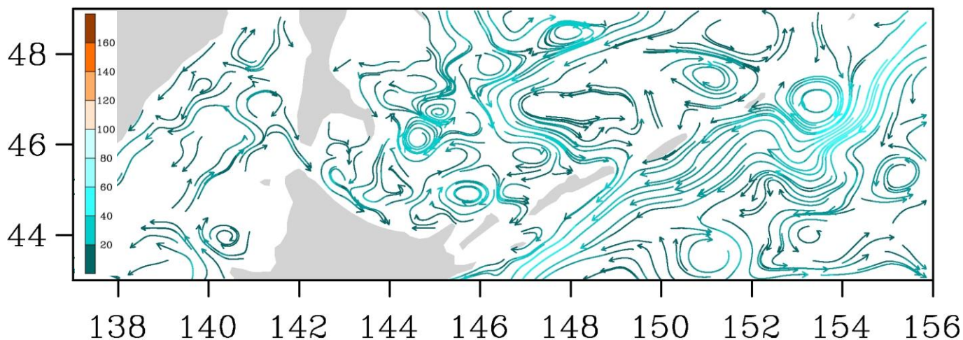
Рис. 3-7 Поверхностные течения, пролив Лаперуза, 5 февраля 2014 г.
