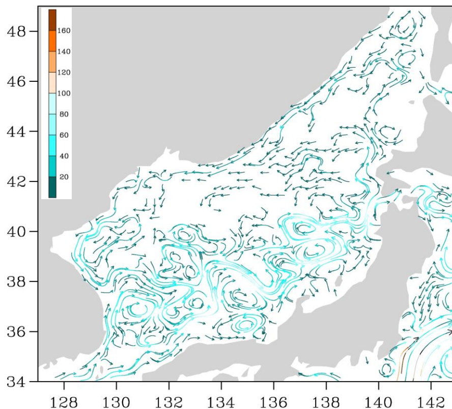
Рис. 3-1 Поверхностные течения Японского моря, 05 февраля 2014 г.
