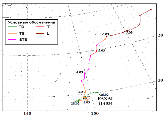
Рис. 5-2 Траектория ТЦ FAXAI (1403), возникшего в северо-западной части Тихого океана в феврале 2014 г.
