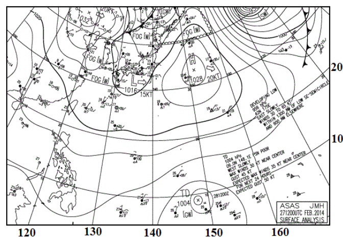
Рис. 5-2 Карта приземного анализа (JMA) за 12 ВСВ 27 февраля 2014 г.
