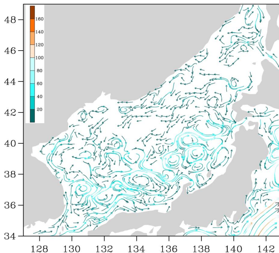
Рис. 3-1 Поверхностные течения Японского моря, 05 марта 2014 г.
