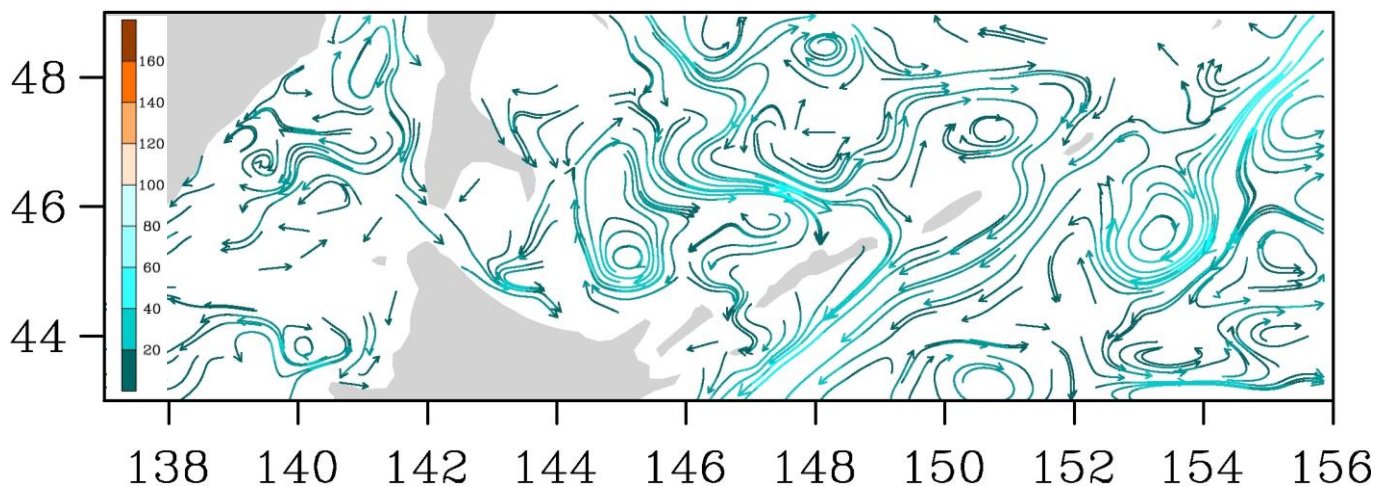
Рис. 3-7 Поверхностные течения, пролив Лаперуза, 5 марта 2014 г.
