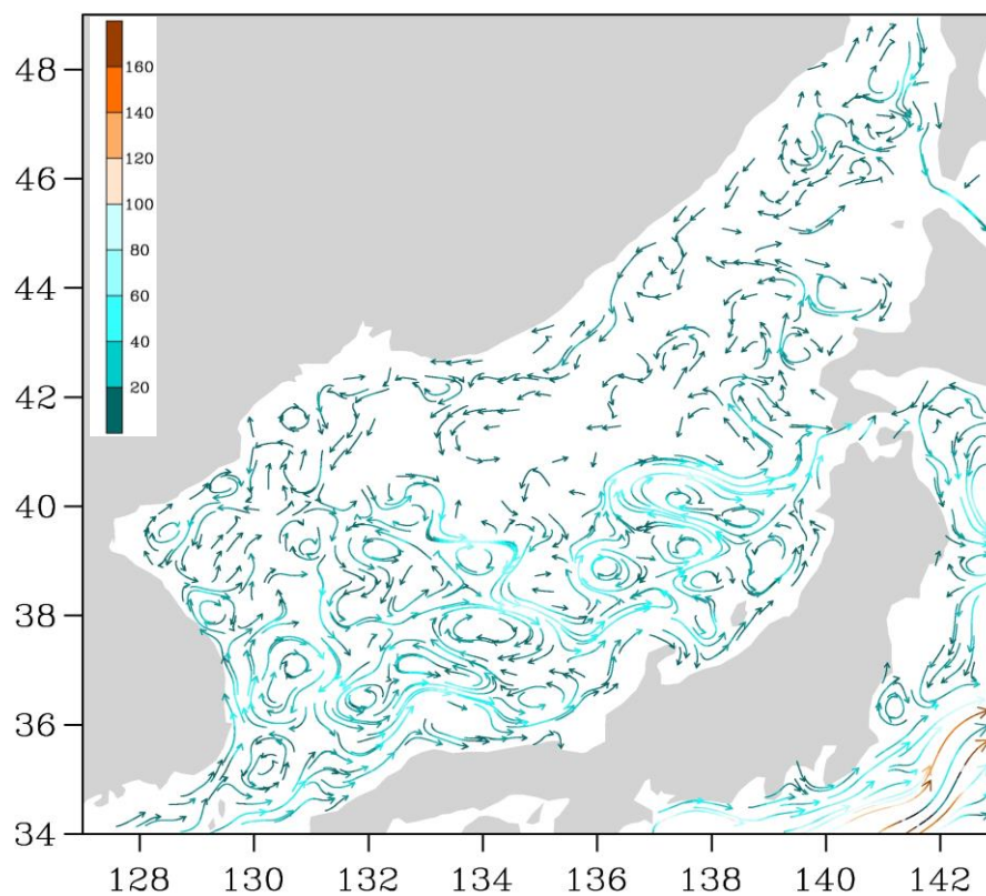
Рис. 3-2 Поверхностные течения Японского моря, 15 марта 2014 г.
