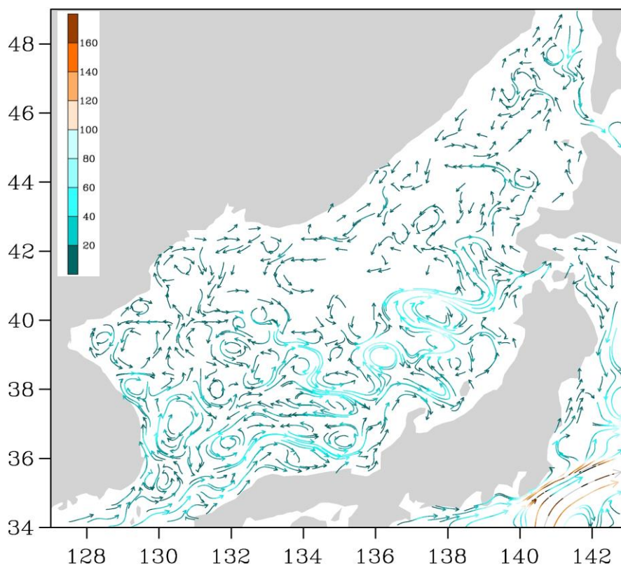
Рис. 3-3 Поверхностные течения Японского моря, 25 марта 2014 г.
