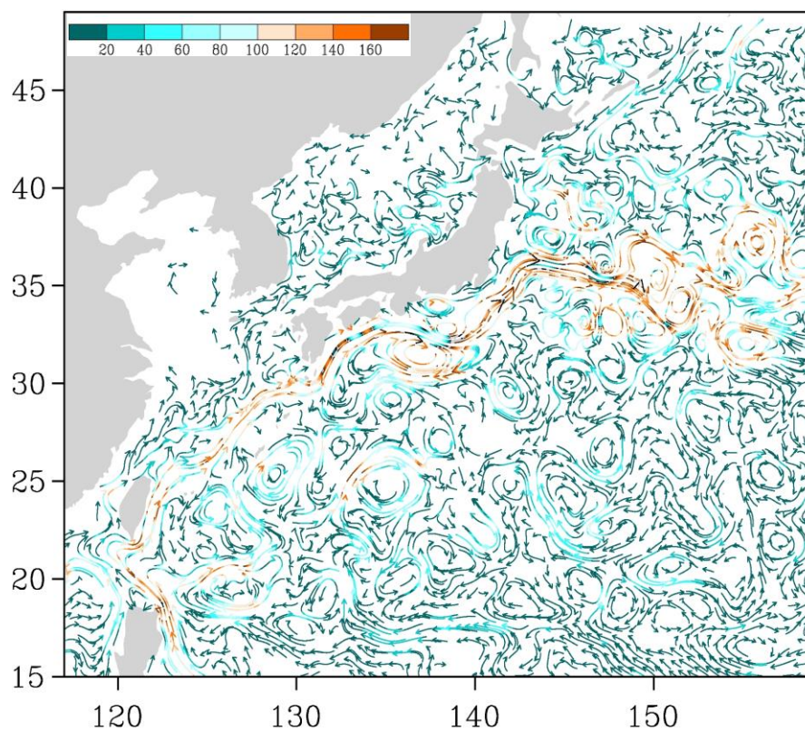
Рис. 3-5 Поверхностные течения западной части Тихого океана, 15 марта 2014 г.
