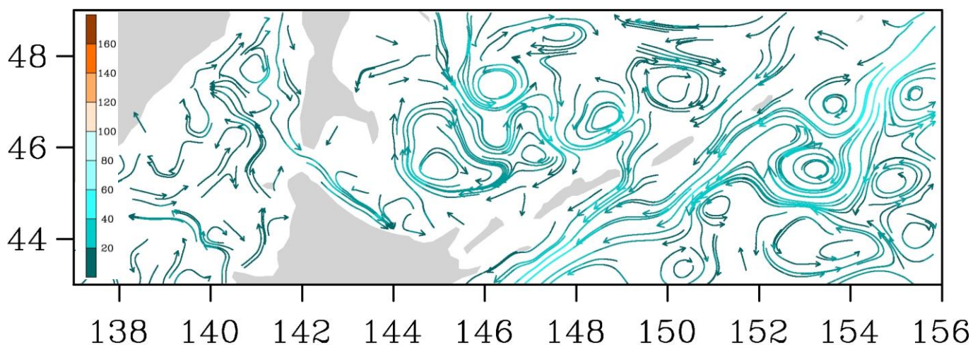
Рис. 3-9 Поверхностные течения, пролив Лаперуза, 25 марта 2014 г.
