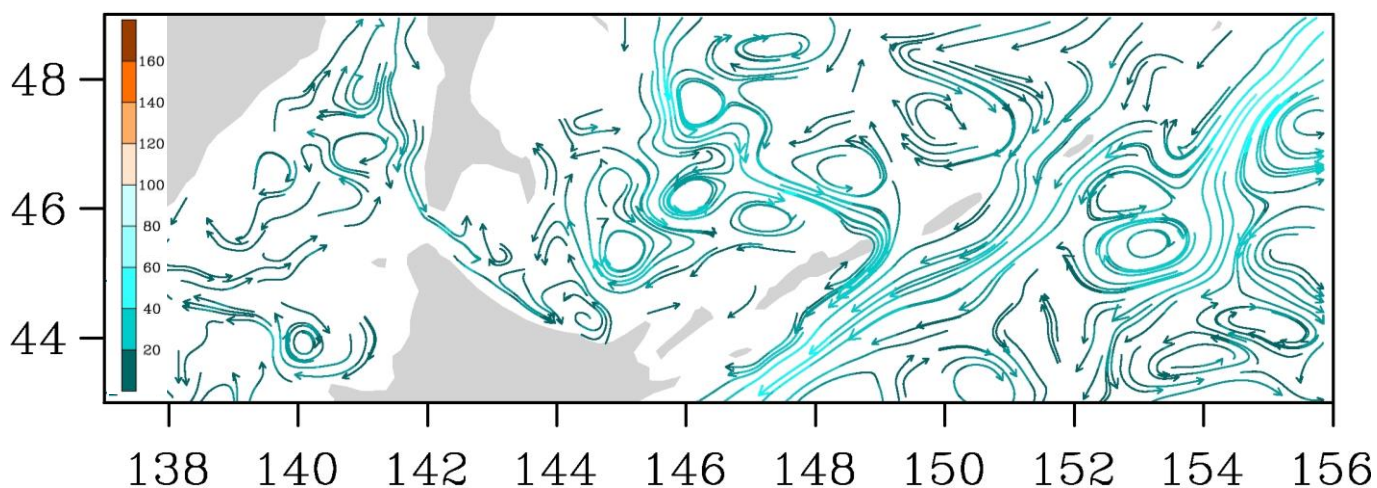
Рис. 3-8 Поверхностные течения, пролив Лаперуза, 15 марта 2014 г.
