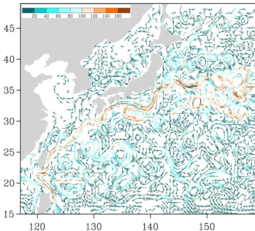
Рис. 3-6 Поверхностные течения западной части Тихого океана, 25 марта 2014 г.
