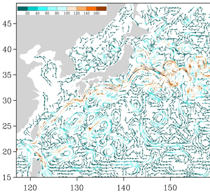
Рис. 3-4 Поверхностные течения западной части Тихого океана, 5 марта 2014 г.
