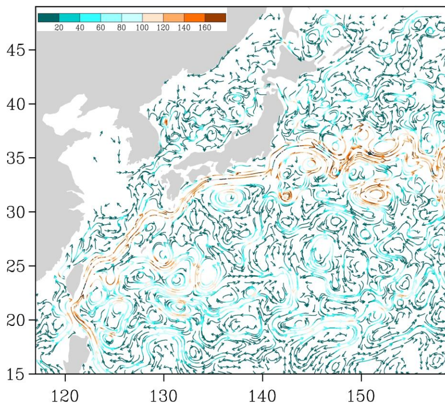
Рис. 3-5 Поверхностные течения западной части Тихого океана, 15 июня 2014 г.
