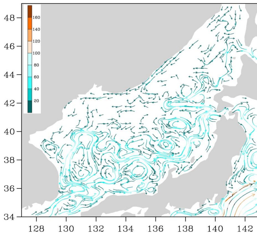
Рис. 3-2 Поверхностные течения Японского моря, 15 июня 2014 г.
