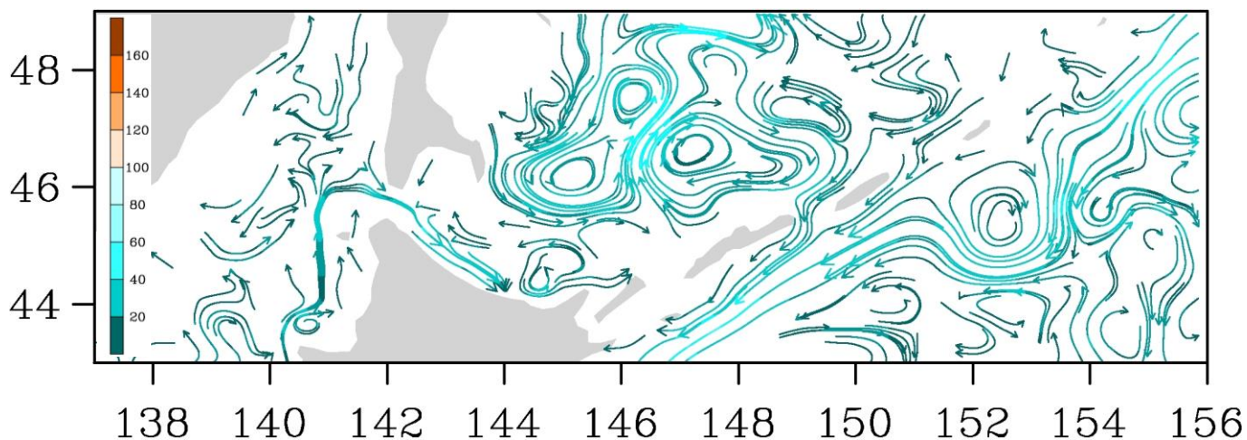
Рис. 3-7 Поверхностные течения, пролив Лаперуза, 5 июня 2014 г.
