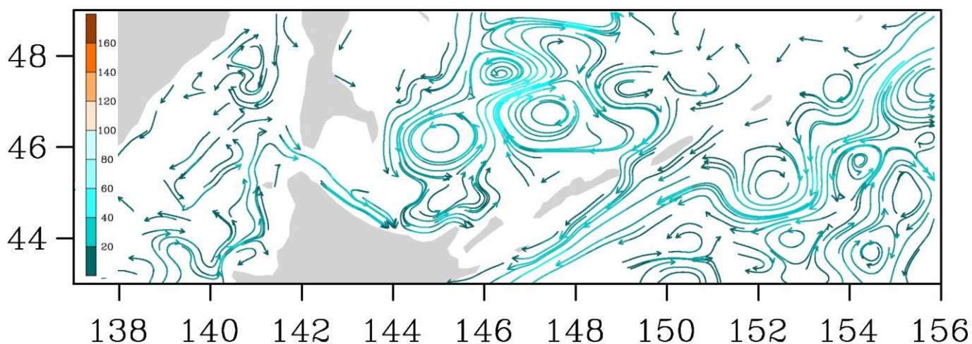
Рис. 3-8 Поверхностные течения, пролив Лаперуза, 15 июня 2014 г.
