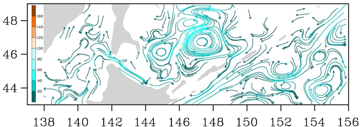
Рис. 3-9 Поверхностные течения, пролив Лаперуза, 25 июня 2014 г.
