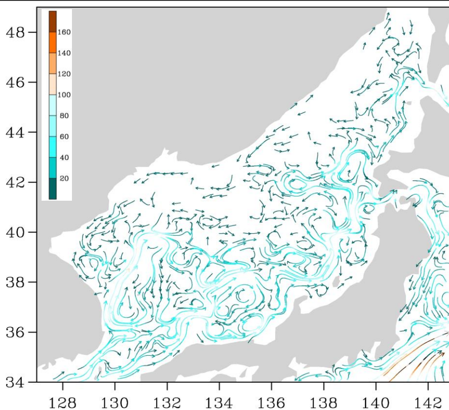
Рис. 3-3 Поверхностные течения Японского моря, 25 июня 2014 г.
