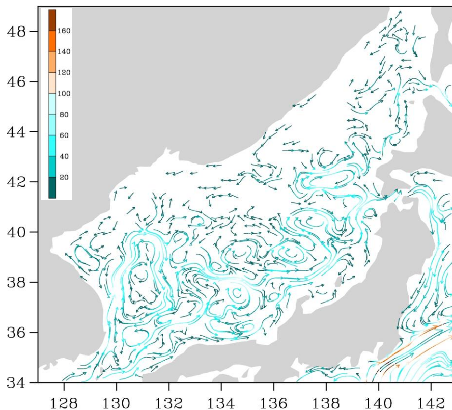
Рис. 3-1 Поверхностные течения Японского моря, 05 июня 2014 г.
