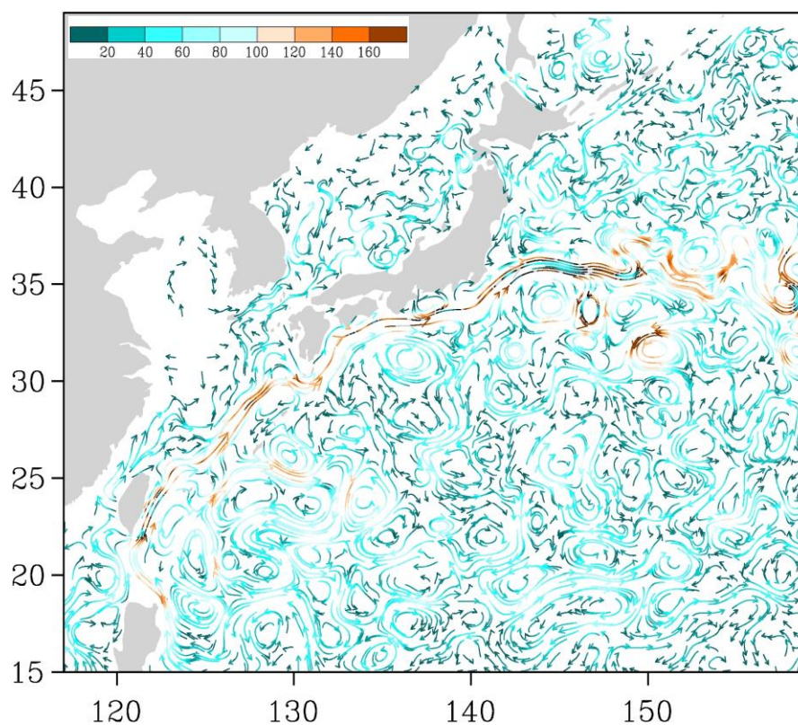
Рис. 3-6 Поверхностные течения западной части Тихого океана, 25 июня 2014 г.
