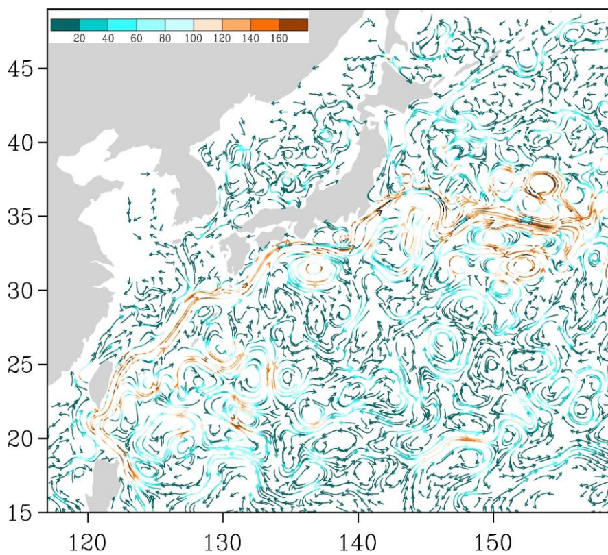
Рис. 3-4 Поверхностные течения западной части Тихого океана, 5 июня 2014 г.
