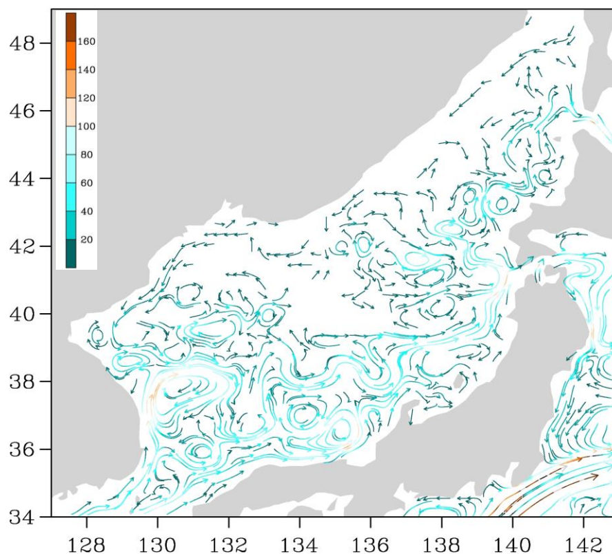
Рис. 3-1 Поверхностные течения Японского моря, 05 августа 2014 г.
