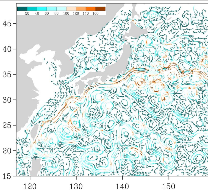
Рис. 3-5 Поверхностные течения западной части Тихого океана, 15 августа 2014 г.
