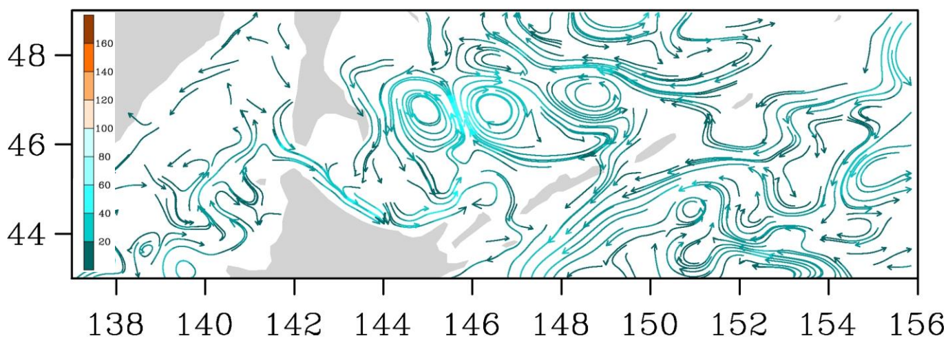
Рис. 3-9 Поверхностные течения, пролив Лаперуза, 25 августа 2014 г.
