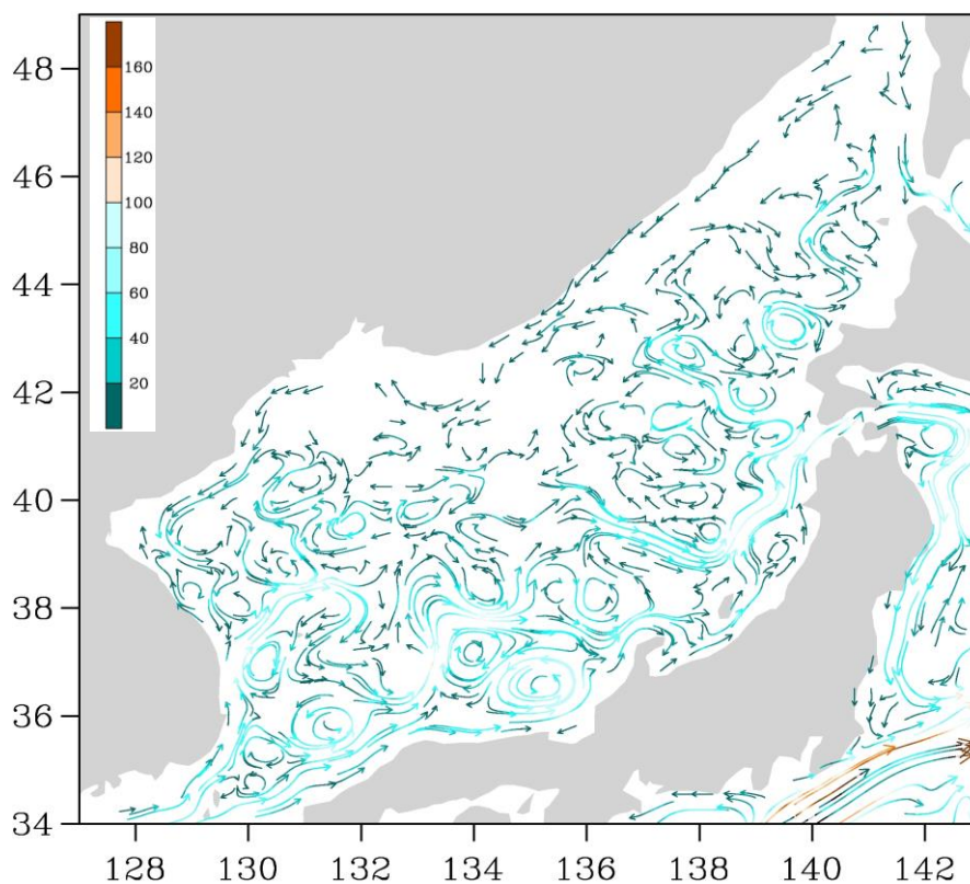
Рис. 3-3 Поверхностные течения Японского моря, 25 августа 2014 г.
