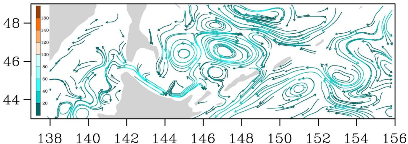
Рис. 3-7 Поверхностные течения, пролив Лаперуза, 5 августа 2014 г.
