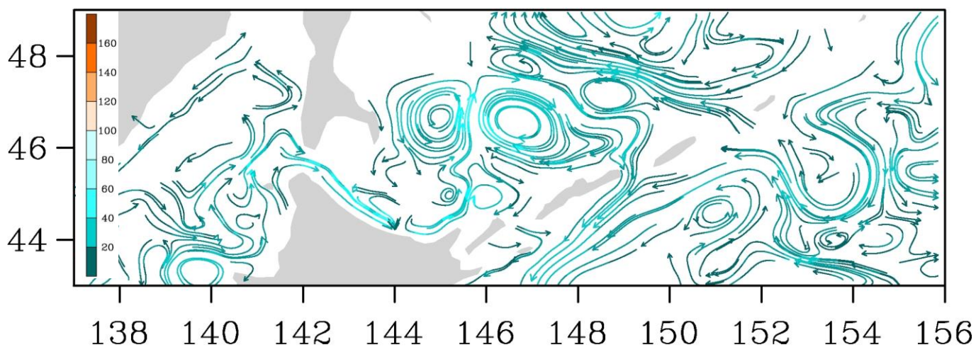
Рис. 3-8 Поверхностные течения, пролив Лаперуза, 15 августа 2014 г.
