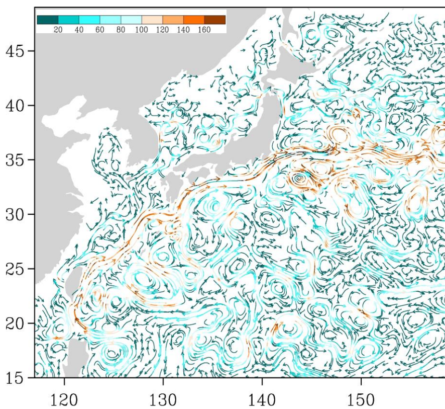
Рис. 3-4 Поверхностные течения западной части Тихого океана, 5 августа 2014 г.
