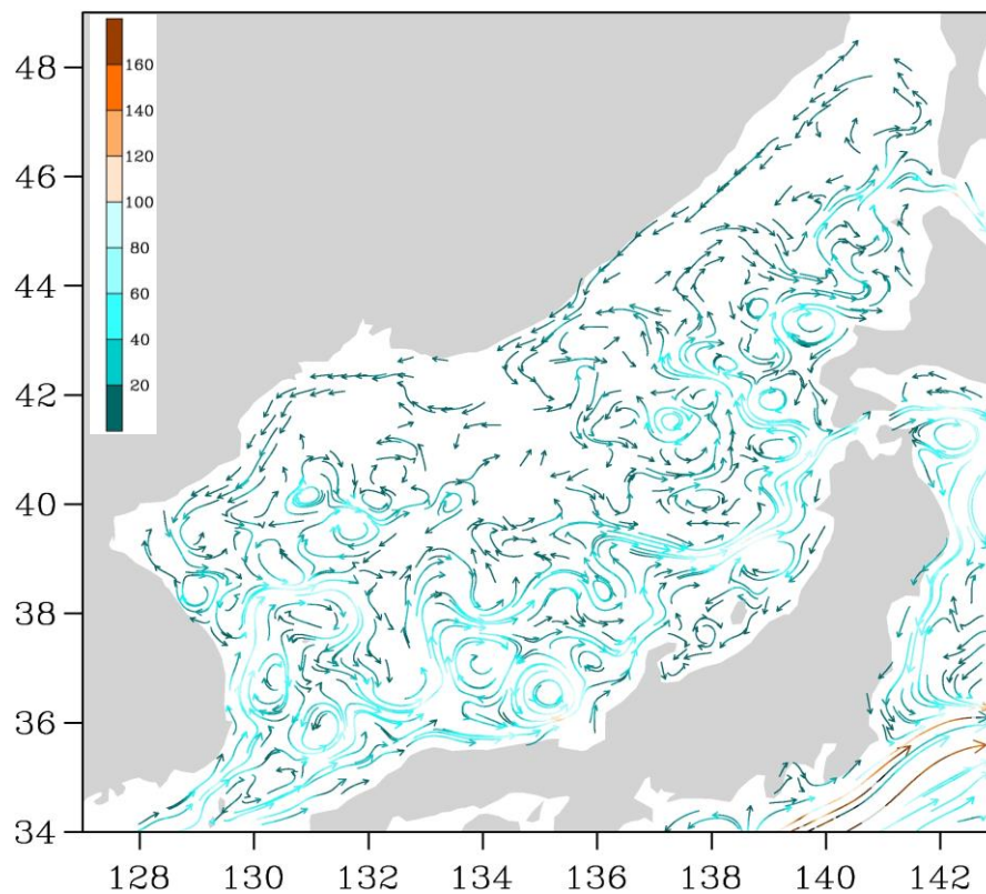
Рис. 3-2 Поверхностные течения Японского моря, 15 августа 2014 г.
