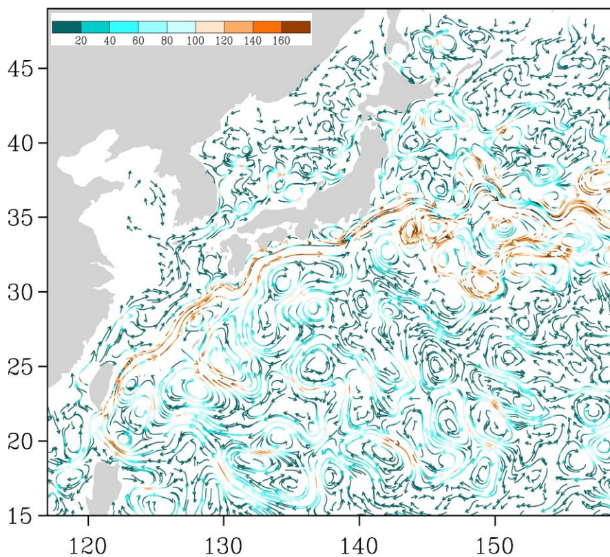
Рис. 3-6 Поверхностные течения западной части Тихого океана, 25 августа 2014 г.
