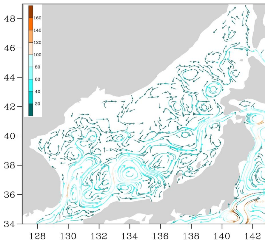
Рис. 3-1 Поверхностные течения Японского моря, 05 октября 2014 г.
