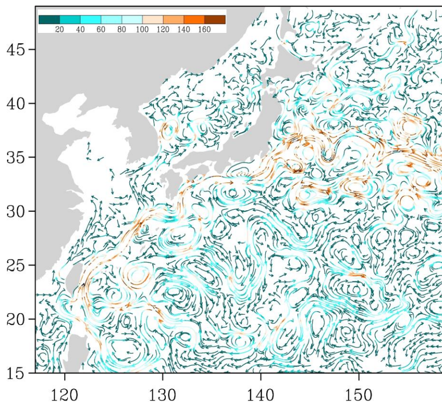
Рис. 3-6 Поверхностные течения западной части Тихого океана, 25 октября 2014 г.
