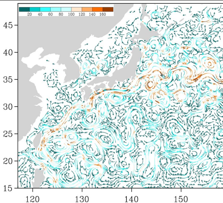
Рис. 3-5 Поверхностные течения западной части Тихого океана, 15 октября 2014 г.
