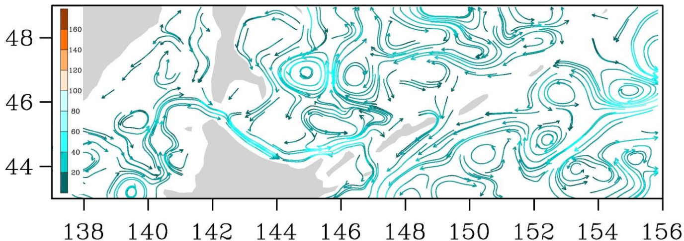
Рис. 3-7 Поверхностные течения, пролив Лаперуза, 5 октября 2014 г.
