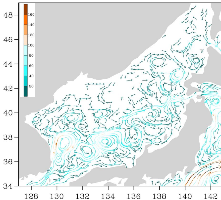
Рис. 3-2 Поверхностные течения Японского моря, 15 октября 2014 г.
