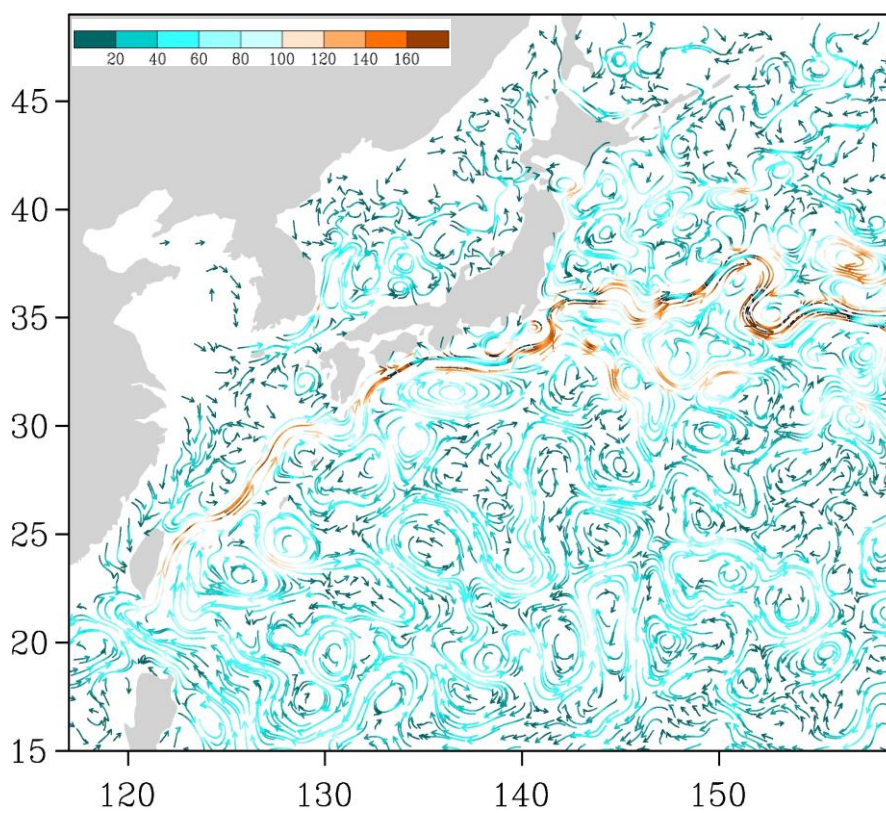
Рис. 3-4 Поверхностные течения западной части Тихого океана, 5 октября 2014 г.
