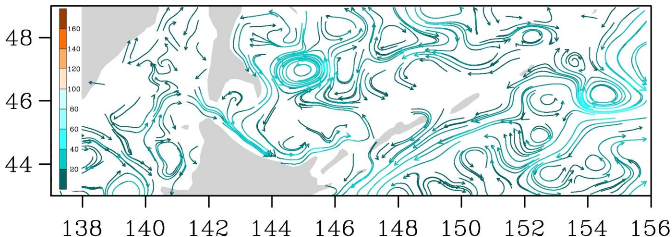
Рис. 3-8 Поверхностные течения, пролив Лаперуза, 15 октября 2014 г.
