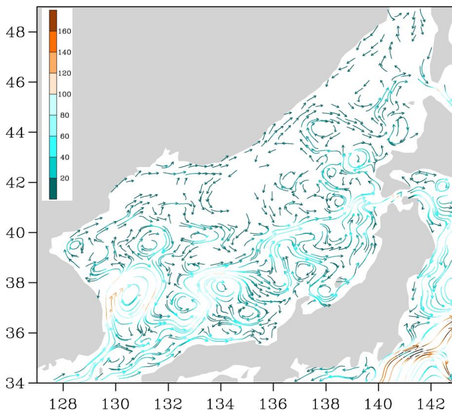
Рис. 3-3 Поверхностные течения Японского моря, 25 октября 2014 г.
