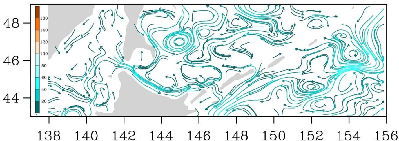
Рис. 3-9 Поверхностные течения, пролив Лаперуза, 25 октября 2014 г.
