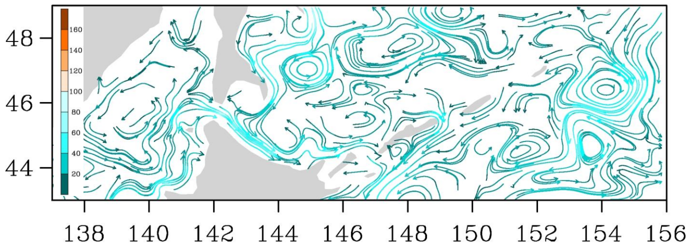
Рис. 3-7 Поверхностные течения, пролив Лаперуза, 5 ноября 2014 г.
