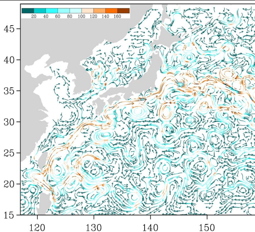
Рис. 3-5 Поверхностные течения западной части Тихого океана, 15 ноября 2014 г.
