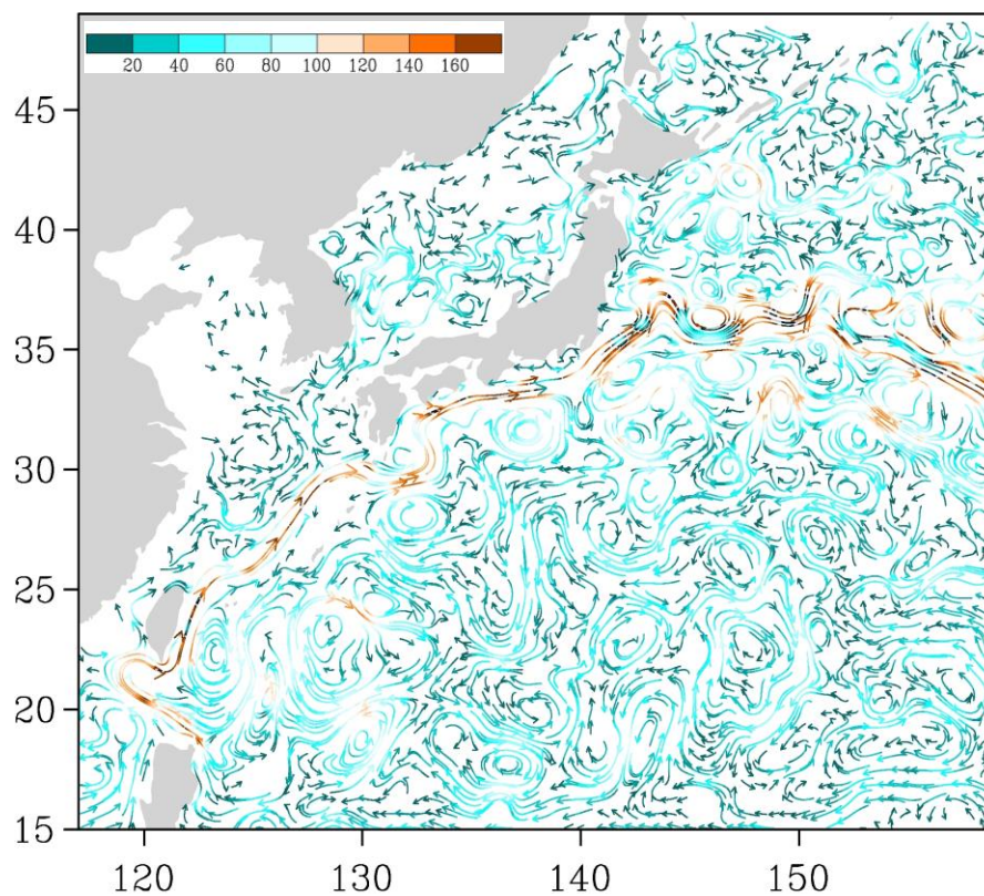
Рис. 3-6 Поверхностные течения западной части Тихого океана, 25 ноября 2014 г.
