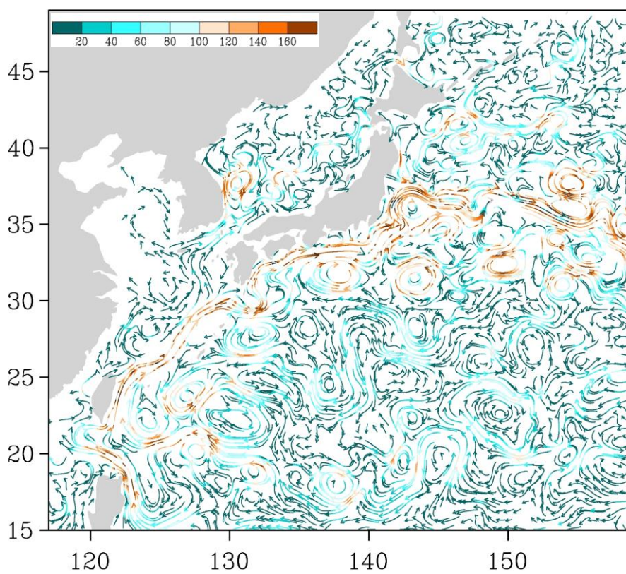
Рис. 3-4 Поверхностные течения западной части Тихого океана, 5 ноября 2014 г.
