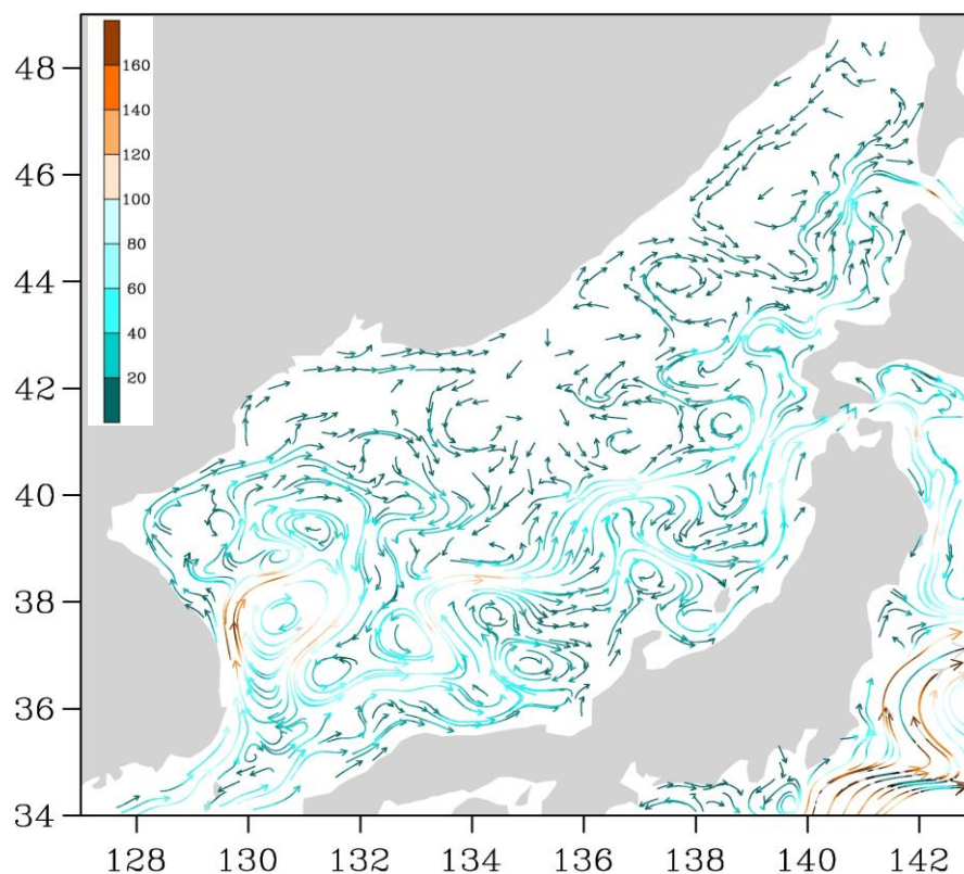
Рис. 3-1 Поверхностные течения Японского моря, 05 ноября 2014 г.
