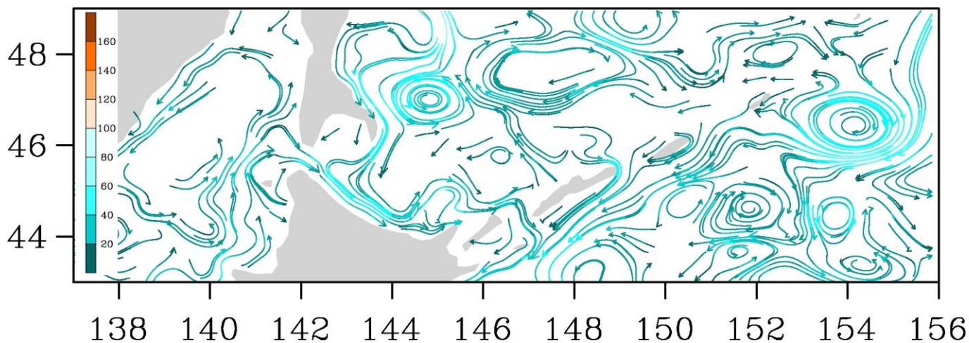
Рис. 3-8 Поверхностные течения, пролив Лаперуза, 15 ноября 2014 г.
