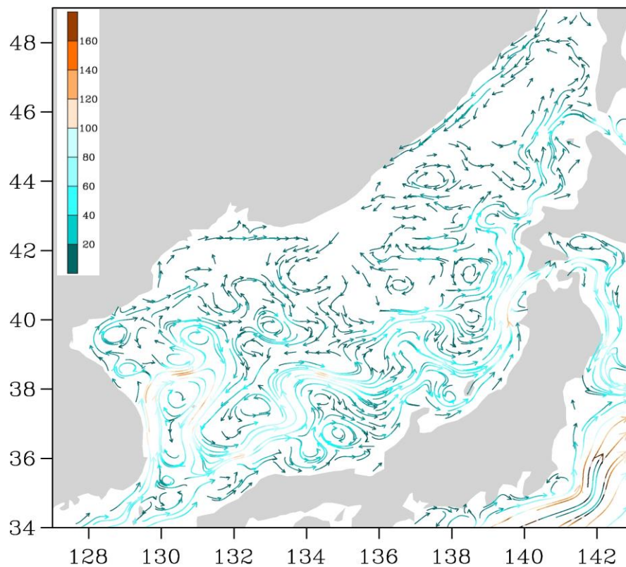
Рис. 3-2 Поверхностные течения Японского моря, 15 ноября 2014 г.
