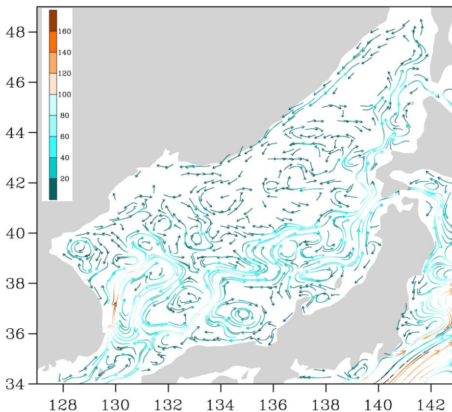
Рис. 3-3 Поверхностные течения Японского моря, 25 ноября 2014 г.
