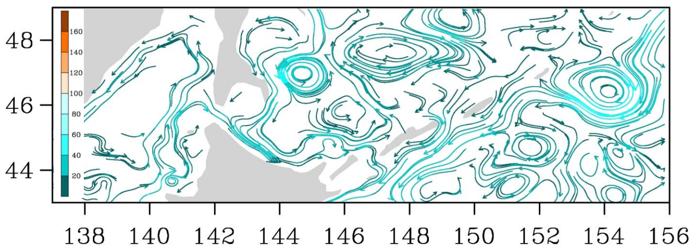
Рис. 3-9 Поверхностные течения, пролив Лаперуза, 25 ноября 2014 г.
