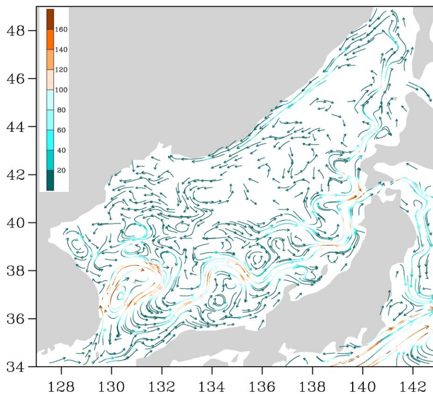
Рис. 3-2 Поверхностные течения Японского моря, 15 декабря 2014 г.
