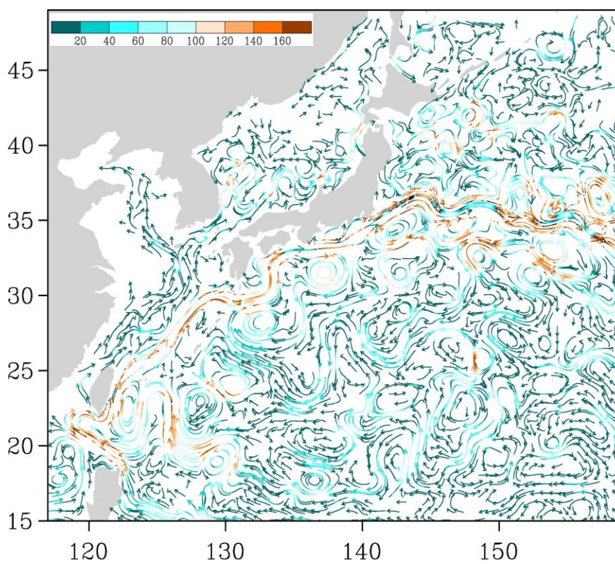
Рис. 3-4 Поверхностные течения западной части Тихого океана, 5 декабря 2014 г.
