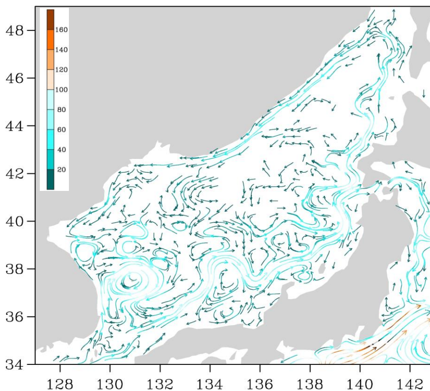
Рис. 3-3 Поверхностные течения Японского моря, 25 декабря 2014 г.
