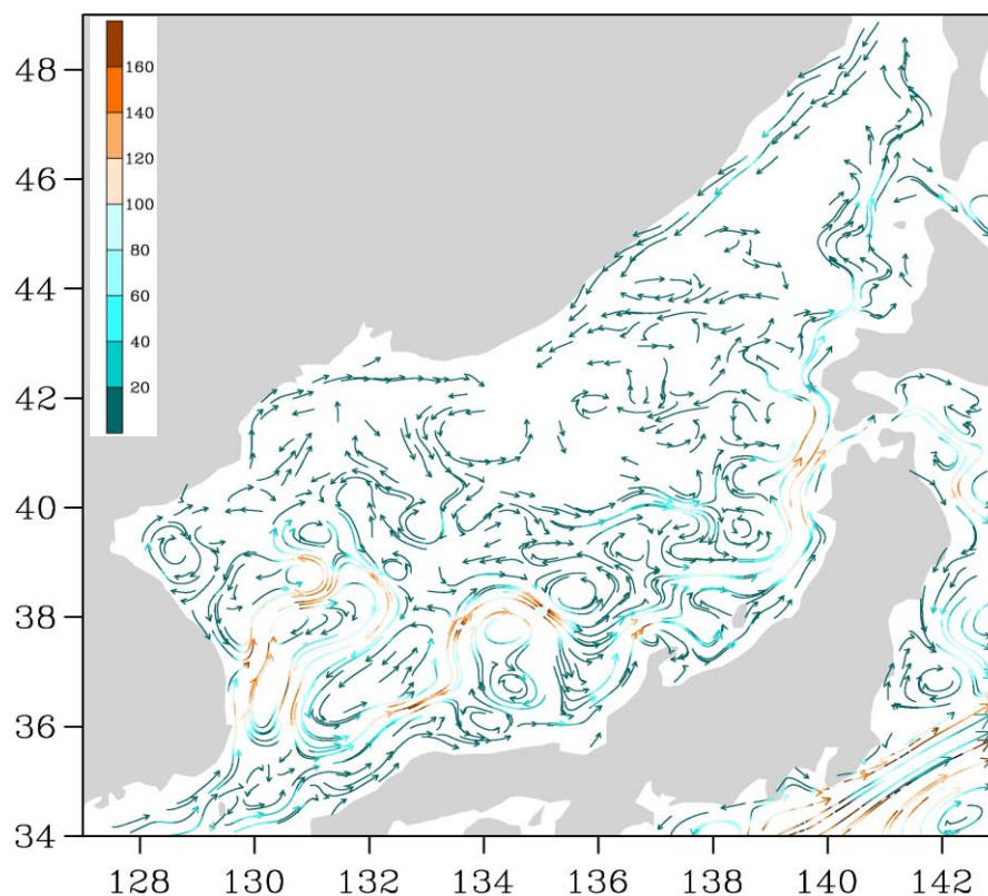
Рис. 3-1 Поверхностные течения Японского моря, 05 декабря 2014 г.
