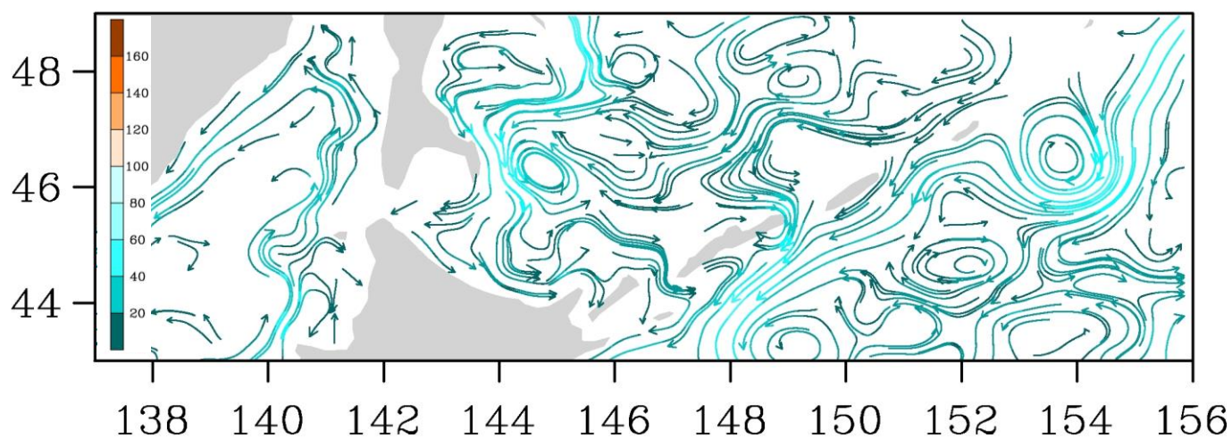
Рис. 3-9 Поверхностные течения, пролив Лаперуза, 25 декабря 2014 г.
