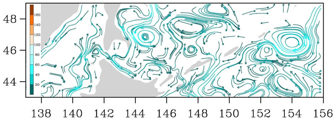
Рис. 3-7 Поверхностные течения, пролив Лаперуза, 5 декабря 2014 г.
