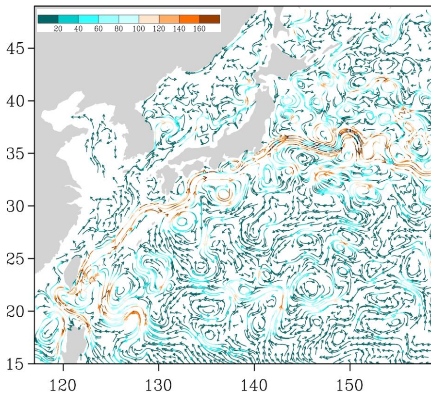
Рис. 3-6 Поверхностные течения западной части Тихого океана, 25 декабря 2014 г.
