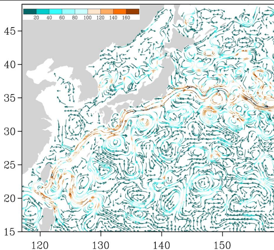
Рис. 3-5 Поверхностные течения западной части Тихого океана, 15 декабря 2014 г.
