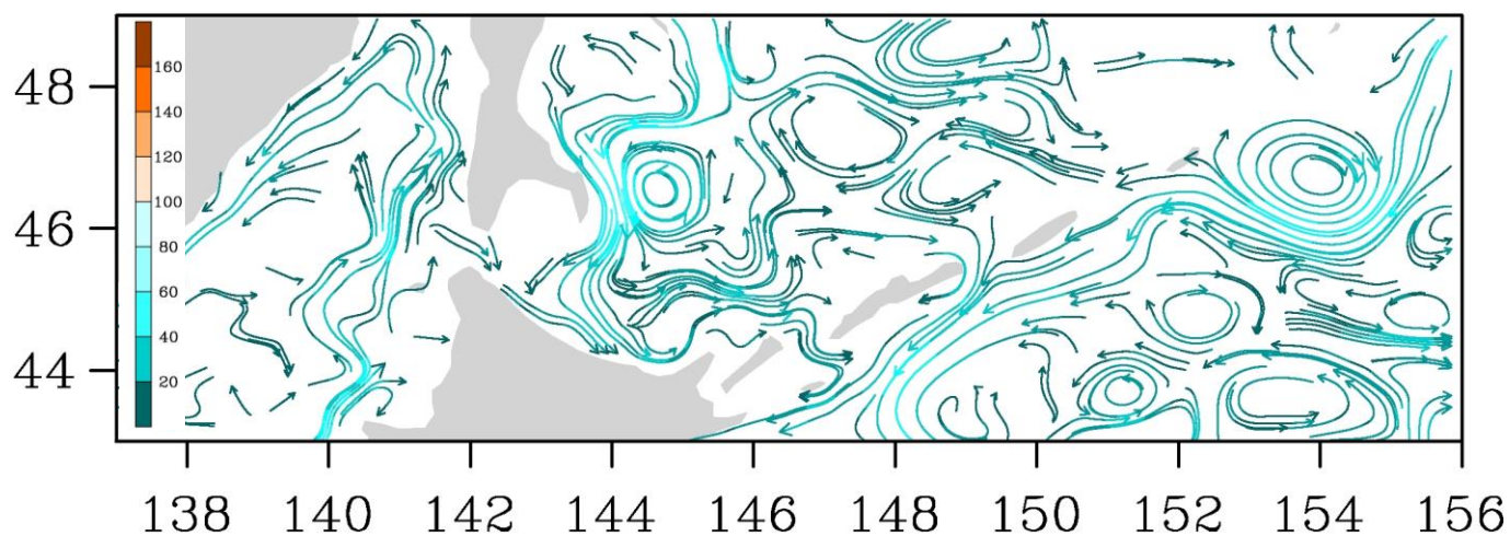
Рис. 3-8 Поверхностные течения, пролив Лаперуза, 15 декабря 2014 г.
