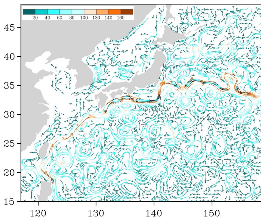
Рис. 3-6 Поверхностные течения западной части Тихого океана, 25 марта 2015 г.
