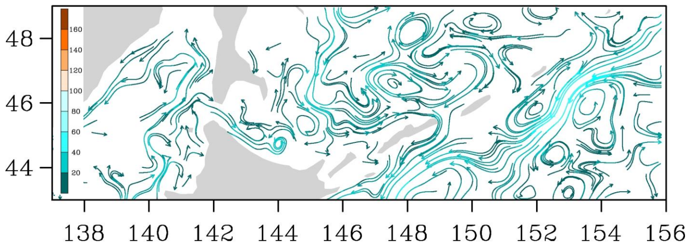
Рис. 3-8 Поверхностные течения, пролив Лаперуза, 15 марта 2015 г.
