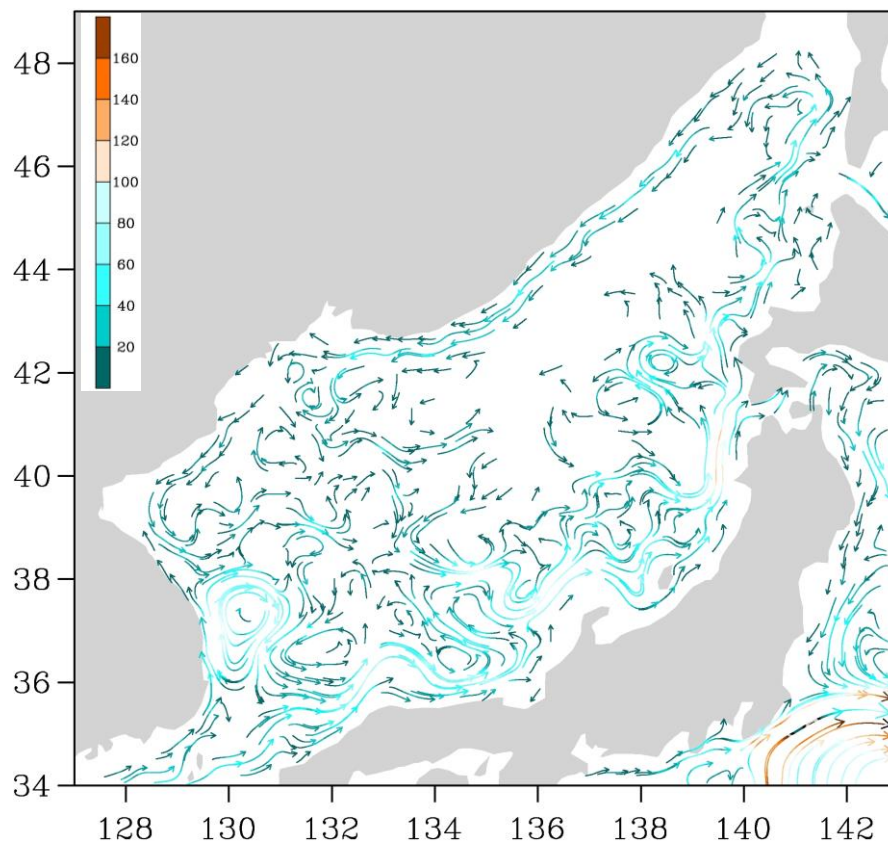
Рис. 3-2 Поверхностные течения Японского моря, 15 марта 2015 г.
