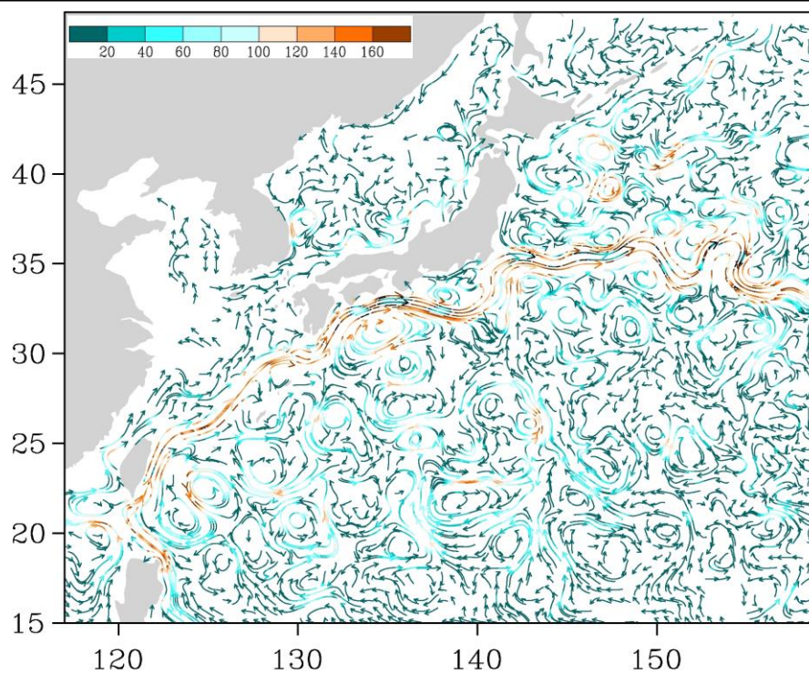
Рис. 3-5 Поверхностные течения западной части Тихого океана, 15 марта 2015 г.
