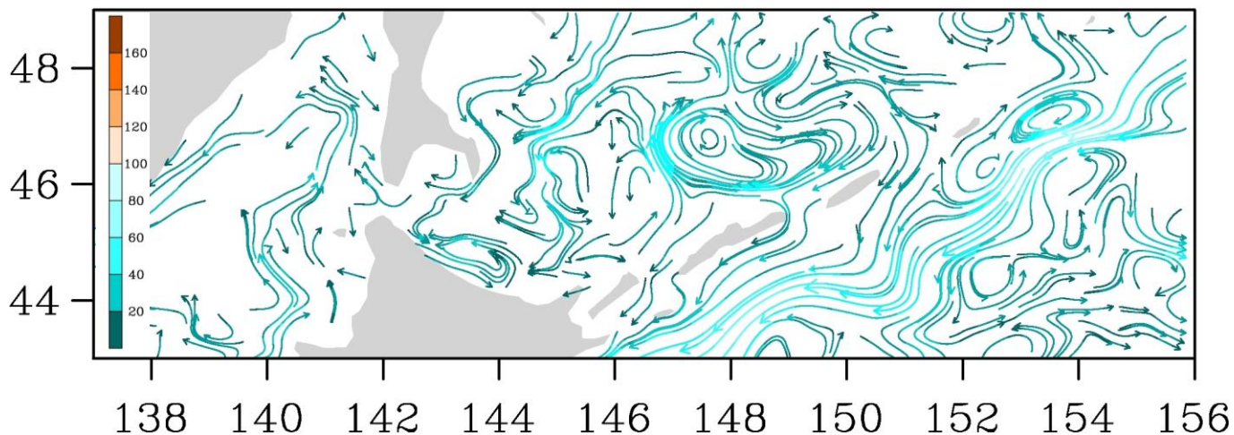
Рис. 3-7 Поверхностные течения, пролив Лаперуза, 5 марта 2015 г.
