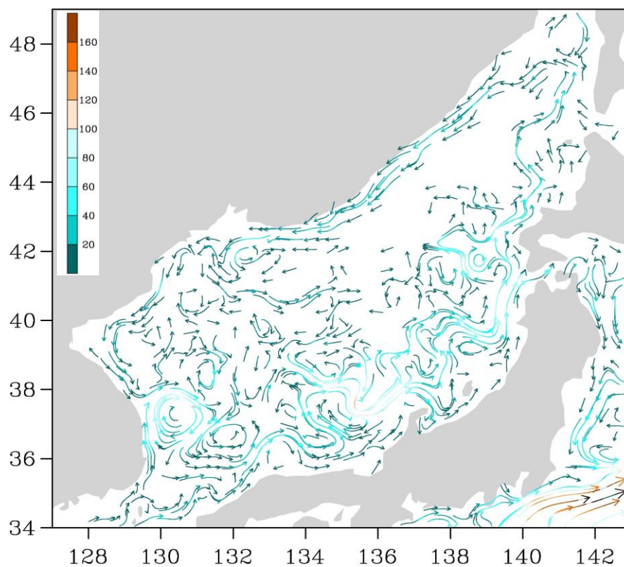
Рис. 3-1 Поверхностные течения Японского моря, 05 марта 2015 г.
