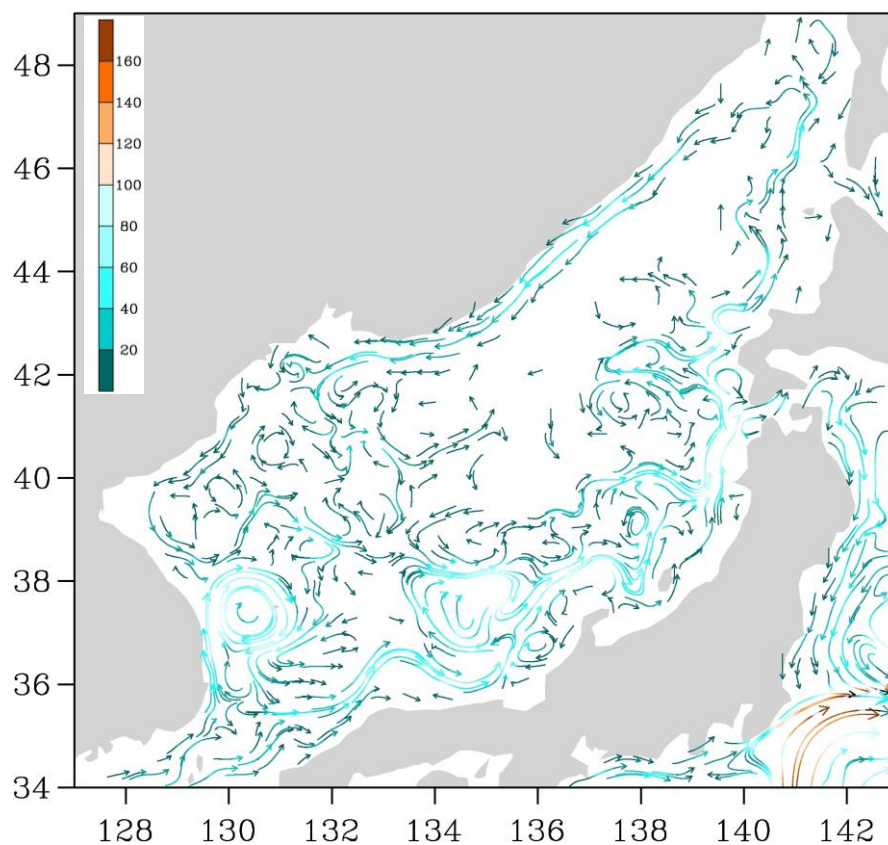
Рис. 3-3 Поверхностные течения Японского моря, 25 марта 2015 г.
