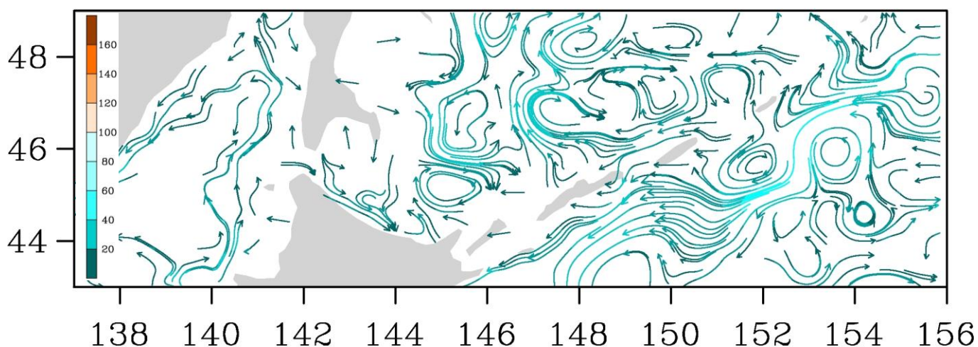
Рис. 3-9 Поверхностные течения, пролив Лаперуза, 25 марта 2015 г.
