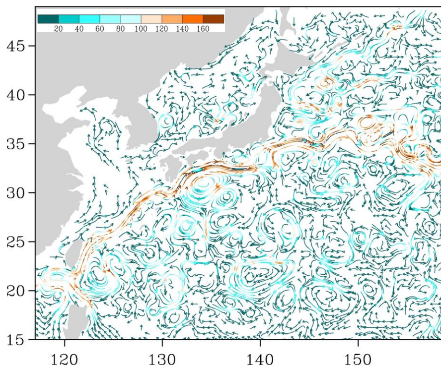
Рис. 3-4 Поверхностные течения западной части Тихого океана, 5 марта 2015 г.
