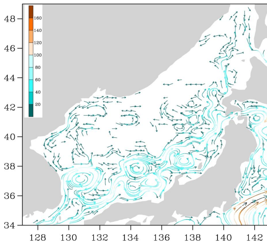
Рис. 3-1 Поверхностные течения Японского моря, 05 сентября 2015 г.
