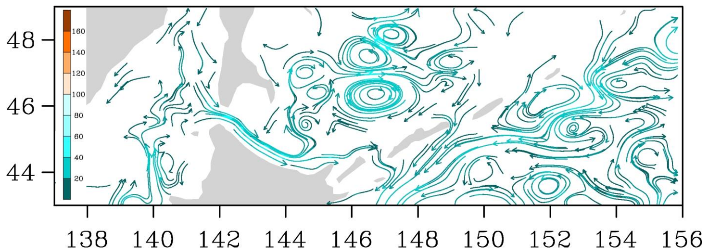
Рис. 3-7 Поверхностные течения, пролив Лаперуза, 5 сентября 2015 г.
