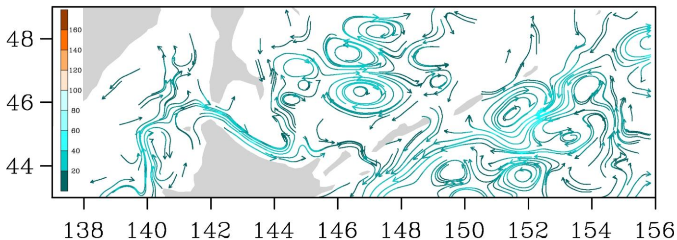
Рис. 3-8 Поверхностные течения, пролив Лаперуза, 15 сентября 2015 г.
