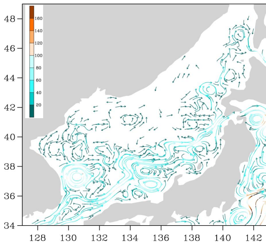
Рис. 3-3 Поверхностные течения Японского моря, 25 сентября 2015 г.
