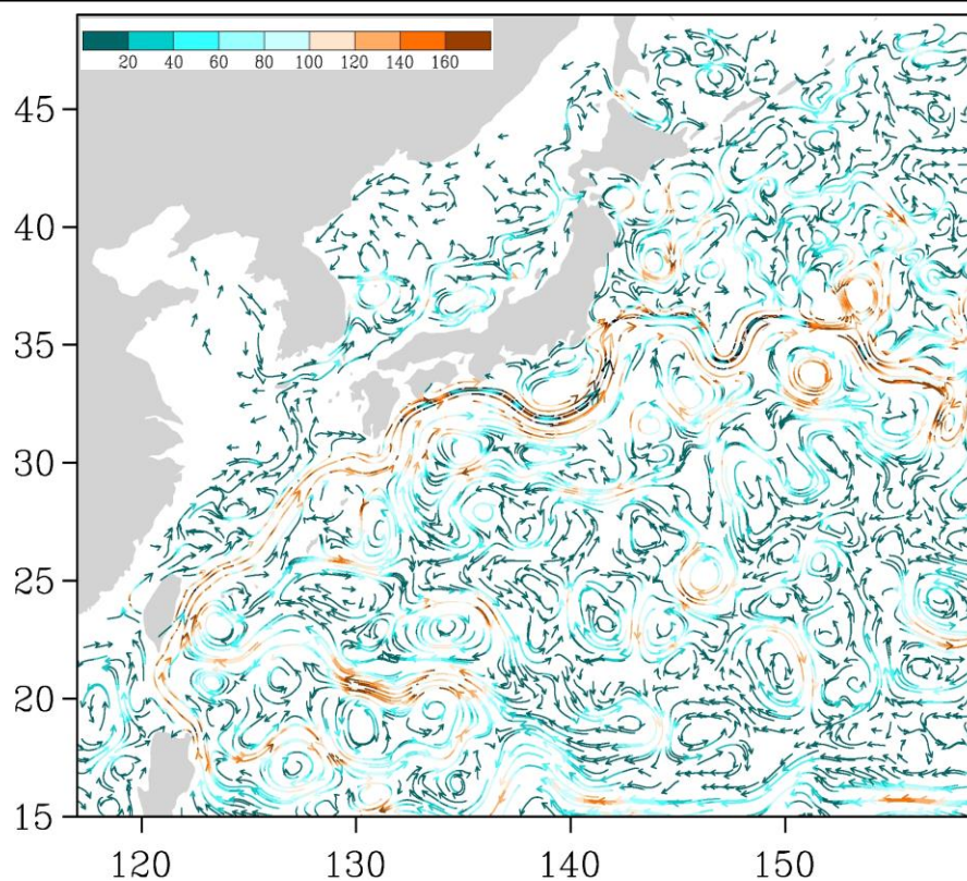
Рис. 3-5 Поверхностные течения западной части Тихого океана, 15 сентября 2015 г.
