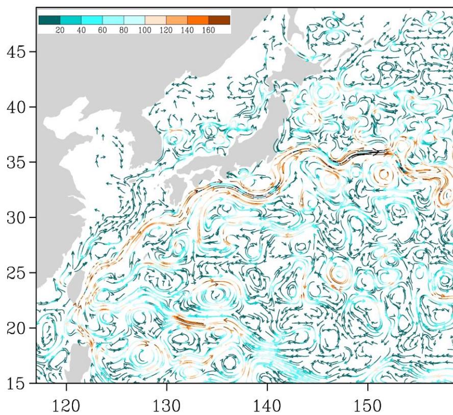
Рис. 3-4 Поверхностные течения западной части Тихого океана, 5 сентября 2015 г.
