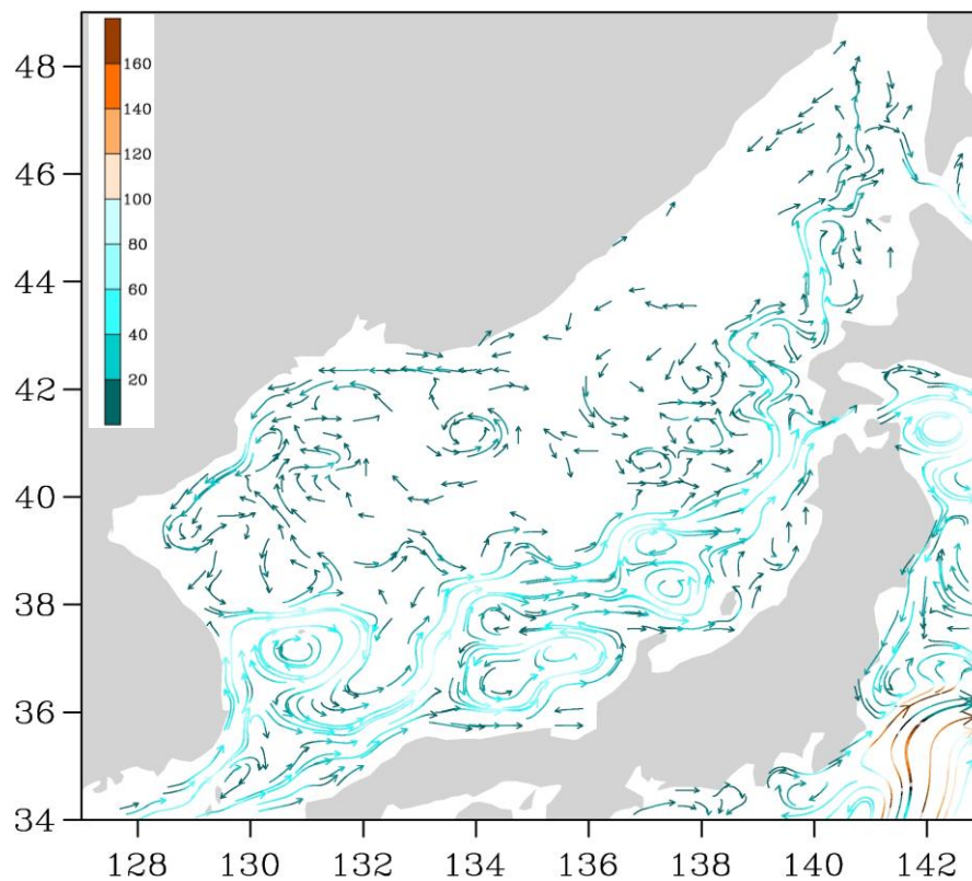
Рис. 3-2 Поверхностные течения Японского моря, 15 сентября 2015 г.
