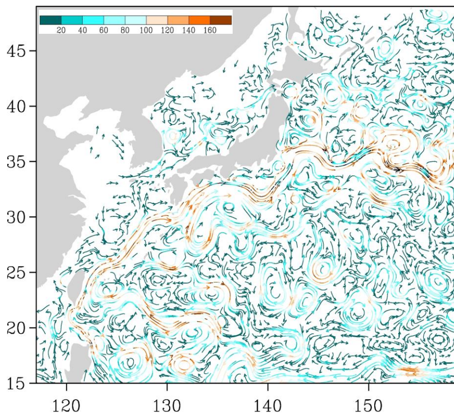
Рис. 3-6 Поверхностные течения западной части Тихого океана, 25 сентября 2015 г.
