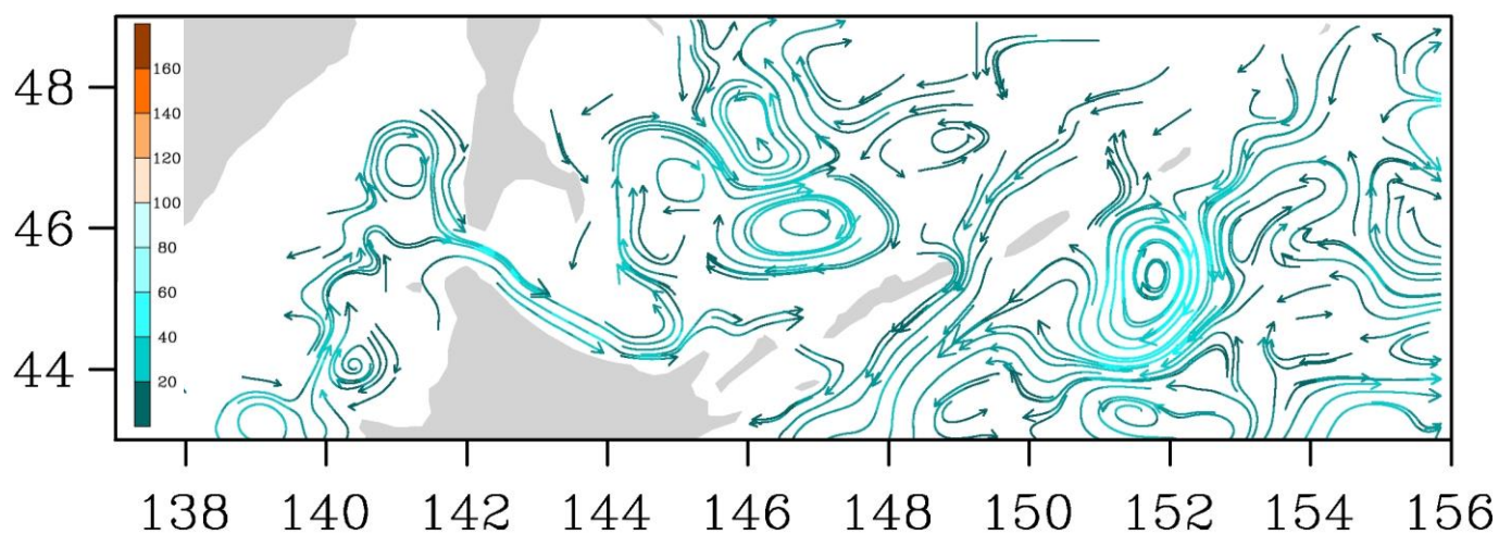
Рис. 3-9 Поверхностные течения, пролив Лаперуза, 25 сентября 2015 г.
