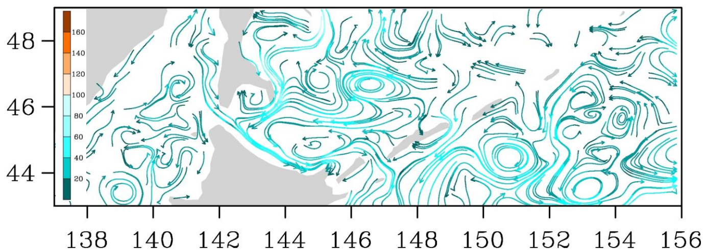
Рис. 3-9 Поверхностные течения, пролив Лаперуза, 25 октября 2015 г.
