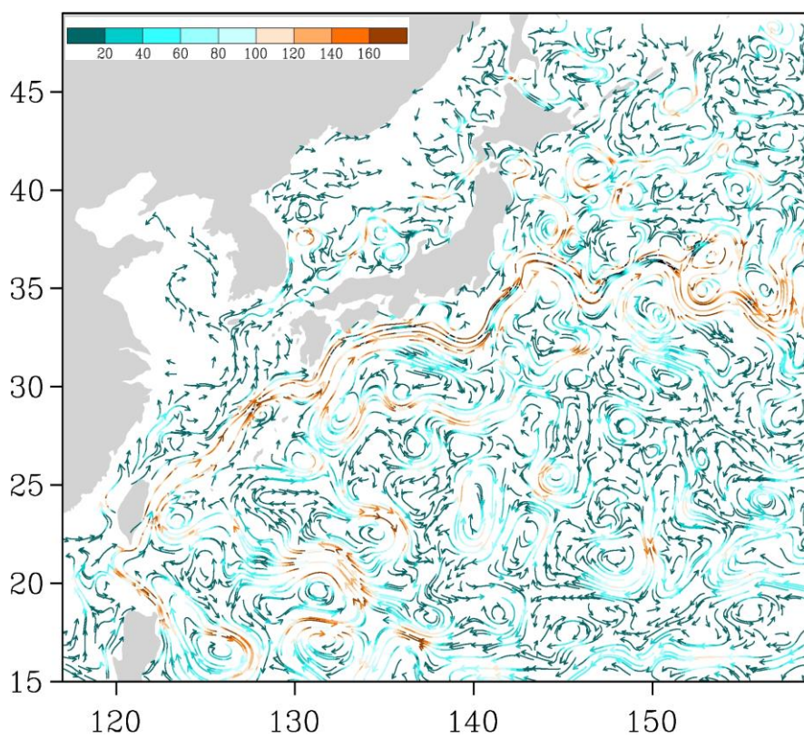
Рис. 3-4 Поверхностные течения западной части Тихого океана, 5 октября 2015 г.
