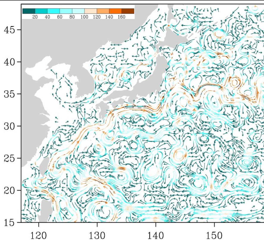
Рис. 3-5 Поверхностные течения западной части Тихого океана, 15 октября 2015 г.
