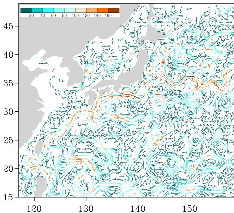
Рис. 3-6 Поверхностные течения западной части Тихого океана, 25 октября 2015 г.
