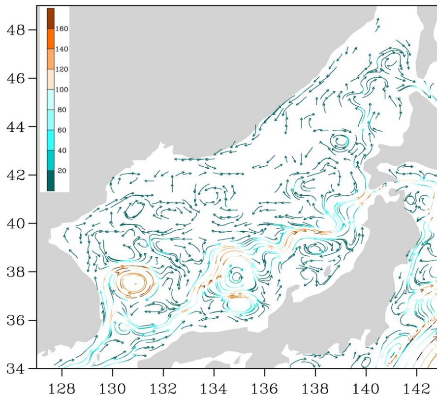
Рис. 3-2 Поверхностные течения Японского моря, 15 октября 2015 г.
