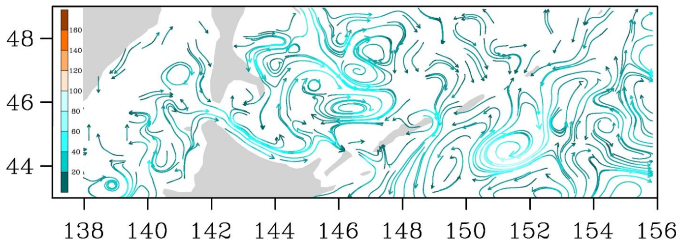
Рис. 3-7 Поверхностные течения, пролив Лаперуза, 5 октября 2015 г.
