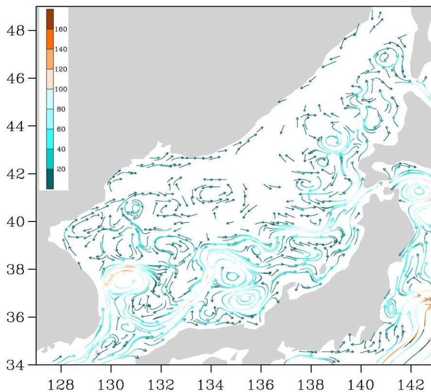
Рис. 3-1 Поверхностные течения Японского моря, 05 октября 2015 г.
