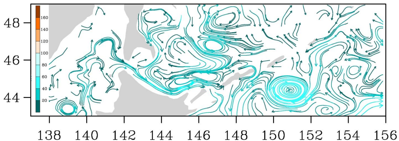
Рис. 3-8 Поверхностные течения, пролив Лаперуза, 15 октября 2015 г.
