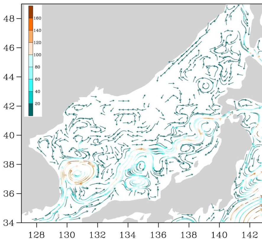
Рис. 3-3 Поверхностные течения Японского моря, 25 октября 2015 г.
