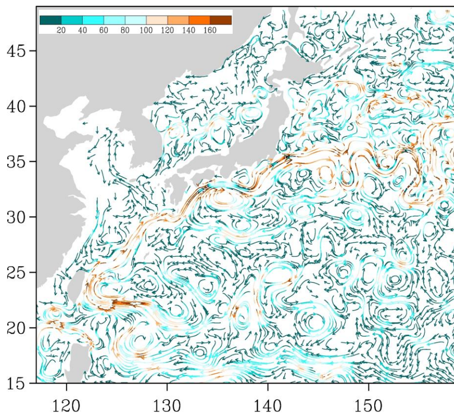
Рис. 3-6 Поверхностные течения западной части Тихого океана, 25 ноября 2015 г.
