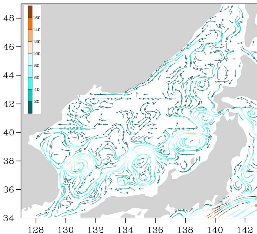
Рис. 3-3 Поверхностные течения Японского моря, 25 ноября 2015 г.
