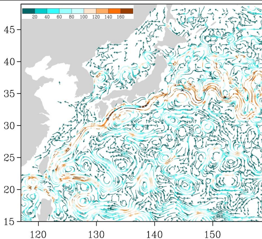
Рис. 3-5 Поверхностные течения западной части Тихого океана, 15 ноября 2015 г.
