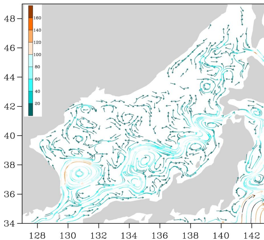
Рис. 3-1 Поверхностные течения Японского моря, 05 ноября 2015 г.
