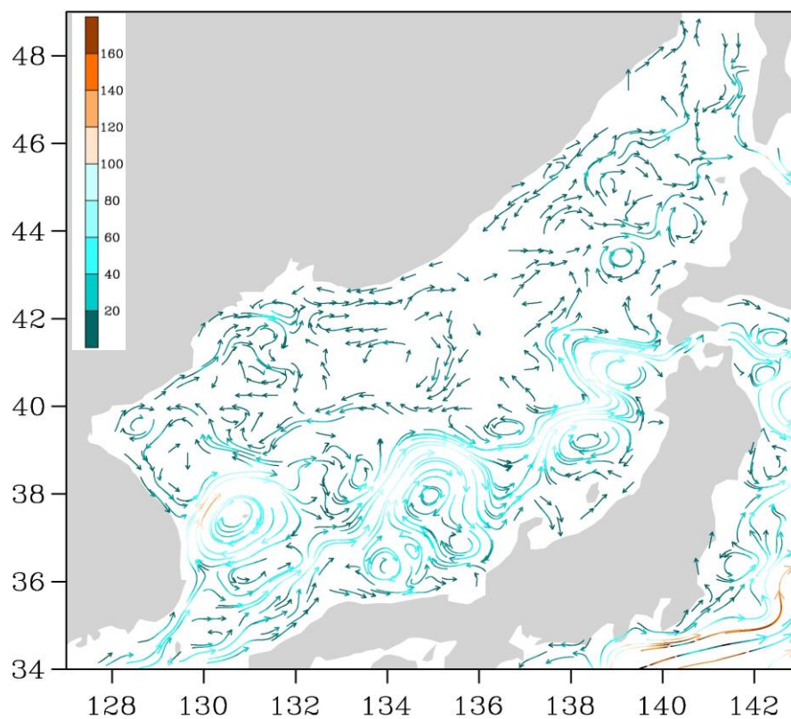
Рис. 3-2 Поверхностные течения Японского моря, 15 ноября 2015 г.
