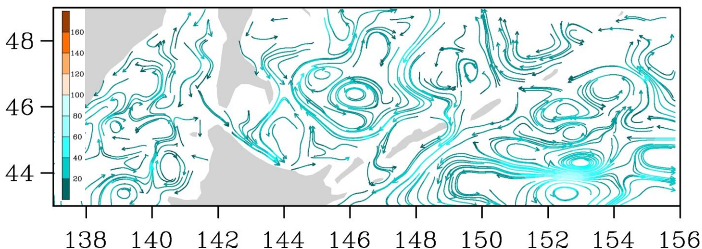
Рис. 3-9 Поверхностные течения, пролив Лаперуза, 25 ноября 2015 г.
