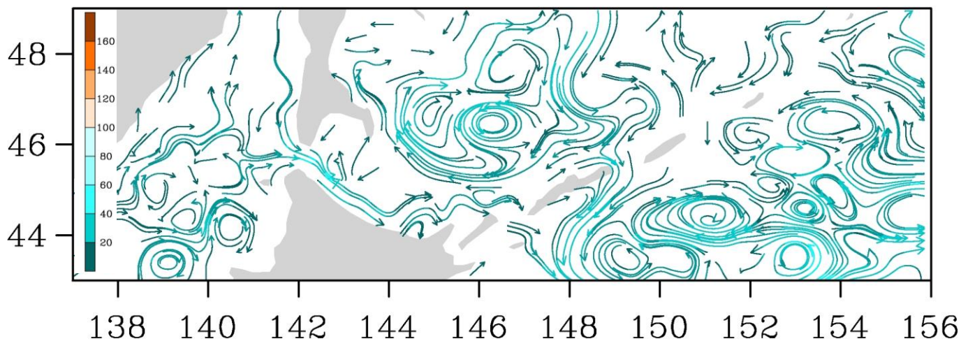
Рис. 3-8 Поверхностные течения, пролив Лаперуза, 15 ноября 2015 г.
