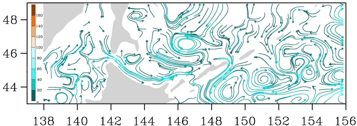
Рис. 3-7 Поверхностные течения, пролив Лаперуза, 5 ноября 2015 г.
