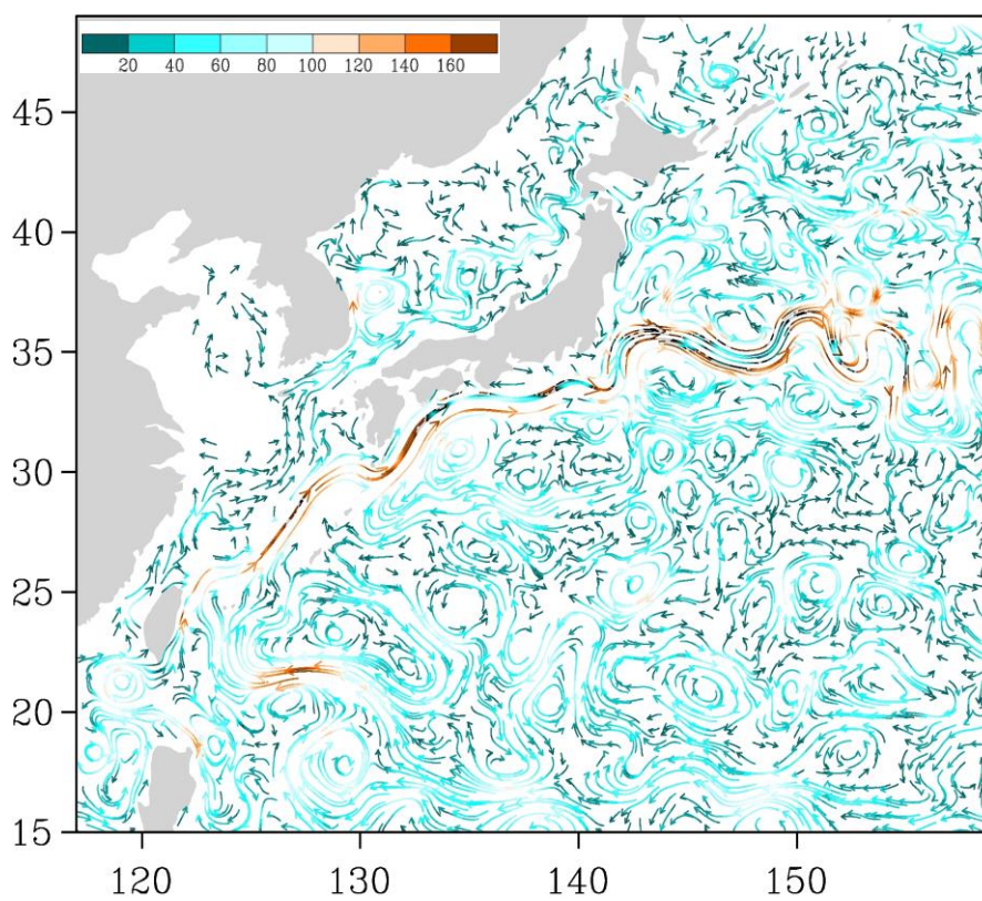
Рис. 3-4 Поверхностные течения западной части Тихого океана, 5 ноября 2015 г.
