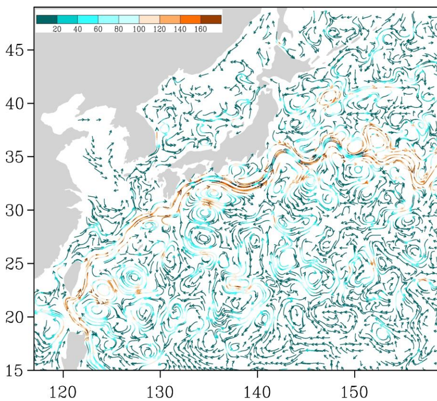
Рис. 3-4 Поверхностные течения западной части Тихого океана, 5 апреля 2015 г.
