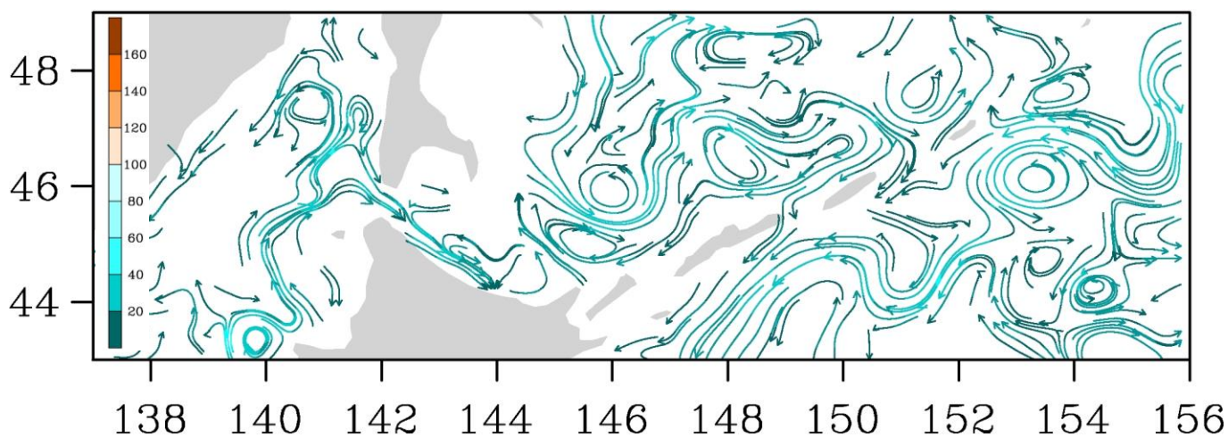
Рис. 3-8 Поверхностные течения, пролив Лаперуза, 15 апреля 2015 г.
