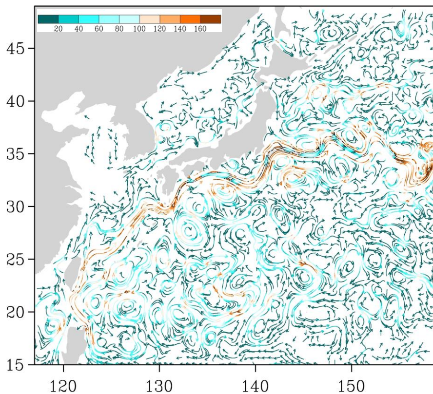
Рис. 3-6 Поверхностные течения западной части Тихого океана, 25 апреля 2015 г.
