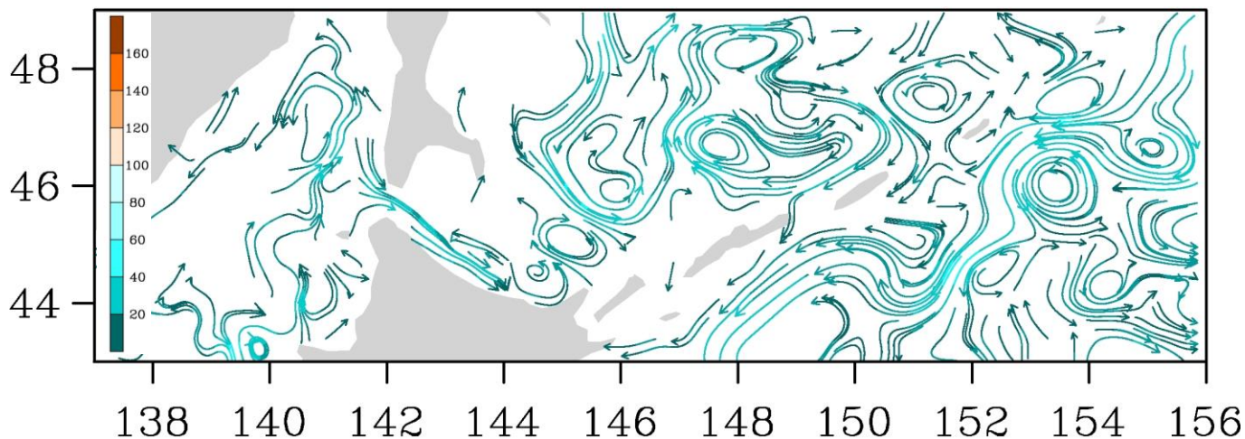
Рис. 3-7 Поверхностные течения, пролив Лаперуза, 5 апреля 2015 г.
