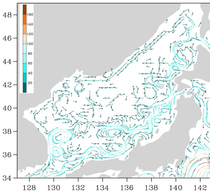
Рис. 3-3 Поверхностные течения Японского моря, 25 апреля 2015 г.
