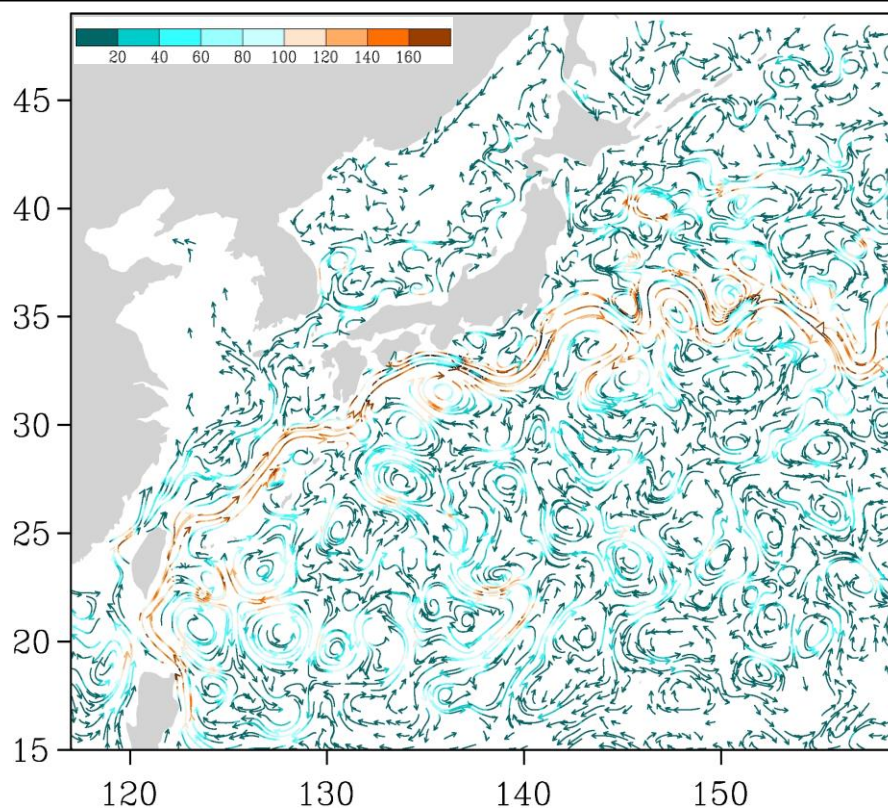
Рис. 3-5 Поверхностные течения западной части Тихого океана, 15 апреля 2015 г.
