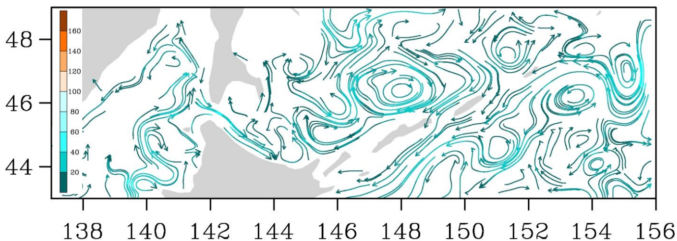
Рис. 3-9 Поверхностные течения, пролив Лаперуза, 25 апреля 2015 г.
