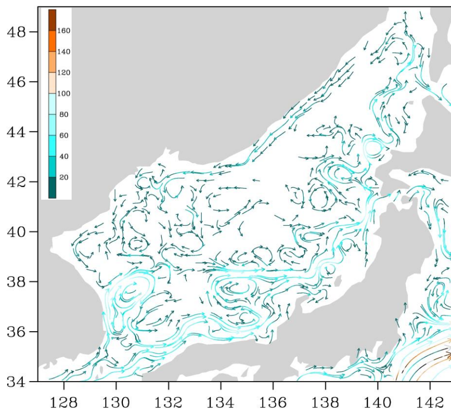
Рис. 3-2 Поверхностные течения Японского моря, 15 апреля 2015 г.
