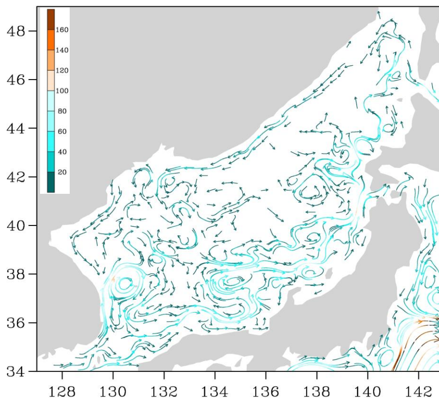
Рис. 3-1 Поверхностные течения Японского моря, 05 апреля 2015 г.
