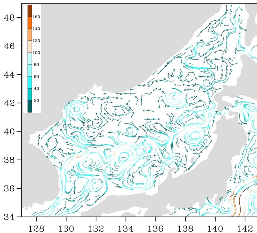
Рис. 3-2 Поверхностные течения Японского моря, 15 ноября 2016 г.
