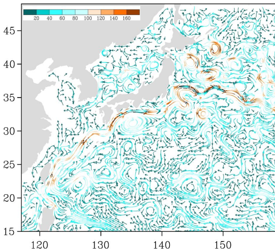
Рис. 3-6 Поверхностные течения западной части Тихого океана, 25 ноября 2016 г.
