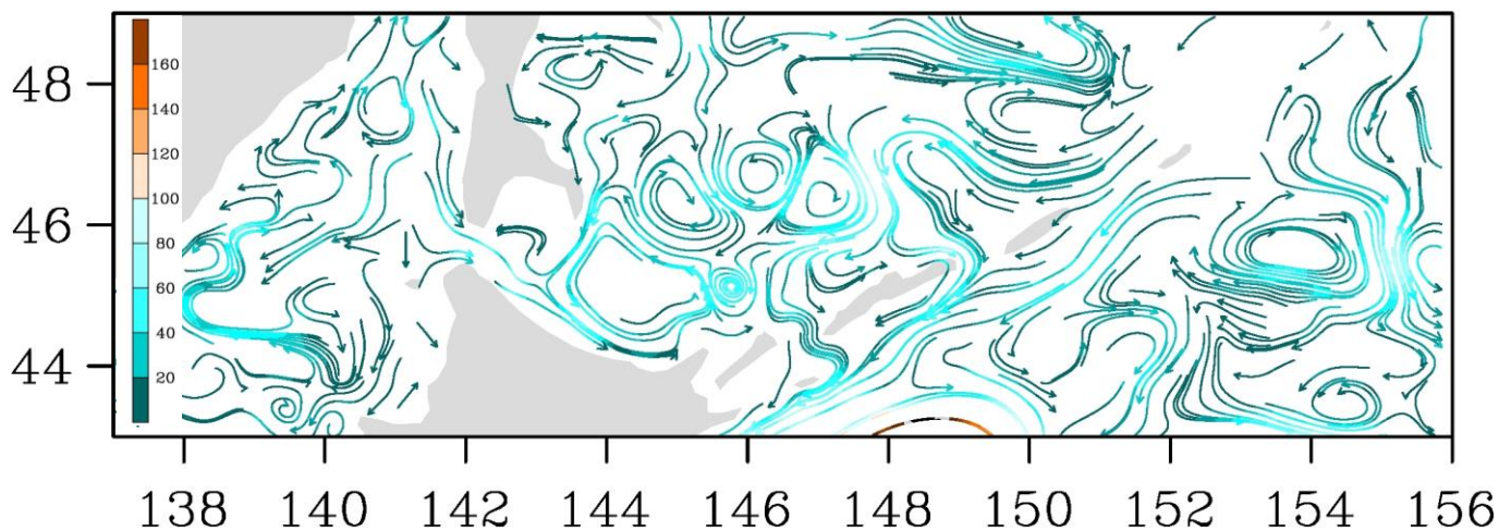
Рис. 3-8 Поверхностные течения, пролив Лаперуза, 15 ноября 2016 г.
