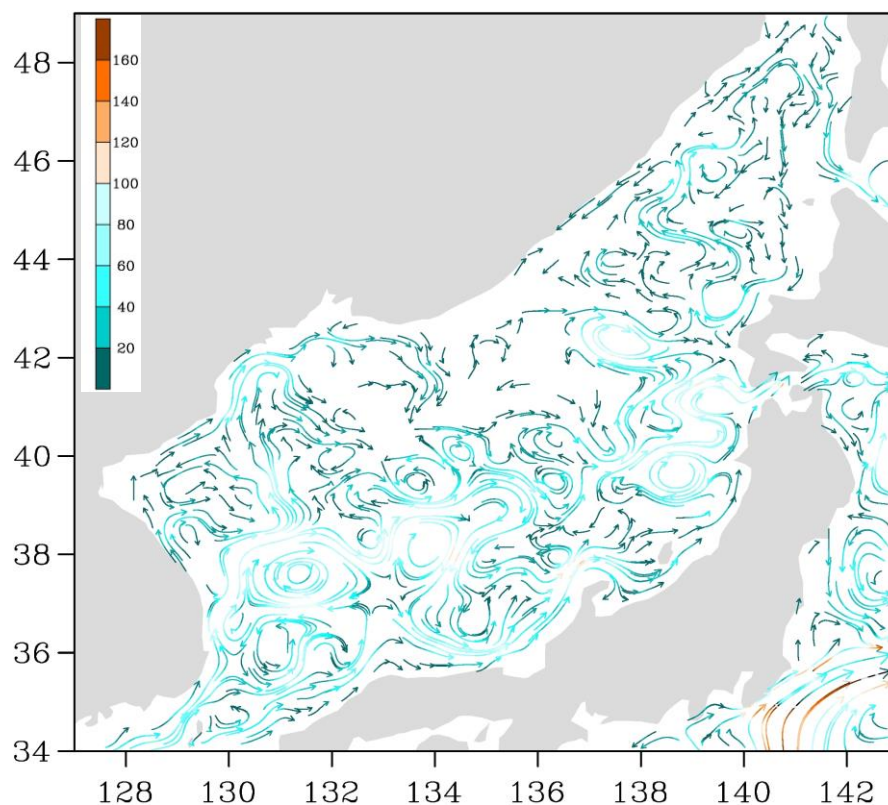
Рис. 3-1 Поверхностные течения Японского моря, 05 ноября 2016 г.
