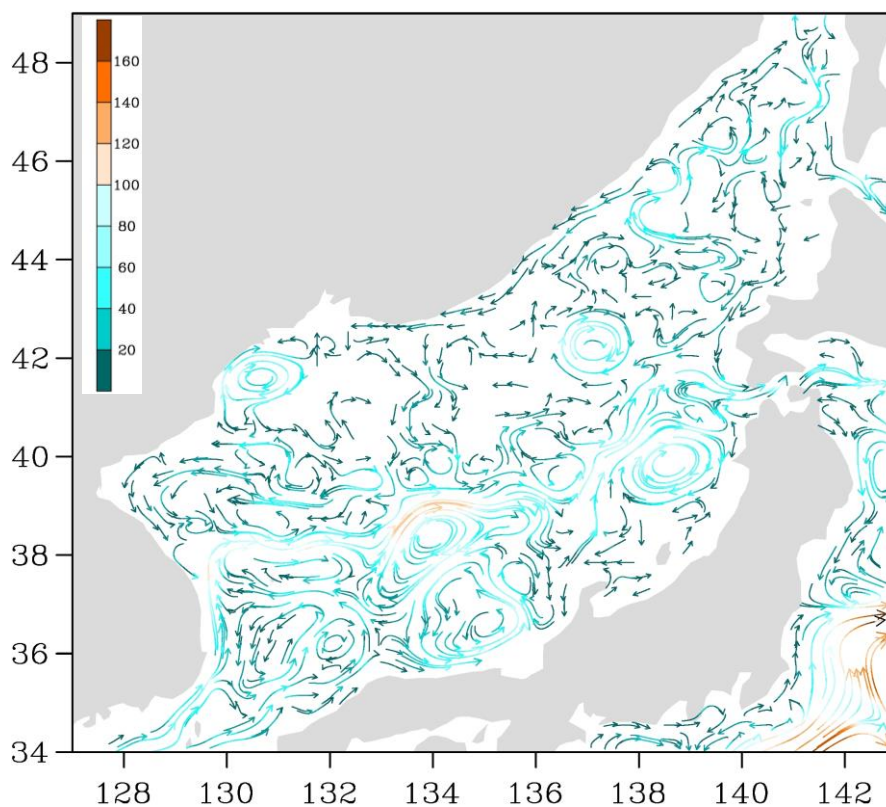
Рис. 3-3 Поверхностные течения Японского моря, 25 ноября 2016 г.
