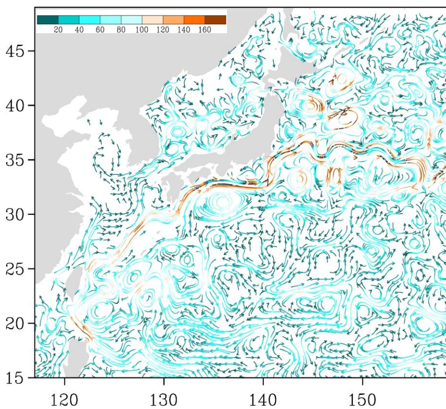
Рис. 3-4 Поверхностные течения западной части Тихого океана, 5 ноября 2016 г.
