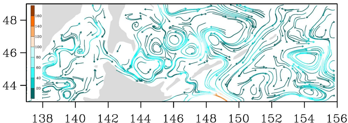
Рис. 3-9 Поверхностные течения, пролив Лаперуза, 25 ноября 2016 г.
