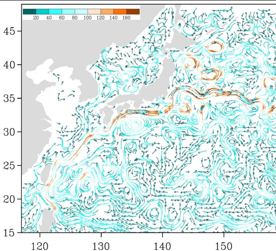
Рис. 3-5 Поверхностные течения западной части Тихого океана, 15 ноября 2016 г.
