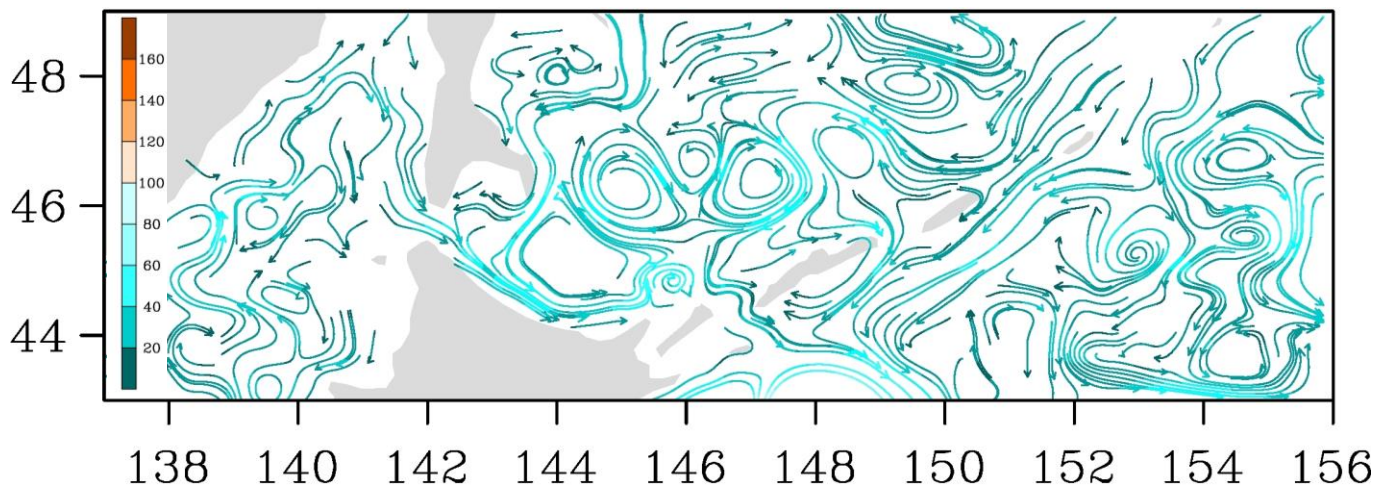
Рис. 3-7 Поверхностные течения, пролив Лаперуза, 5 ноября 2016 г.
