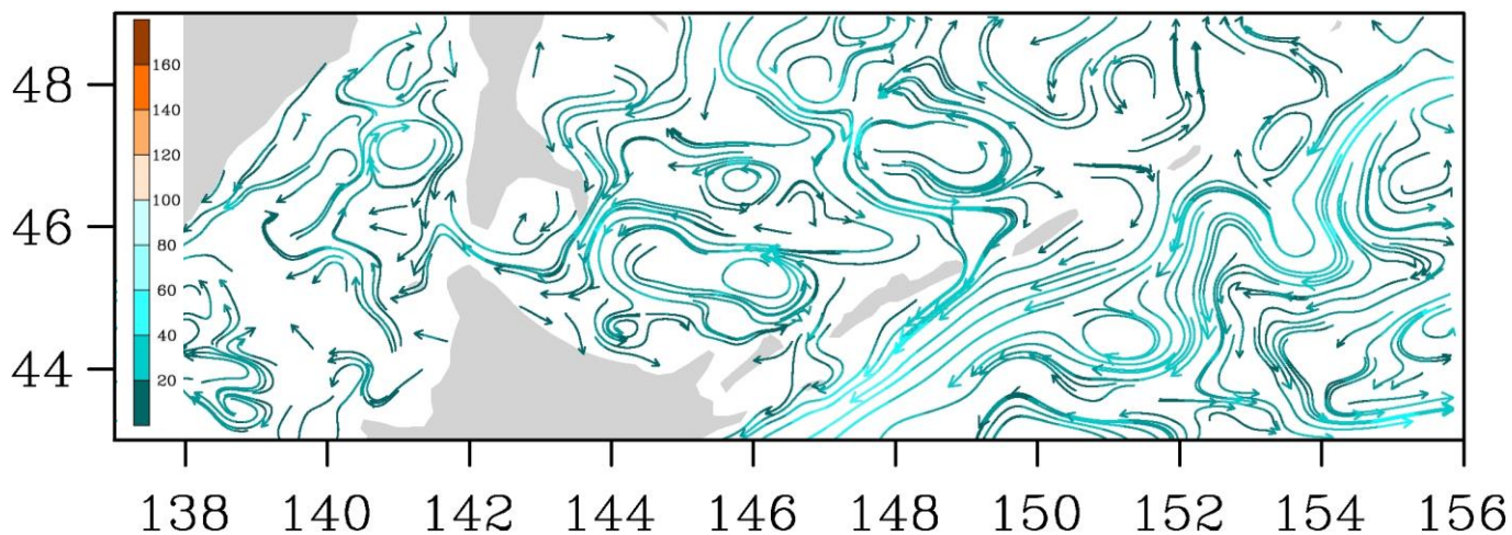
Рис. 3-8 Поверхностные течения, пролив Лаперуза, 15 февраля 2016 г.
