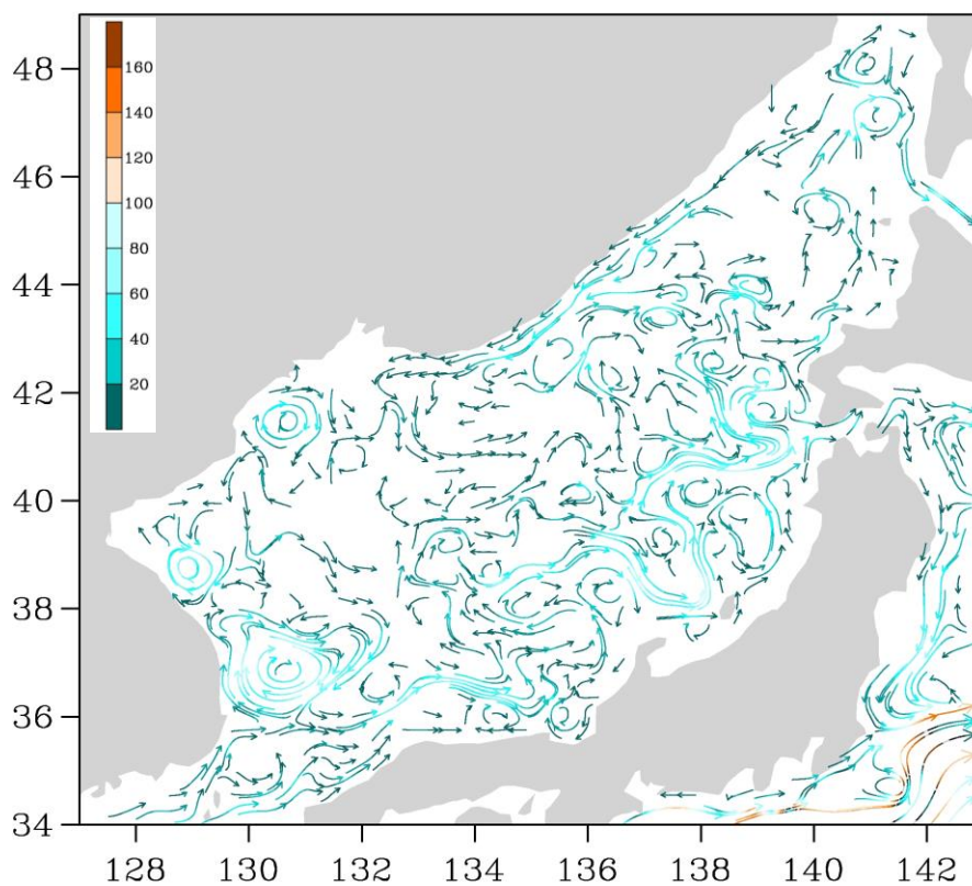
Рис. 3-3 Поверхностные течения Японского моря, 25 февраля 2016 г.
