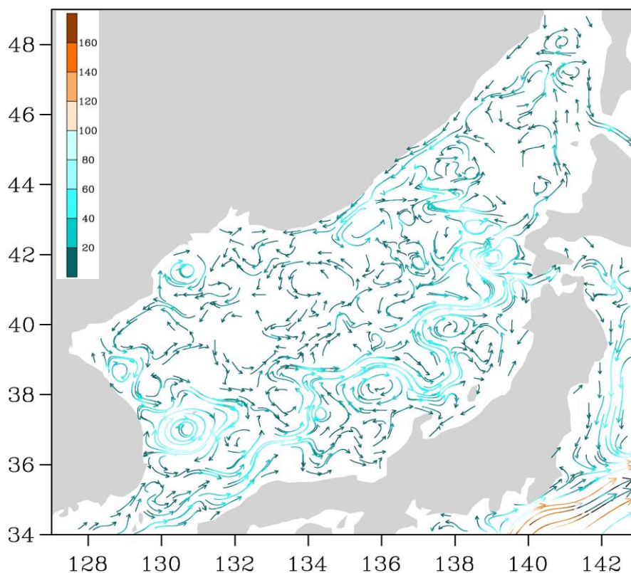
Рис. 3-1 Поверхностные течения Японского моря, 05 февраля 2016 г.
