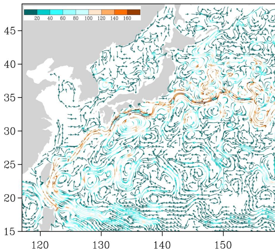
Рис. 3-6 Поверхностные течения западной части Тихого океана, 25 февраля 2016 г.
