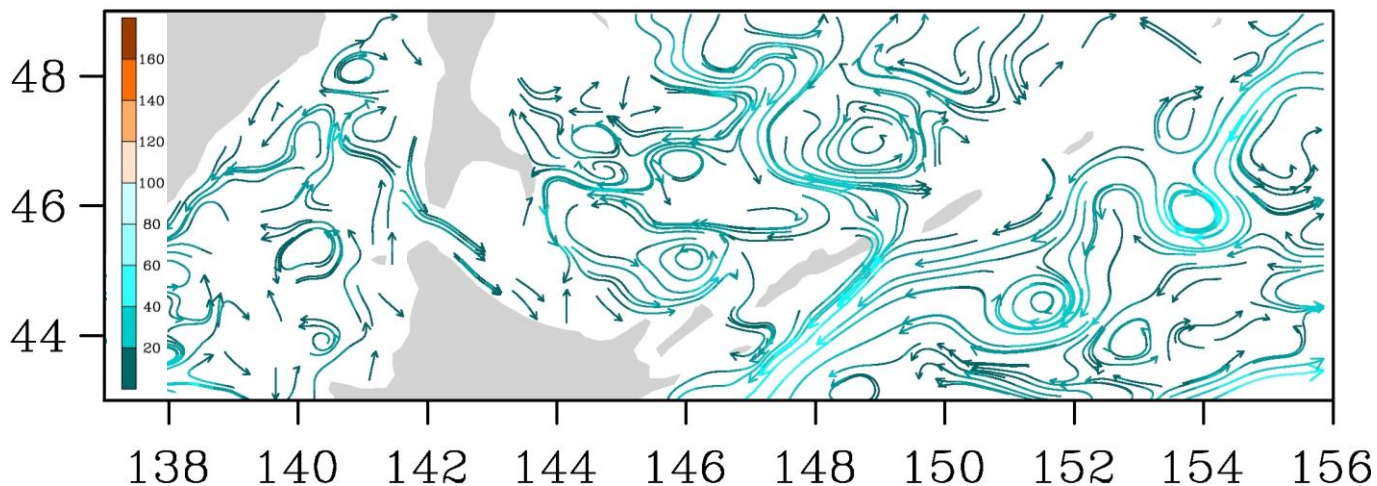
Рис. 3-7 Поверхностные течения, пролив Лаперуза, 5 февраля 2016 г.
