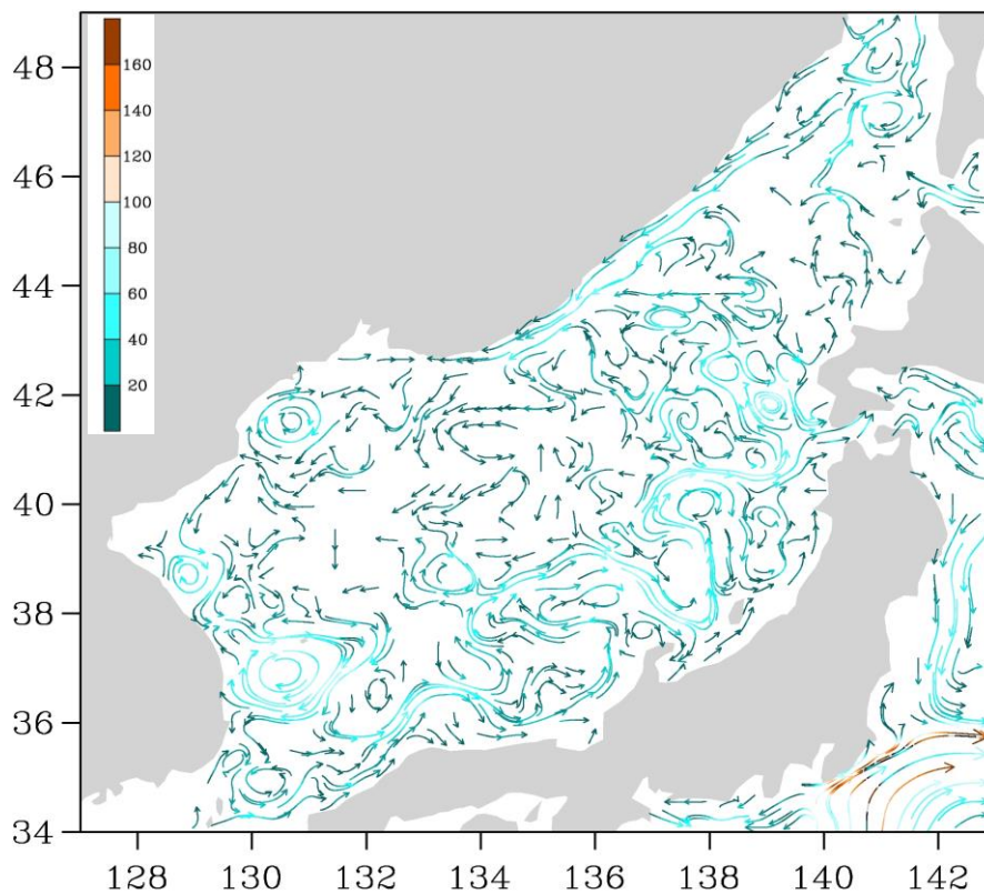
Рис. 3-2 Поверхностные течения Японского моря, 15 февраля 2016 г.
