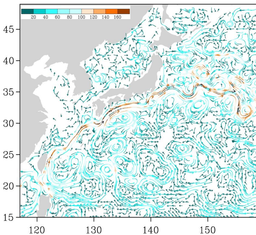
Рис. 3-4 Поверхностные течения западной части Тихого океана, 5 февраля 2016 г.
