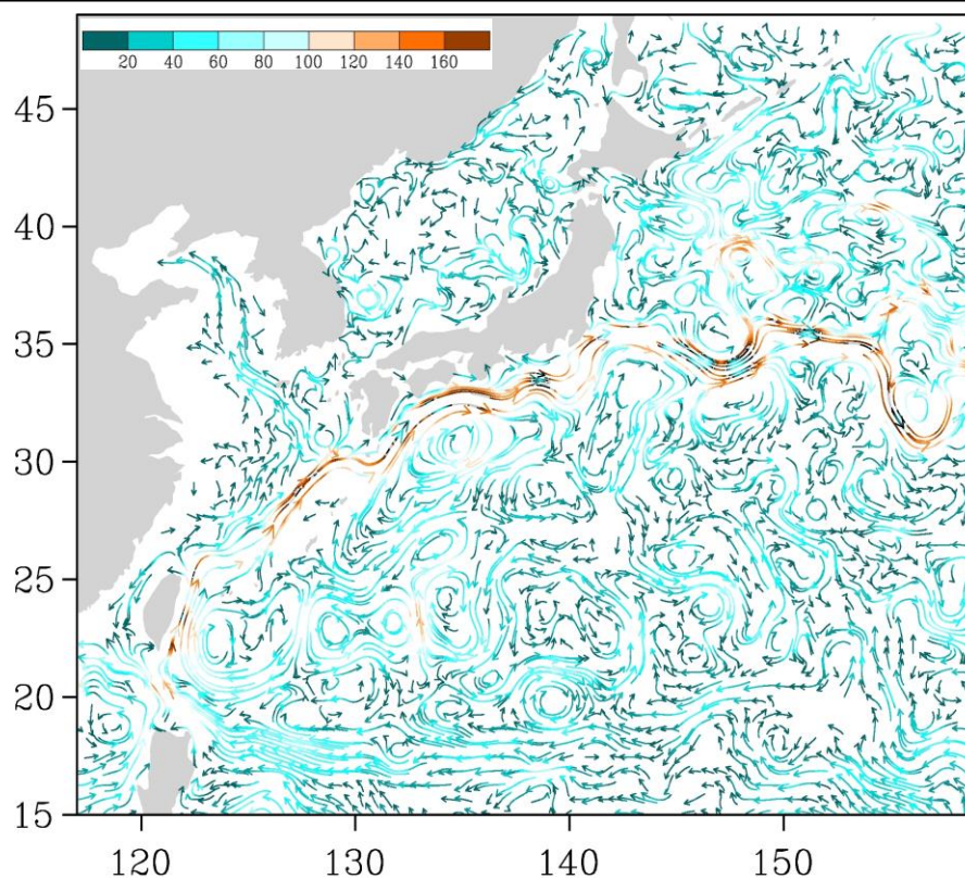
Рис. 3-5 Поверхностные течения западной части Тихого океана, 15 февраля 2016 г.
