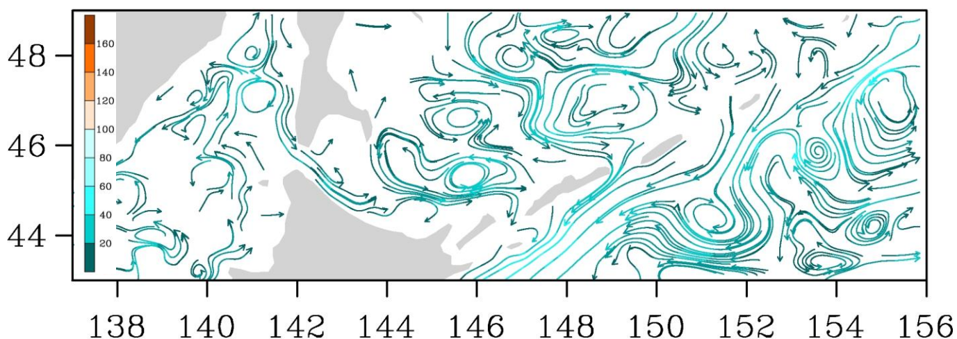
Рис. 3-9 Поверхностные течения, пролив Лаперуза, 25 февраля 2016 г.
