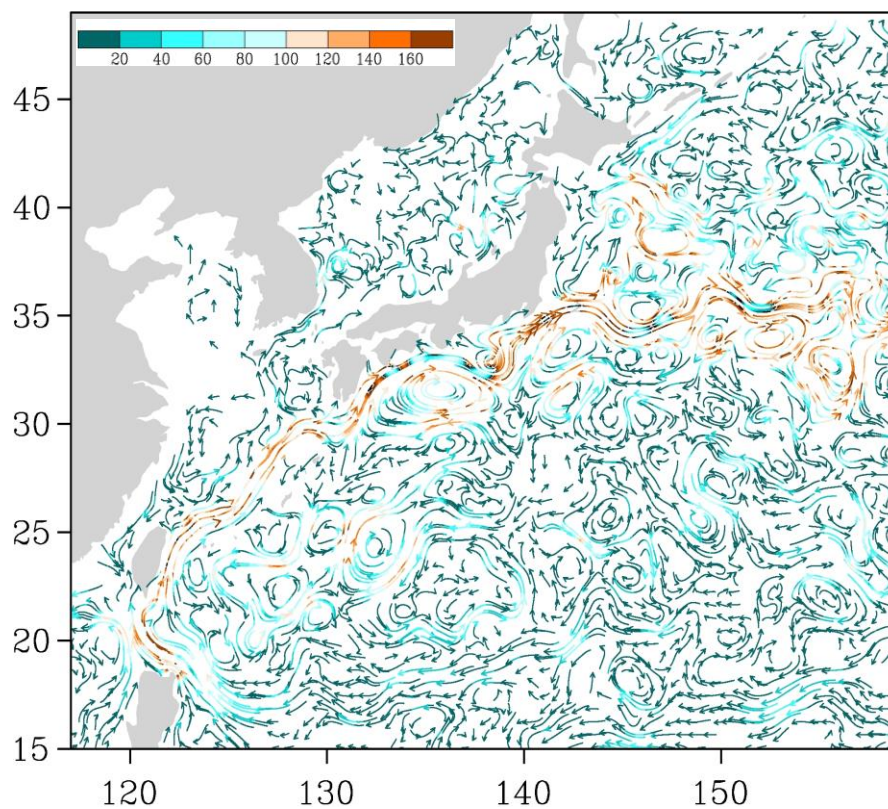
Рис. 3-6 Поверхностные течения западной части Тихого океана, 25 марта 2016 г.
