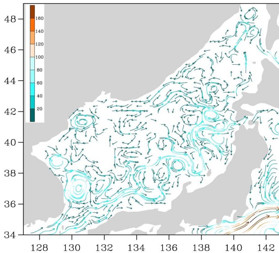
Рис. 3-2 Поверхностные течения Японского моря, 15 марта 2016 г.
