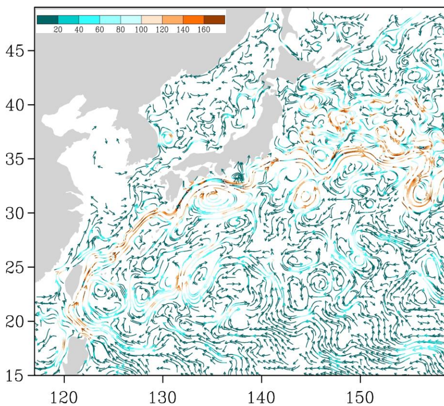
Рис. 3-4 Поверхностные течения западной части Тихого океана, 5 марта 2016 г.
