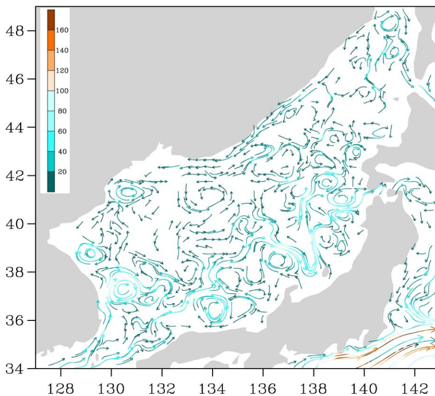
Рис. 3-3 Поверхностные течения Японского моря, 25 марта 2016 г.
