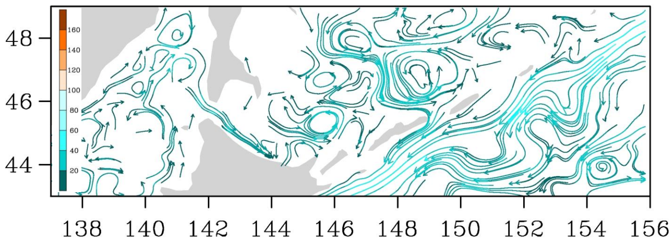
Рис. 3-7 Поверхностные течения, пролив Лаперуза, 5 марта 2016 г.
