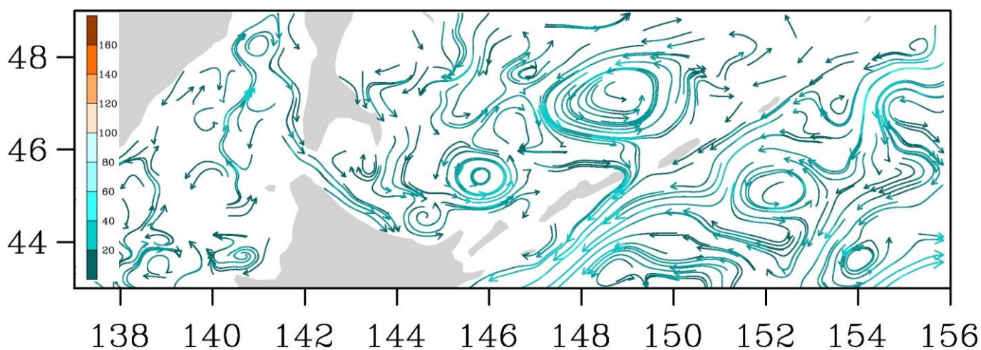
Рис. 3-9 Поверхностные течения, пролив Лаперуза, 25 марта 2016 г.
