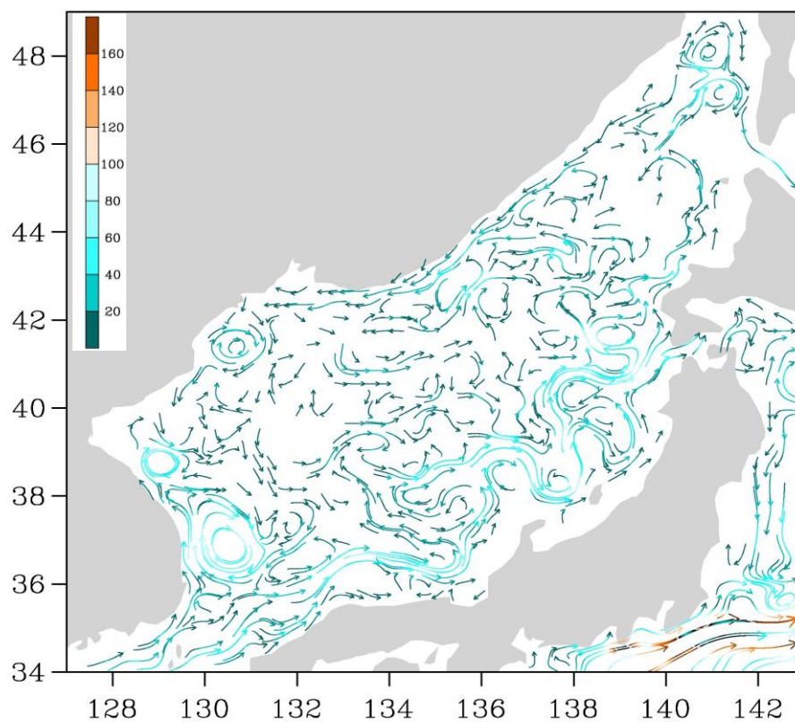
Рис. 3-1 Поверхностные течения Японского моря, 05 марта 2016 г.
