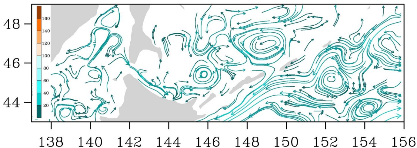
Рис. 3-8 Поверхностные течения, пролив Лаперуза, 15 марта 2016 г.
