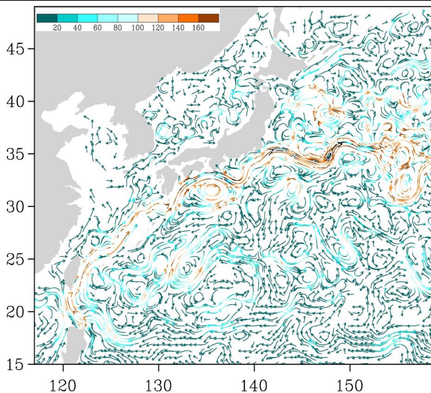
Рис. 3-5 Поверхностные течения западной части Тихого океана, 15 марта 2016 г.
