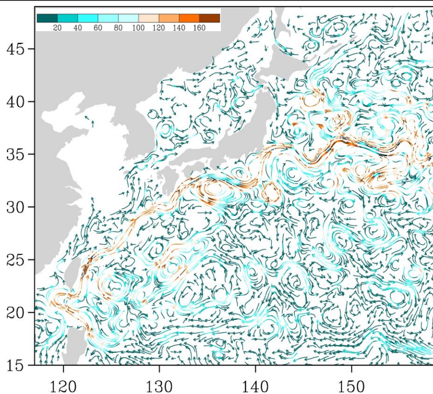
Рис. 3-5 Поверхностные течения западной части Тихого океана, 15 апреля 2016 г.
