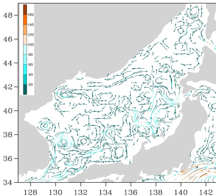
Рис. 3-1 Поверхностные течения Японского моря, 05 апреля 2016 г.
