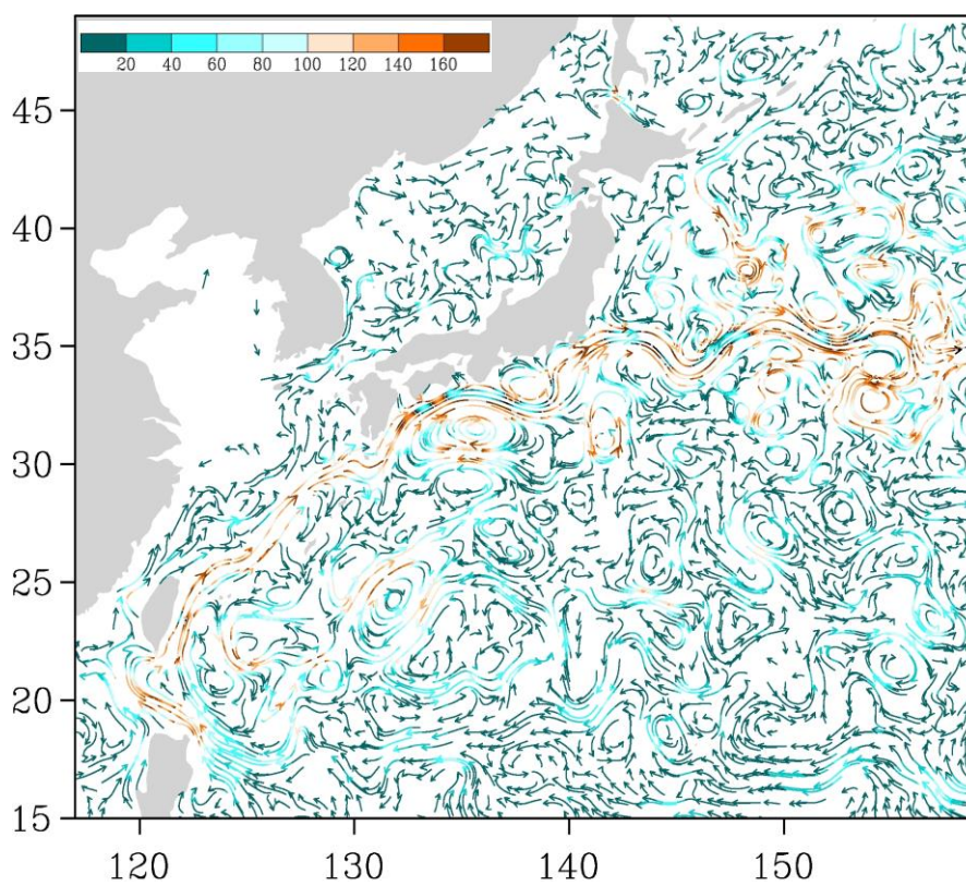
Рис. 3-4 Поверхностные течения западной части Тихого океана, 5 апреля 2016 г.
