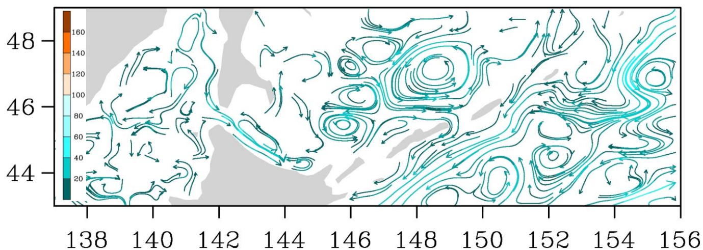
Рис. 3-9 Поверхностные течения, пролив Лаперуза, 25 апреля 2016 г.
