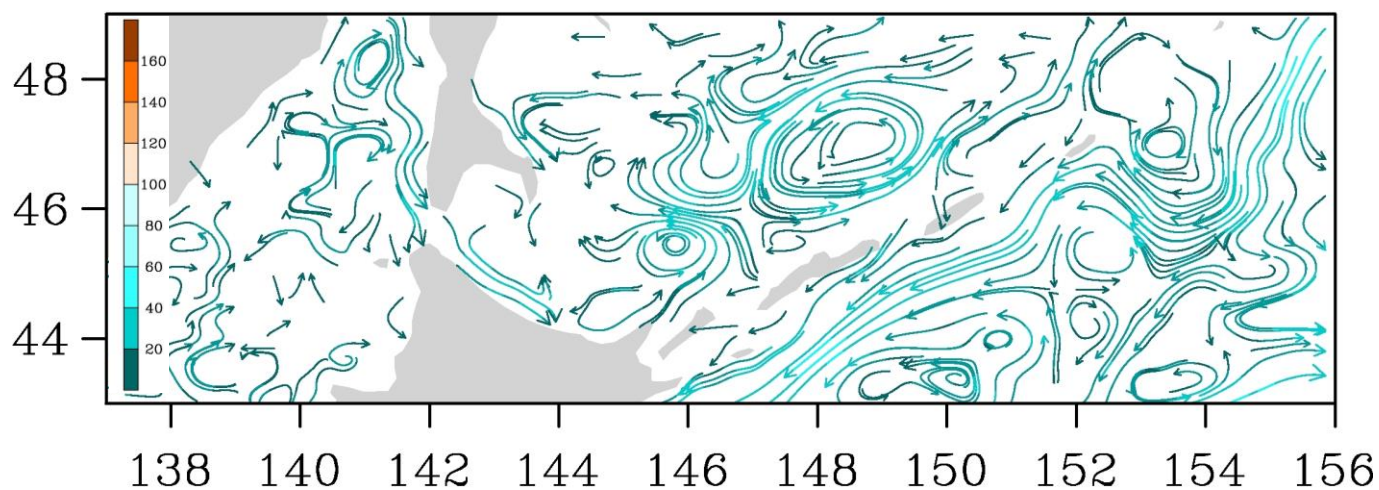
Рис. 3-8 Поверхностные течения, пролив Лаперуза, 15 апреля 2016 г.
