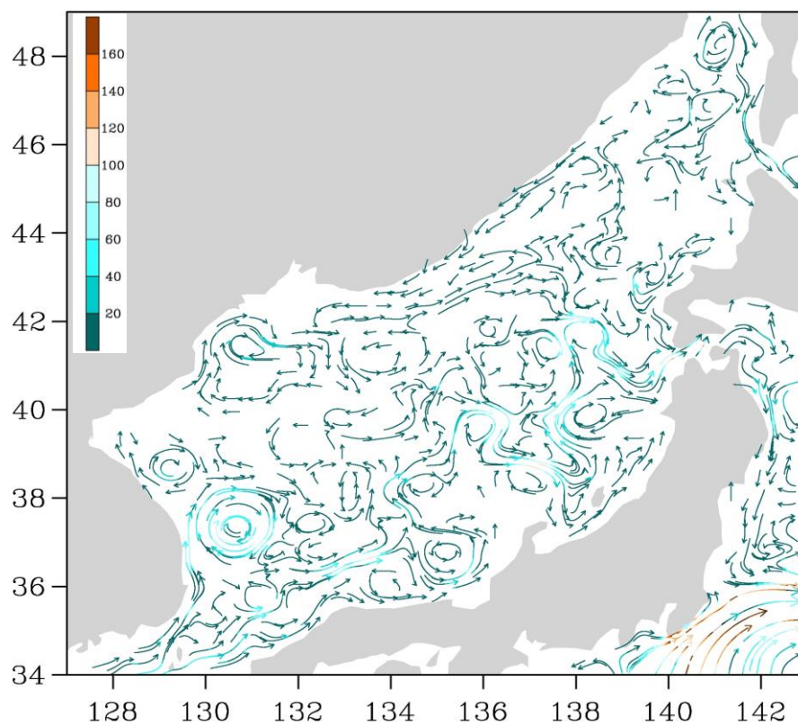
Рис. 3-2 Поверхностные течения Японского моря, 15 апреля 2016 г.
