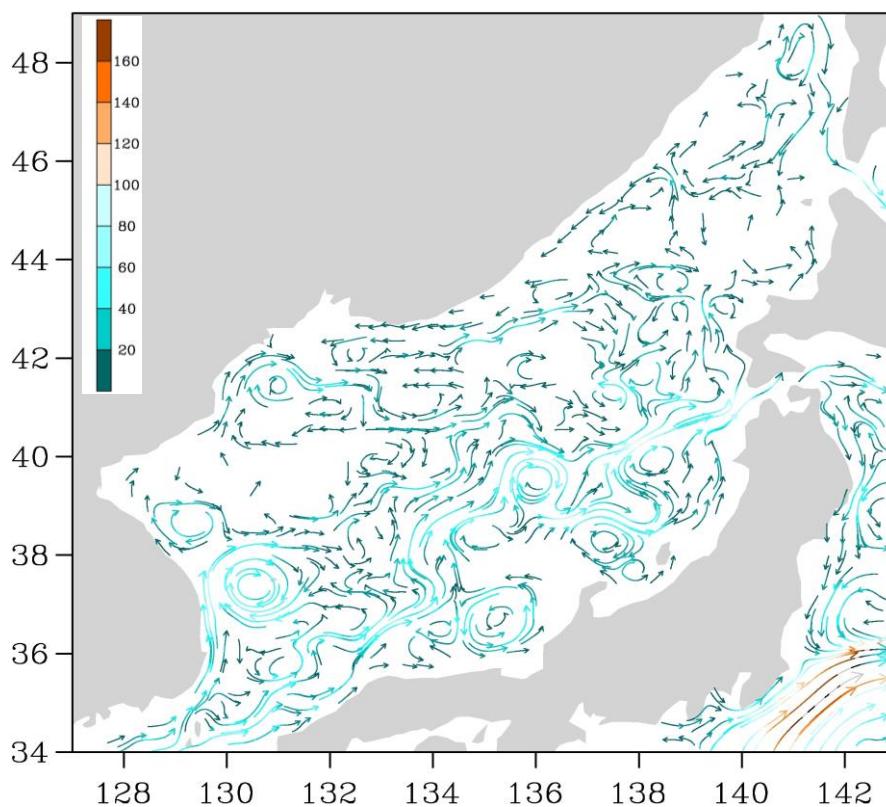
Рис. 3-3 Поверхностные течения Японского моря, 25 апреля 2016 г.
