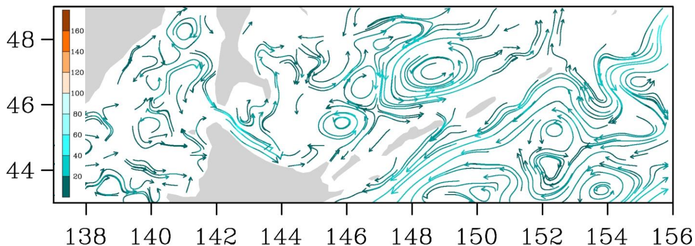
Рис. 3-7 Поверхностные течения, пролив Лаперуза, 5 апреля 2016 г.
