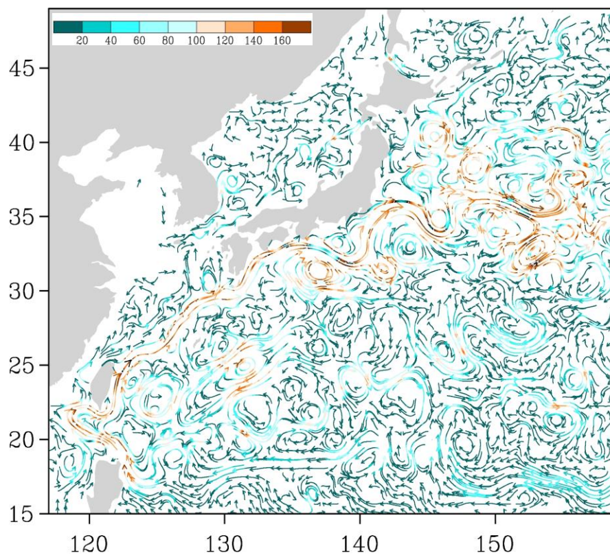
Рис. 3-6 Поверхностные течения западной части Тихого океана, 25 апреля 2016 г.
