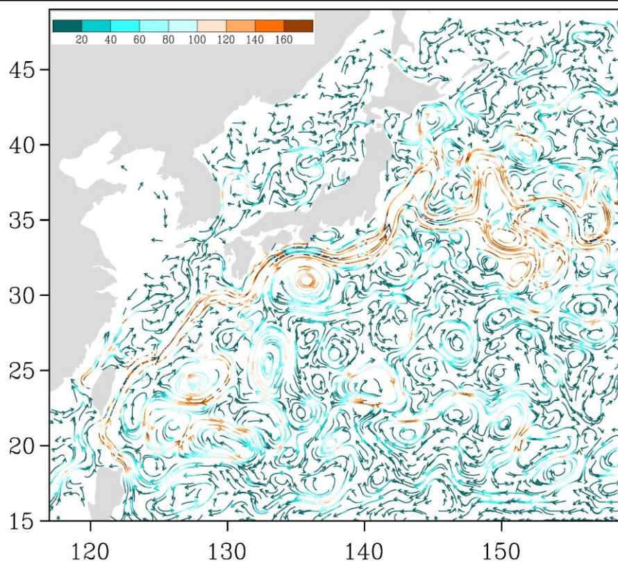
Рис. 3-5 Поверхностные течения западной части Тихого океана, 15 июля 2016 г.
