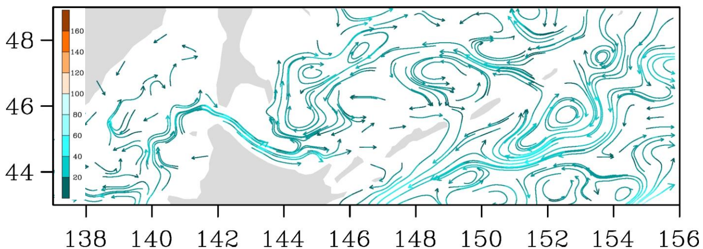
Рис. 3-8 Поверхностные течения, пролив Лаперуза, 15 июля 2016 г.
