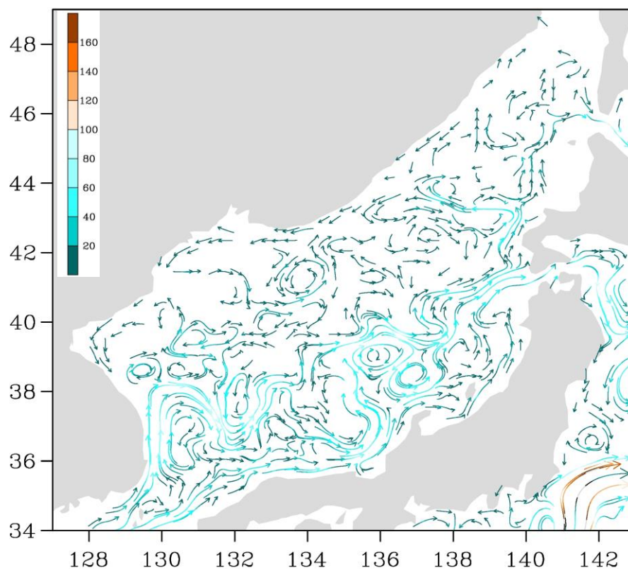
Рис. 3-1 Поверхностные течения Японского моря, 05 июля 2016 г.
