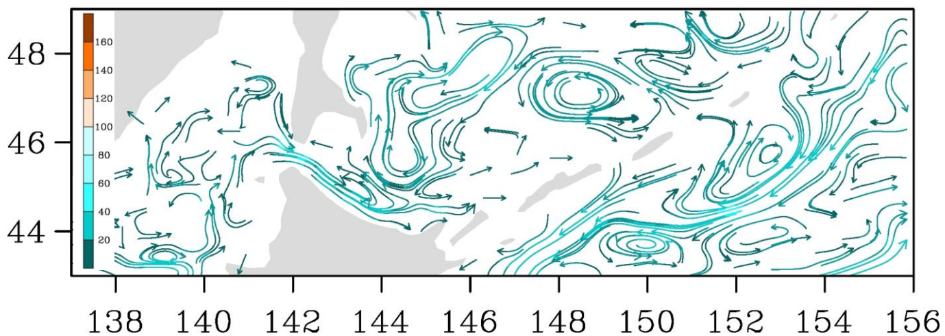
Рис. 3-7 Поверхностные течения, пролив Лаперуза, 5 июля 2016 г.
