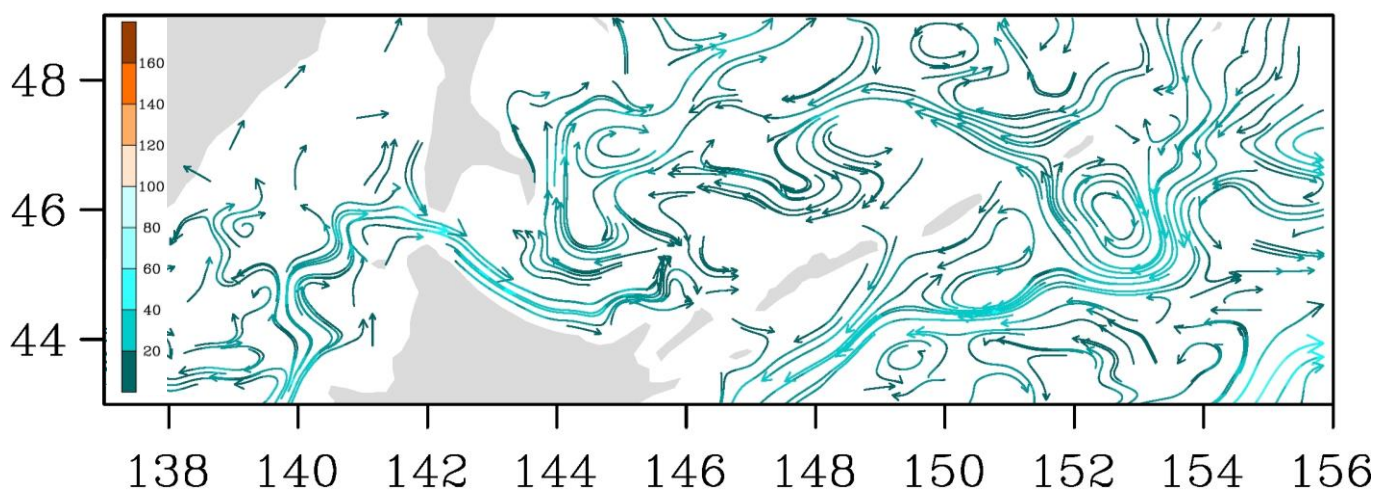
Рис. 3-9 Поверхностные течения, пролив Лаперуза, 25 июля 2016 г.
