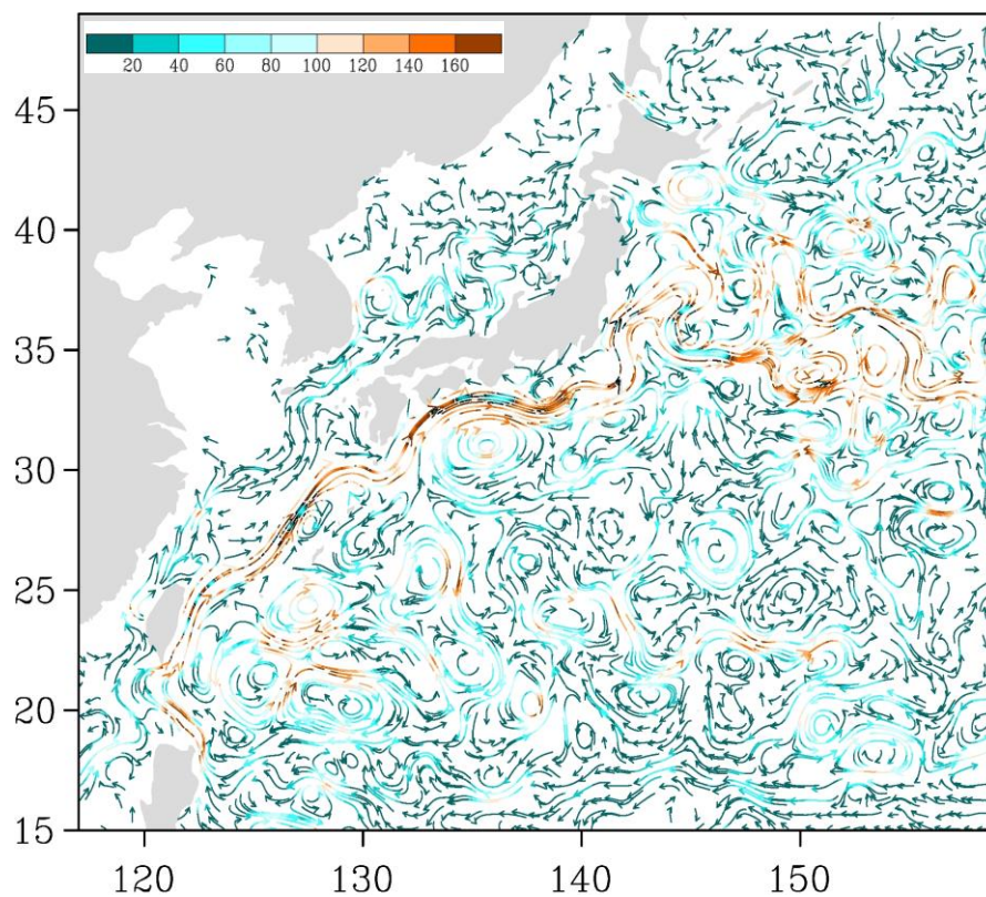
Рис. 3-6 Поверхностные течения западной части Тихого океана, 25 июля 2016 г.
