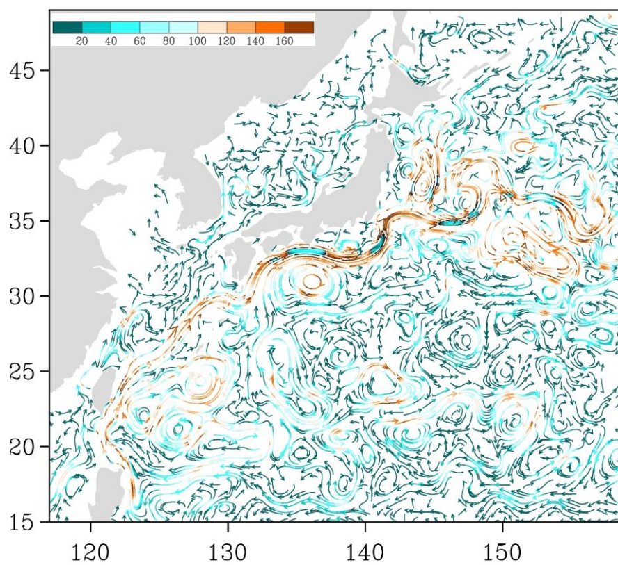
Рис. 3-4 Поверхностные течения западной части Тихого океана, 5 июля 2016 г.
