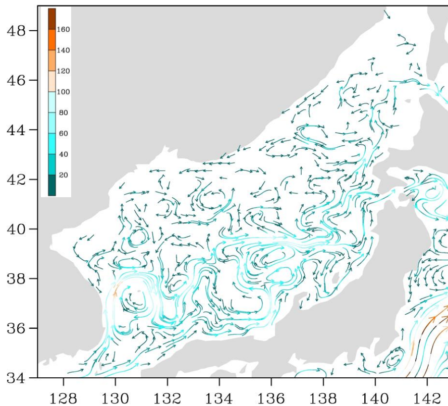
Рис. 3-2 Поверхностные течения Японского моря, 15 июля 2016 г.
