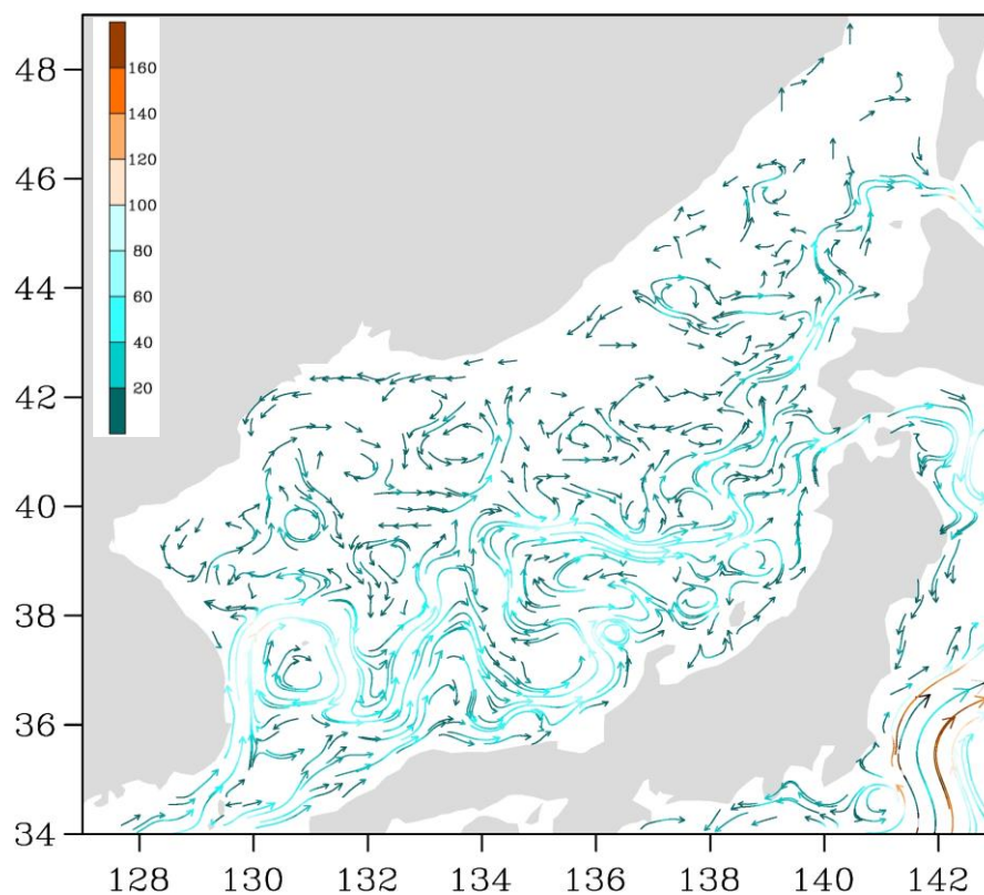
Рис. 3-3 Поверхностные течения Японского моря, 25 июля 2016 г.
