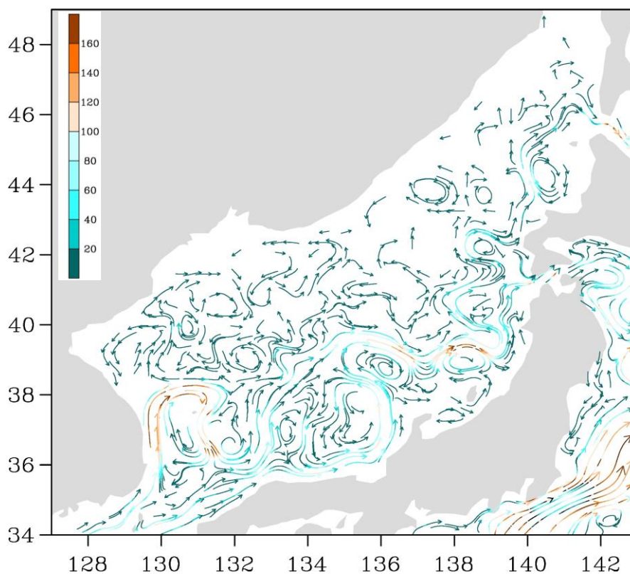
Рис. 3-3 Поверхностные течения Японского моря, 25 августа 2016 г.
