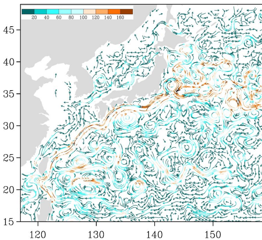
Рис. 3-4 Поверхностные течения западной части Тихого океана, 5 августа 2016 г.
