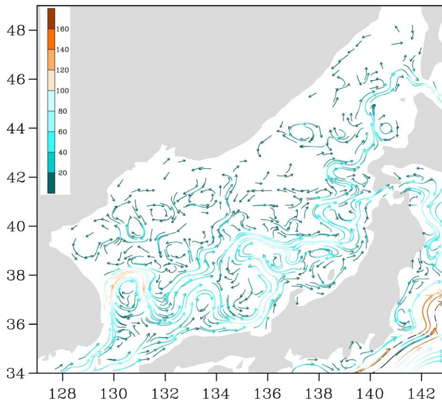
Рис. 3-2 Поверхностные течения Японского моря, 15 августа 2016 г.
