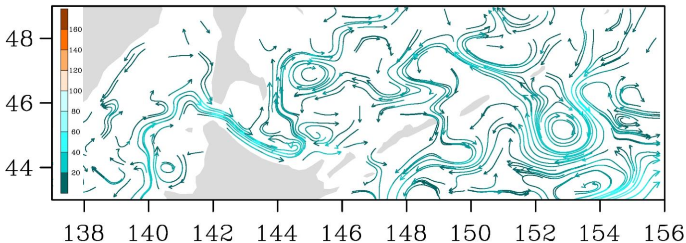
Рис. 3-8 Поверхностные течения, пролив Лаперуза, 15 августа 2016 г.
