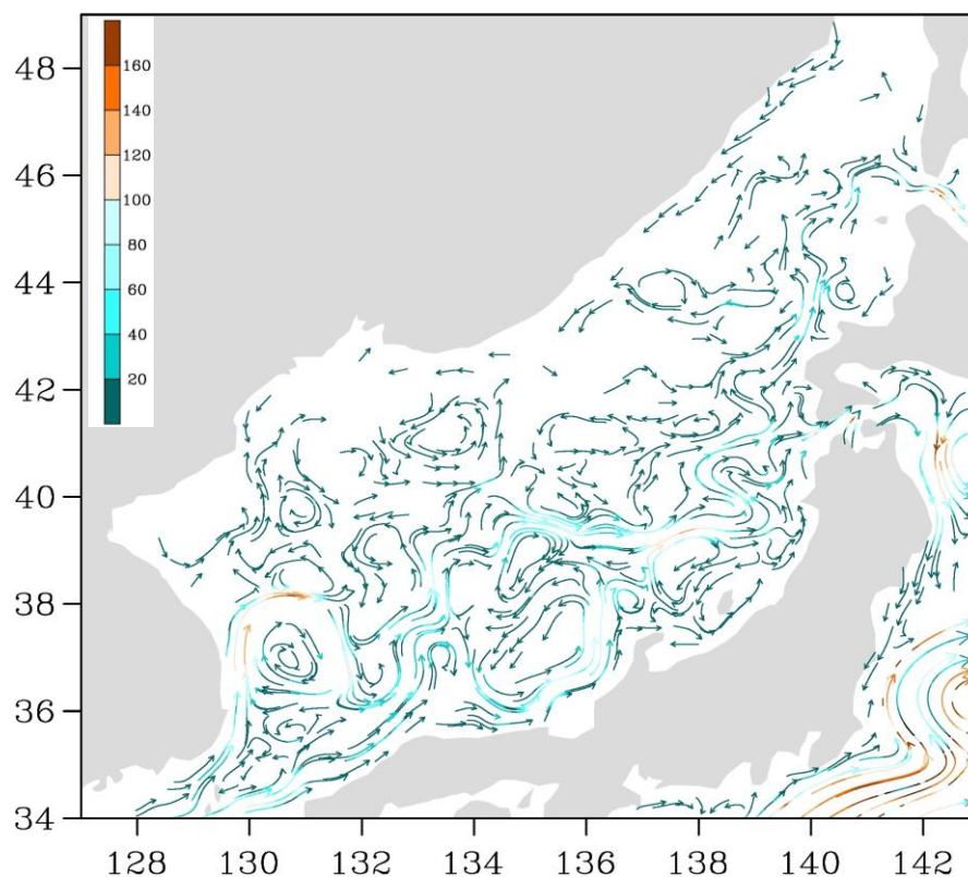
Рис. 3-1 Поверхностные течения Японского моря, 05 августа 2016 г.
