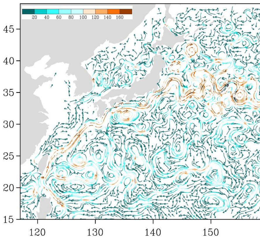
Рис. 3-6 Поверхностные течения западной части Тихого океана, 25 августа 2016 г.
