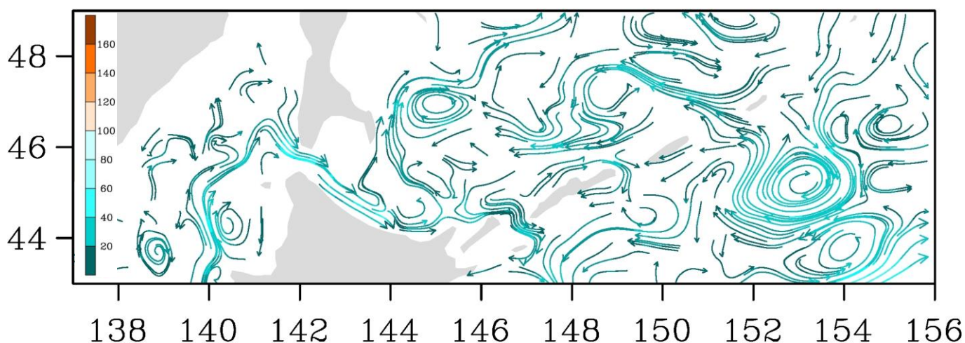
Рис. 3-9 Поверхностные течения, пролив Лаперуза, 25 августа 2016 г.
