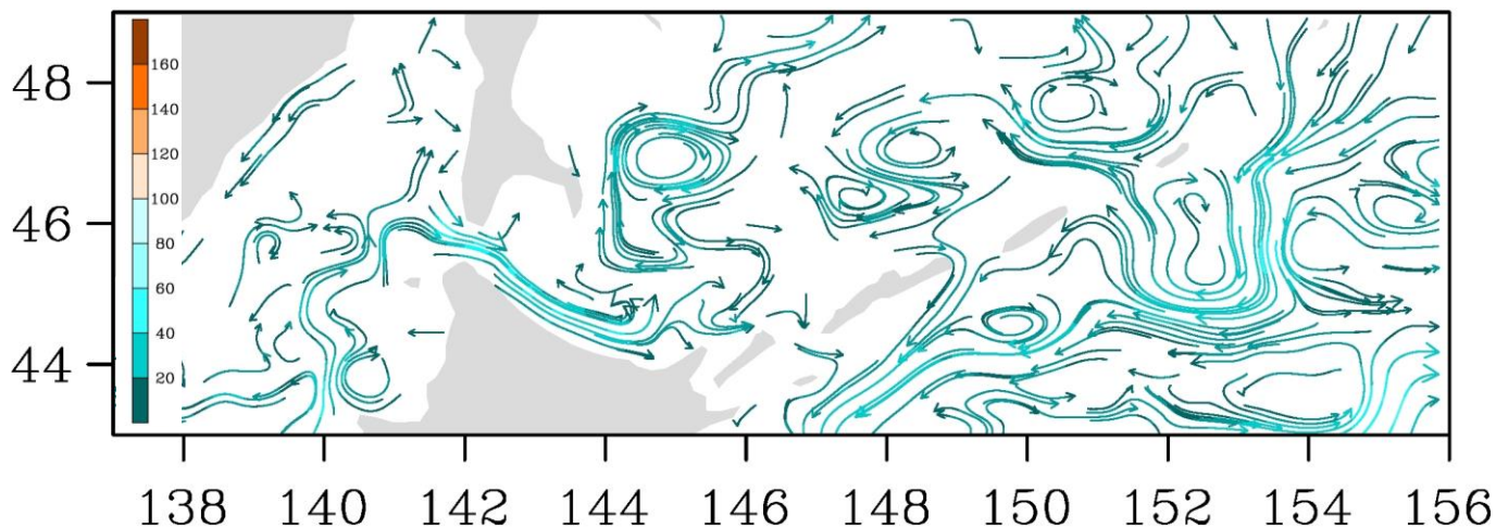
Рис. 3-7 Поверхностные течения, пролив Лаперуза, 5 августа 2016 г.
