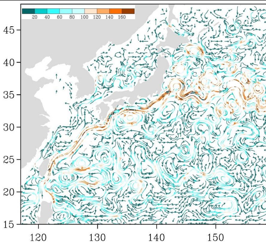
Рис. 3-5 Поверхностные течения западной части Тихого океана, 15 августа 2016 г.
