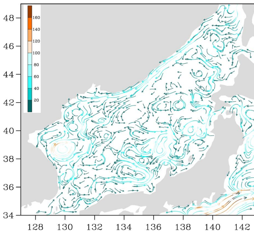
Рис. 3-3 Поверхностные течения Японского моря, 25 января 2018 г.
