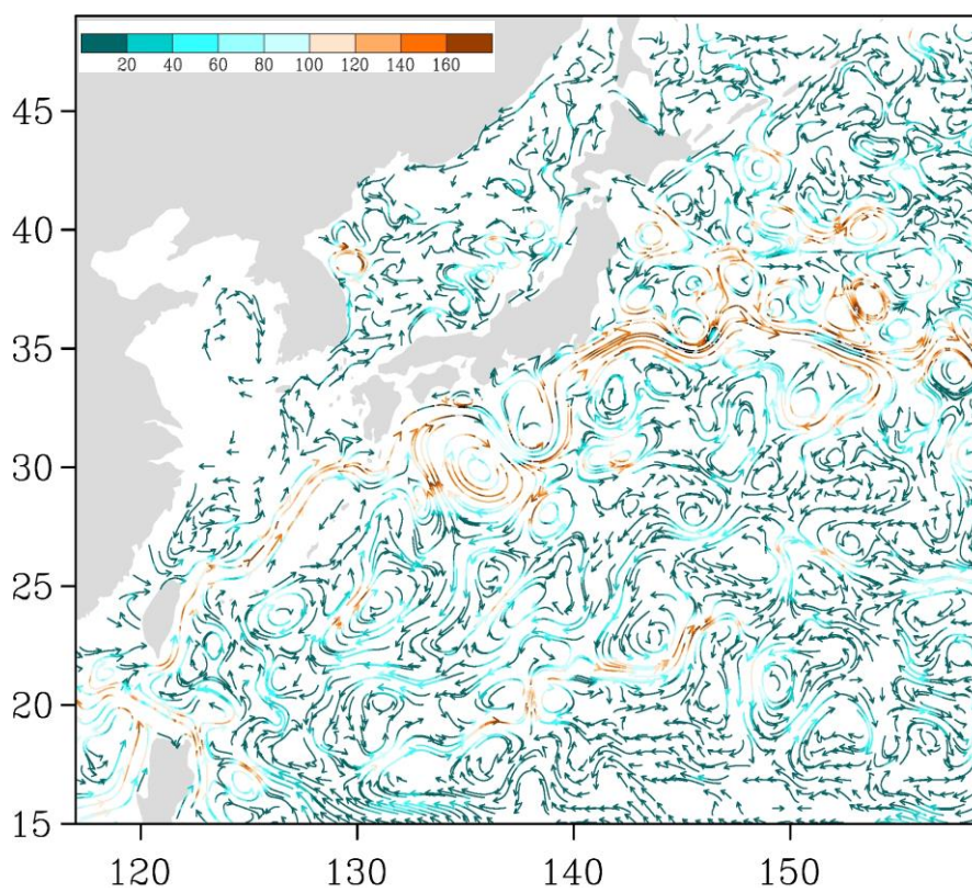
Рис. 3-4 Поверхностные течения западной части Тихого океана, 5 января 2018 г.
