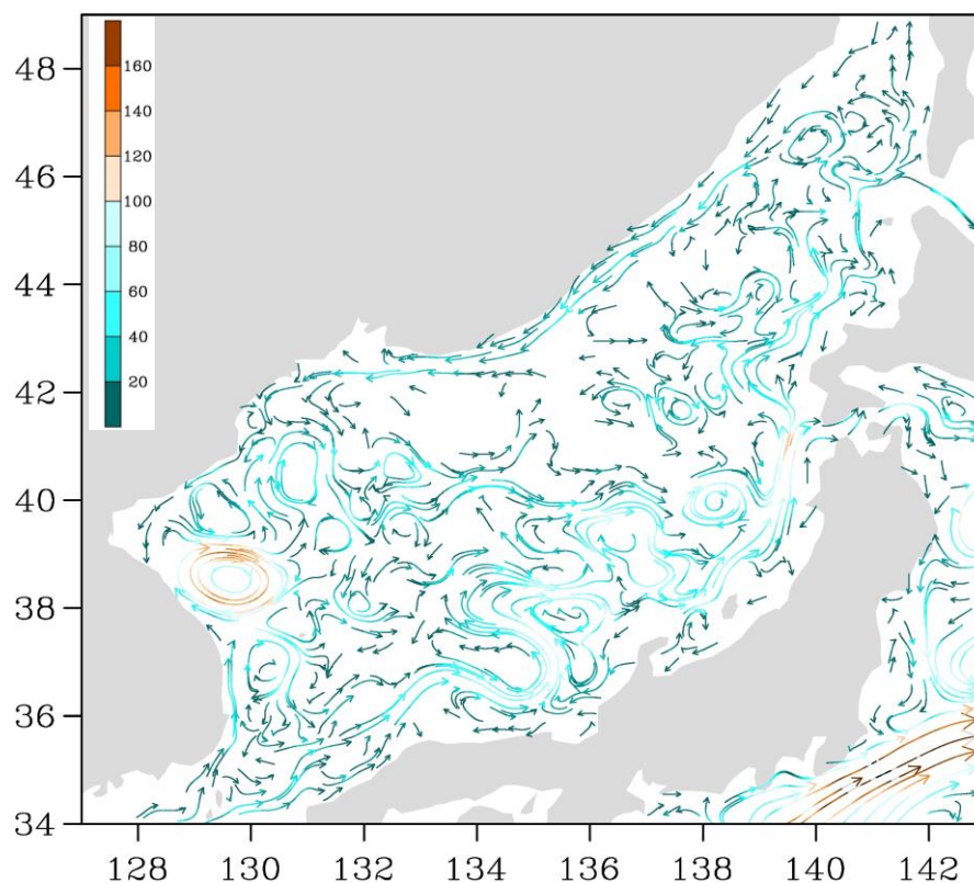
Рис. 3-1 Поверхностные течения Японского моря, 05 января 2018 г.
