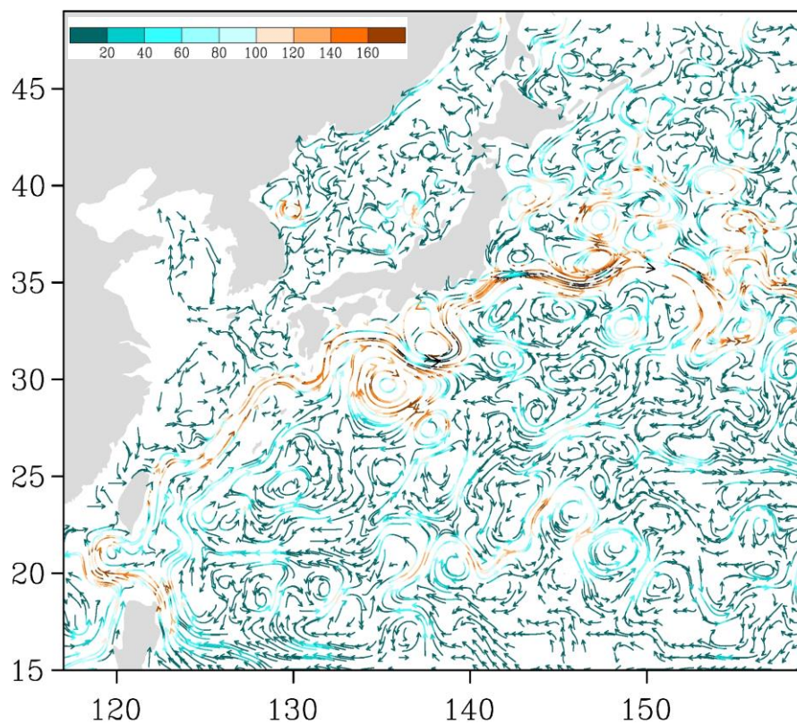
Рис. 3-6 Поверхностные течения западной части Тихого океана, 25 января 2018 г.
