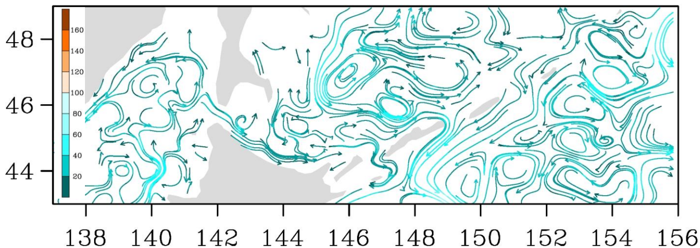
Рис. 3-8 Поверхностные течения, пролив Лаперуза, 15 января 2018 г.
