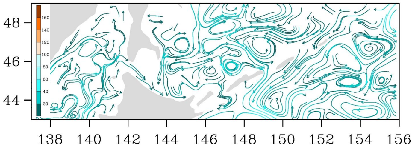
Рис. 3-7 Поверхностные течения, пролив Лаперуза, 5 января 2018 г.
