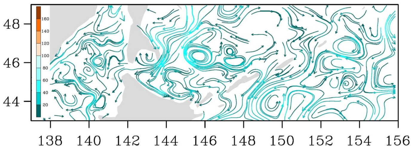
Рис. 3-9 Поверхностные течения, пролив Лаперуза, 25 января 2018 г.
