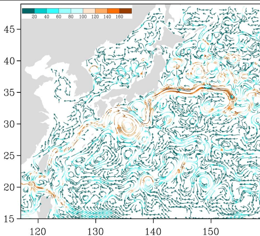
Рис. 3-5 Поверхностные течения западной части Тихого океана, 15 января 2018 г.
