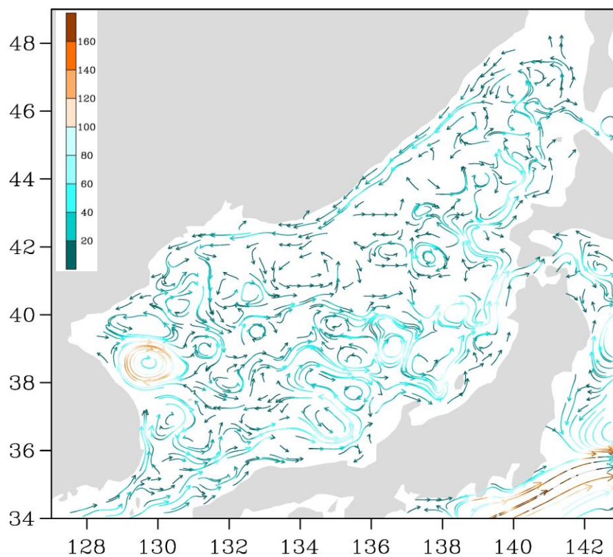
Рис. 3-2 Поверхностные течения Японского моря, 15 января 2018 г.
