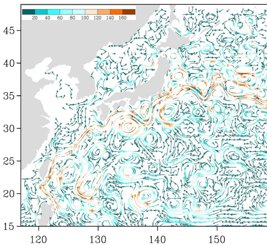
Рис. 3-4 Поверхностные течения западной части Тихого океана, 5 ноября 2018 г.
