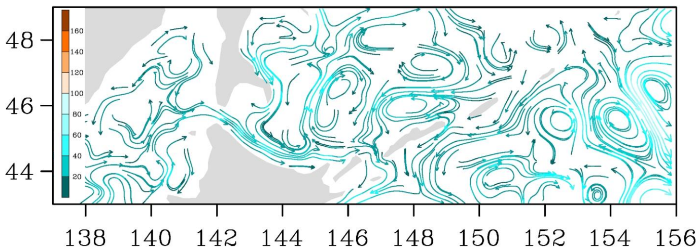
Рис. 3-8 Поверхностные течения, пролив Лаперуза, 15 ноября 2018 г.
