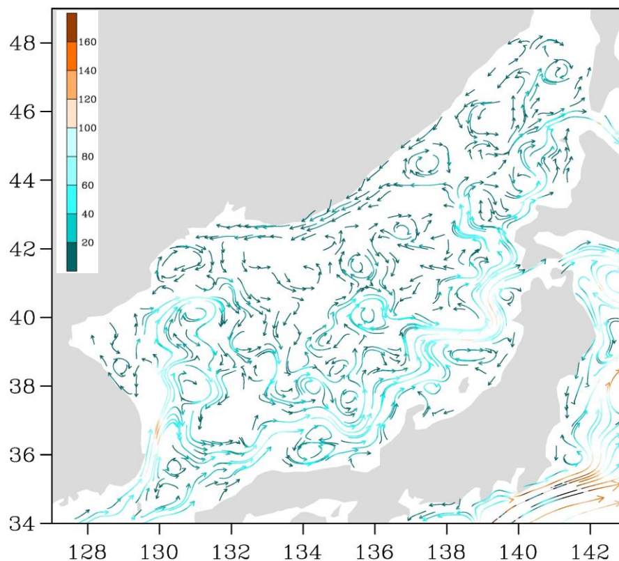
Рис. 3-1 Поверхностные течения Японского моря, 05 ноября 2018 г.
