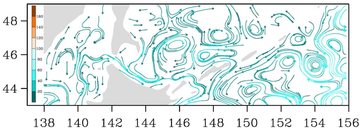
Рис. 3-9 Поверхностные течения, пролив Лаперуза, 25 ноября 2018 г.
