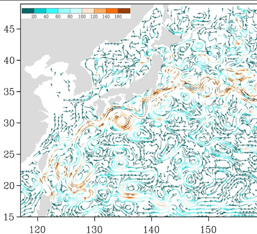
Рис. 3-5 Поверхностные течения западной части Тихого океана, 15 ноября 2018 г.
