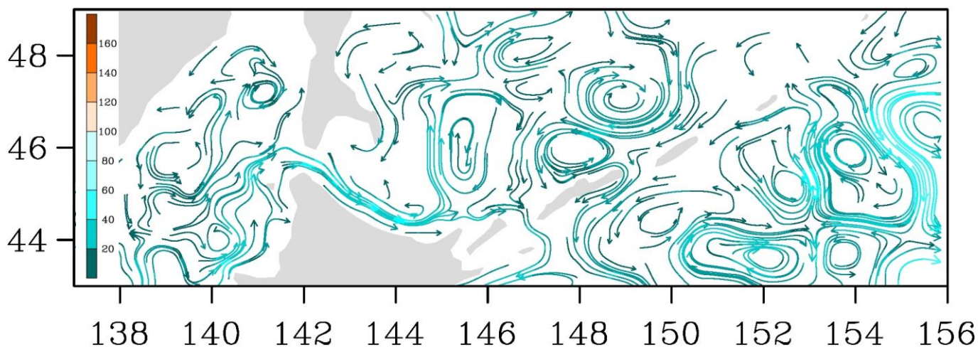
Рис. 3-7 Поверхностные течения, пролив Лаперуза, 5 ноября 2018 г.
