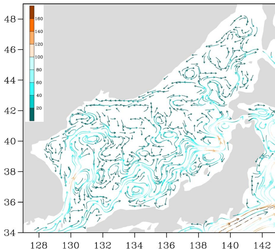
Рис. 3-2 Поверхностные течения Японского моря, 15 ноября 2018 г.
