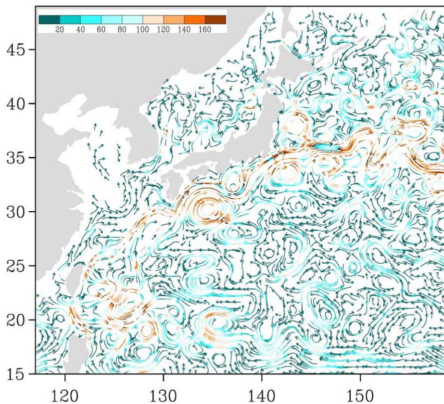
Рис. 3-6 Поверхностные течения западной части Тихого океана, 25 ноября 2018 г.
