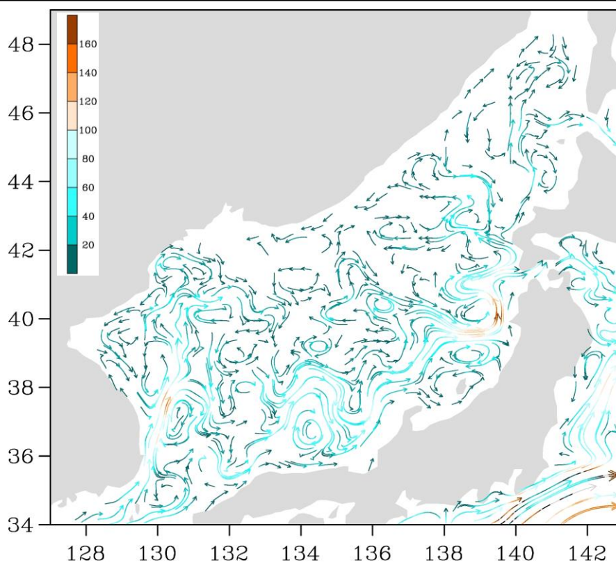
Рис. 3-3 Поверхностные течения Японского моря, 25 ноября 2018 г.
