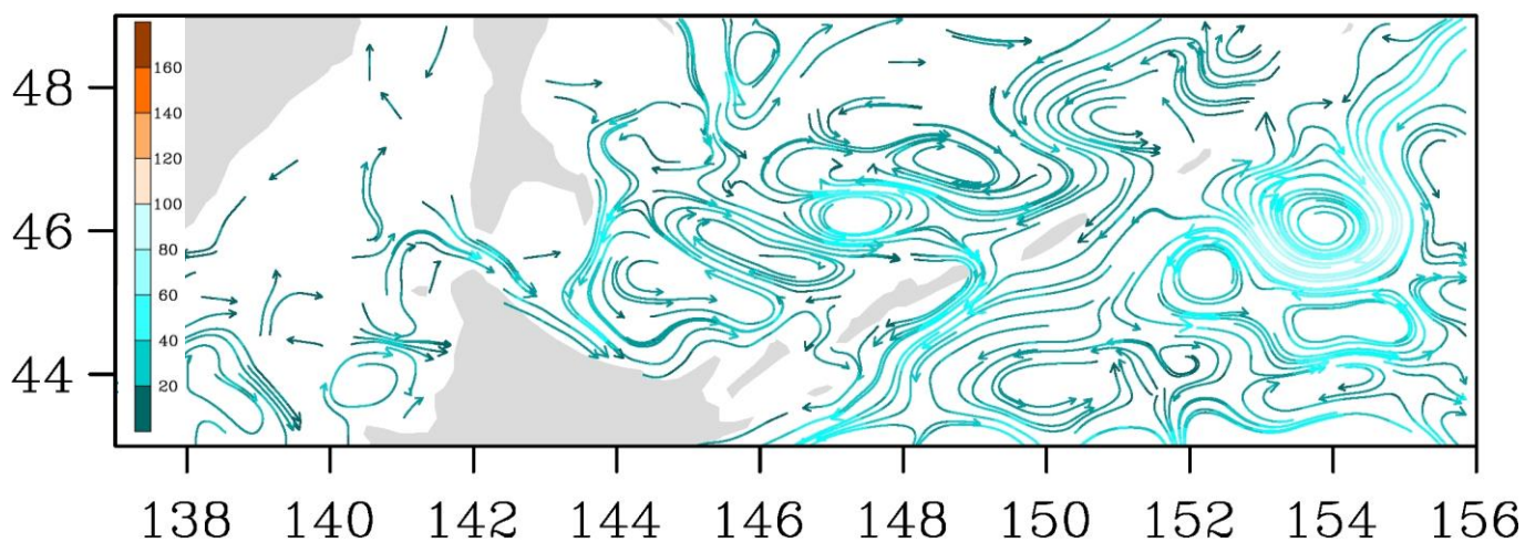
Рис. 3-8 Поверхностные течения, пролив Лаперуза, 15 декабря 2018 г.
