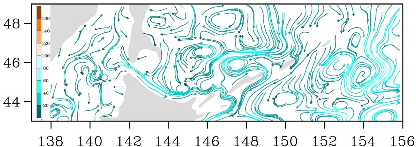
Рис. 3-7 Поверхностные течения, пролив Лаперуза, 5 декабря 2018 г.
