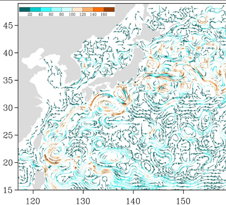
Рис. 3-5 Поверхностные течения западной части Тихого океана, 15 декабря 2018 г.
