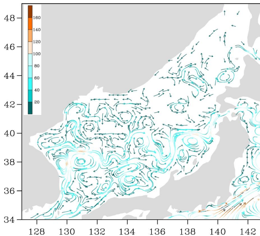
Рис. 3-2 Поверхностные течения Японского моря, 15 декабря 2018 г.
