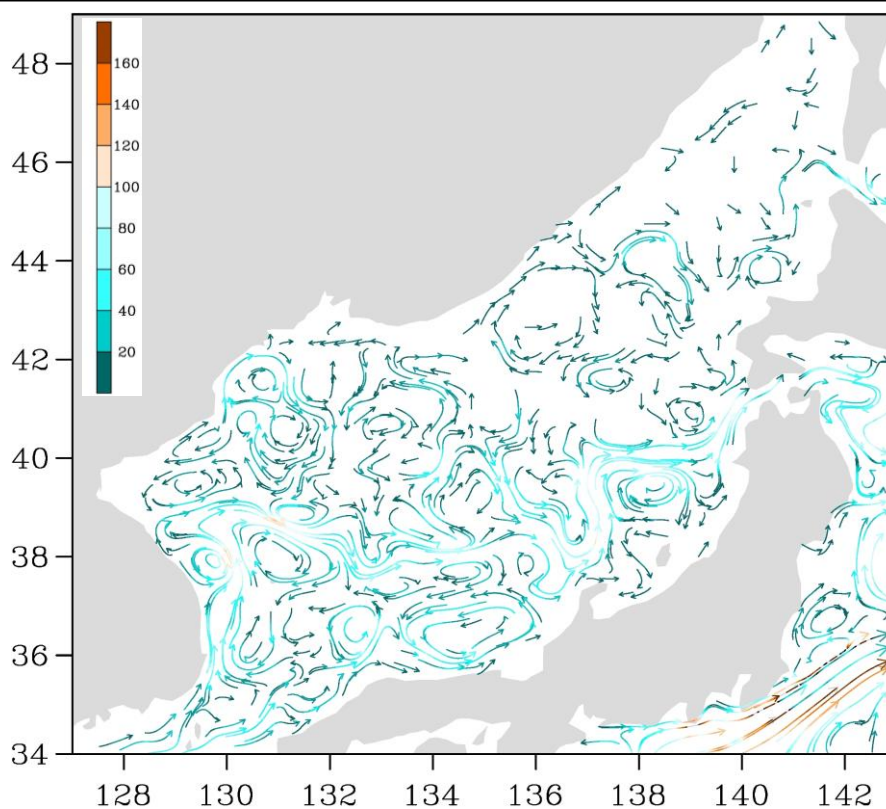
Рис. 3-3 Поверхностные течения Японского моря, 25 декабря 2018 г.
