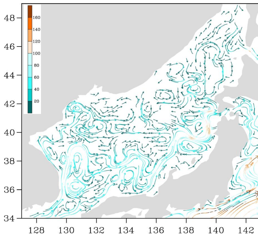
Рис. 3-1 Поверхностные течения Японского моря, 05 декабря 2018 г.
