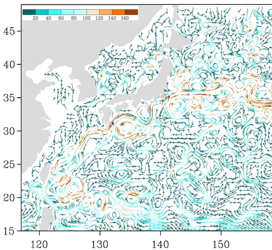
Рис. 3-4 Поверхностные течения западной части Тихого океана, 5 декабря 2018 г.
