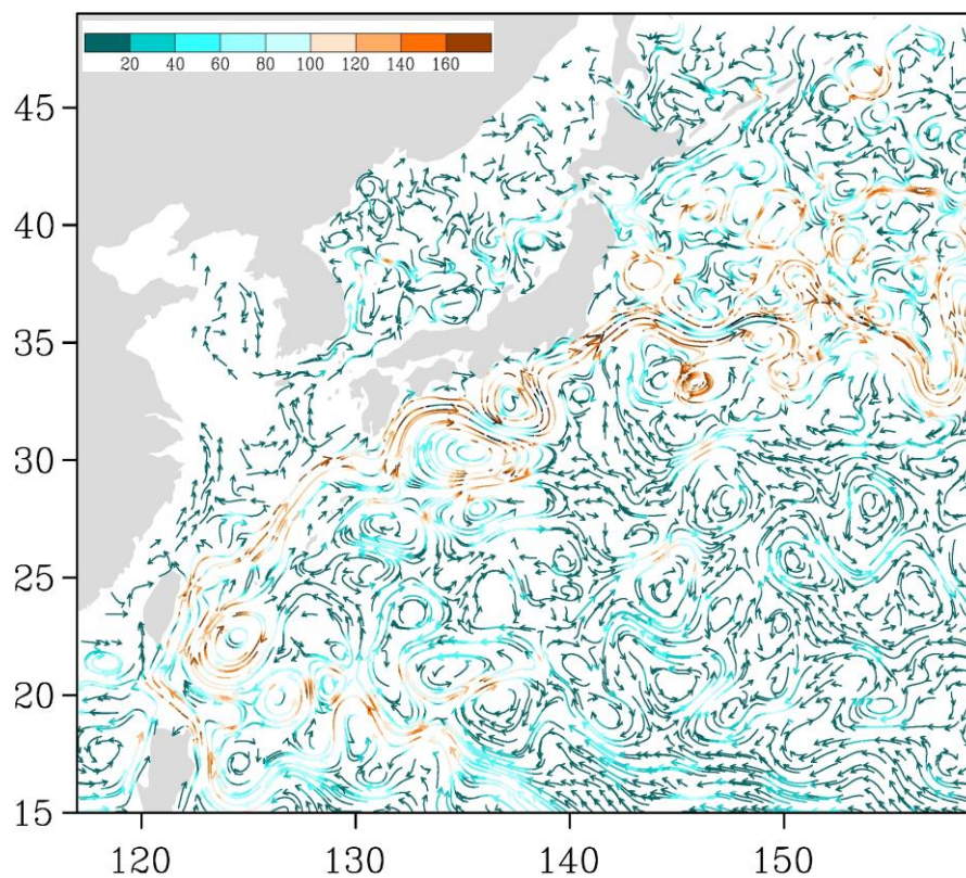
Рис. 3-6 Поверхностные течения западной части Тихого океана, 25 декабря 2018 г.
