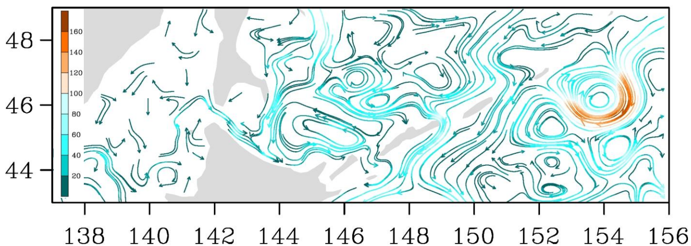
Рис. 3-9 Поверхностные течения, пролив Лаперуза, 25 декабря 2018 г.
