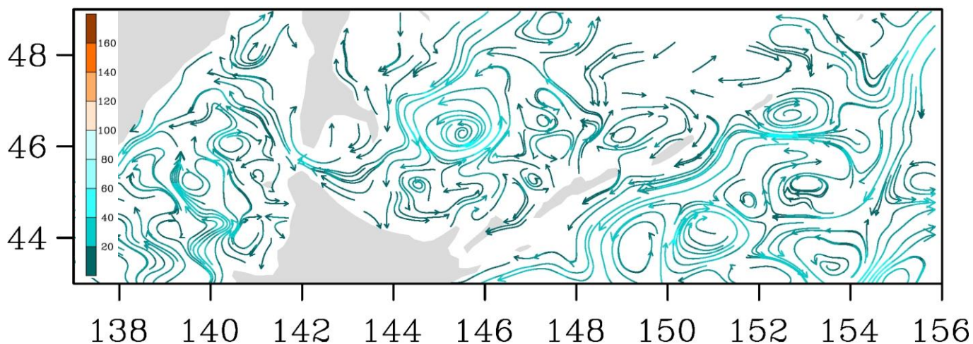
Рис. 3-7 Поверхностные течения, пролив Лаперуза, 5 февраля 2018 г.
