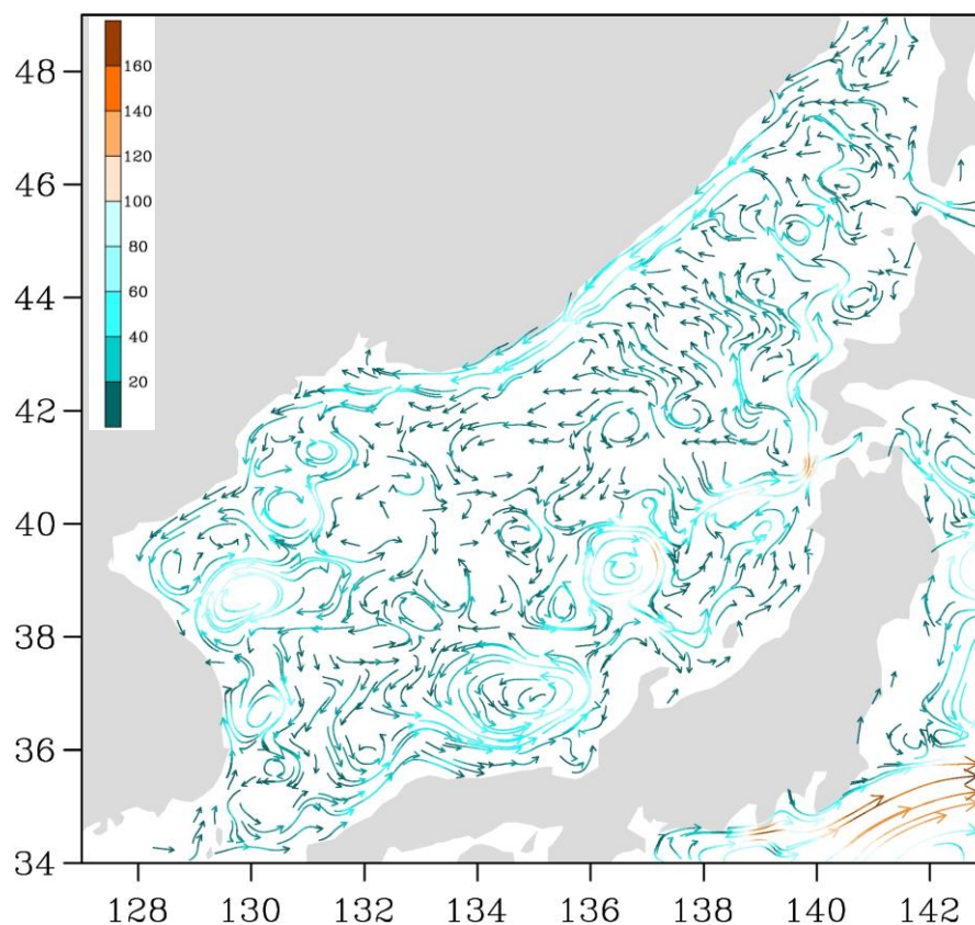
Рис. 3-1 Поверхностные течения Японского моря, 05 февраля 2018 г.
