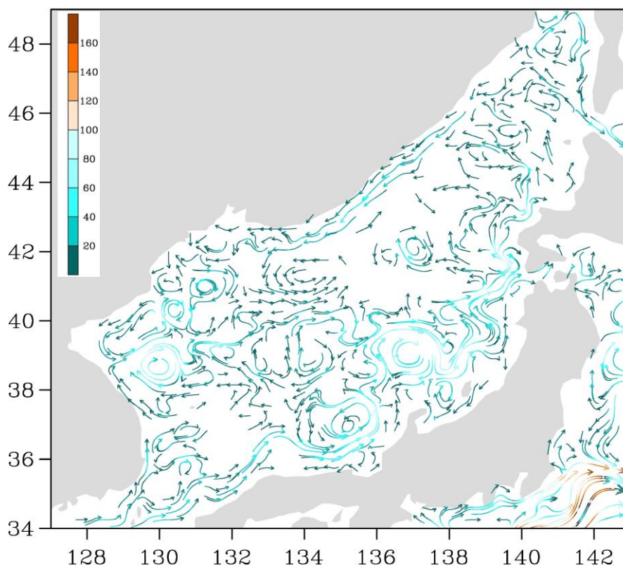
Рис. 3-3 Поверхностные течения Японского моря, 25 февраля 2018 г.
