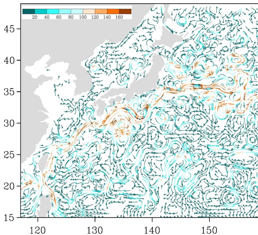
Рис. 3-6 Поверхностные течения западной части Тихого океана, 25 февраля 2018 г.
