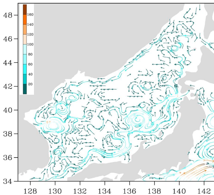
Рис. 3-2 Поверхностные течения Японского моря, 15 февраля 2018 г.
