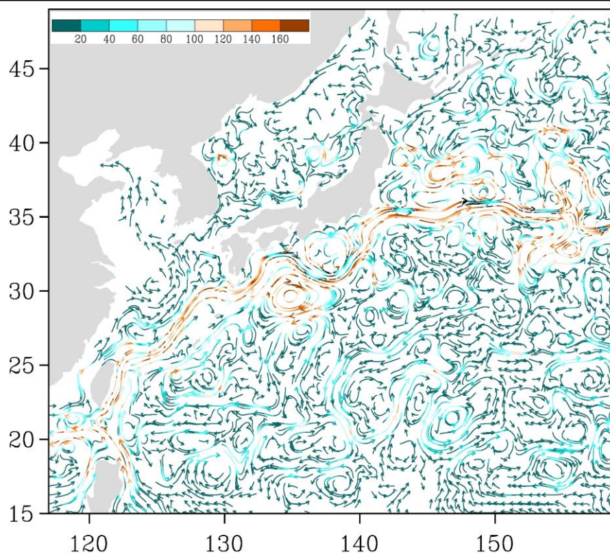
Рис. 3-5 Поверхностные течения западной части Тихого океана, 15 февраля 2018 г.
