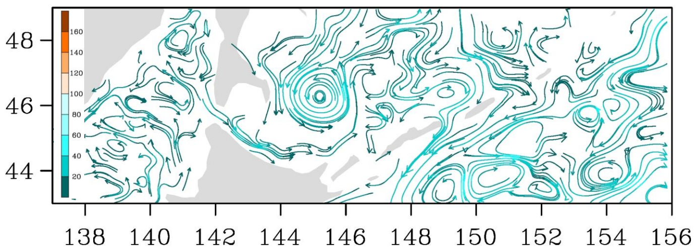
Рис. 3-9 Поверхностные течения, пролив Лаперуза, 25 февраля 2018 г.
