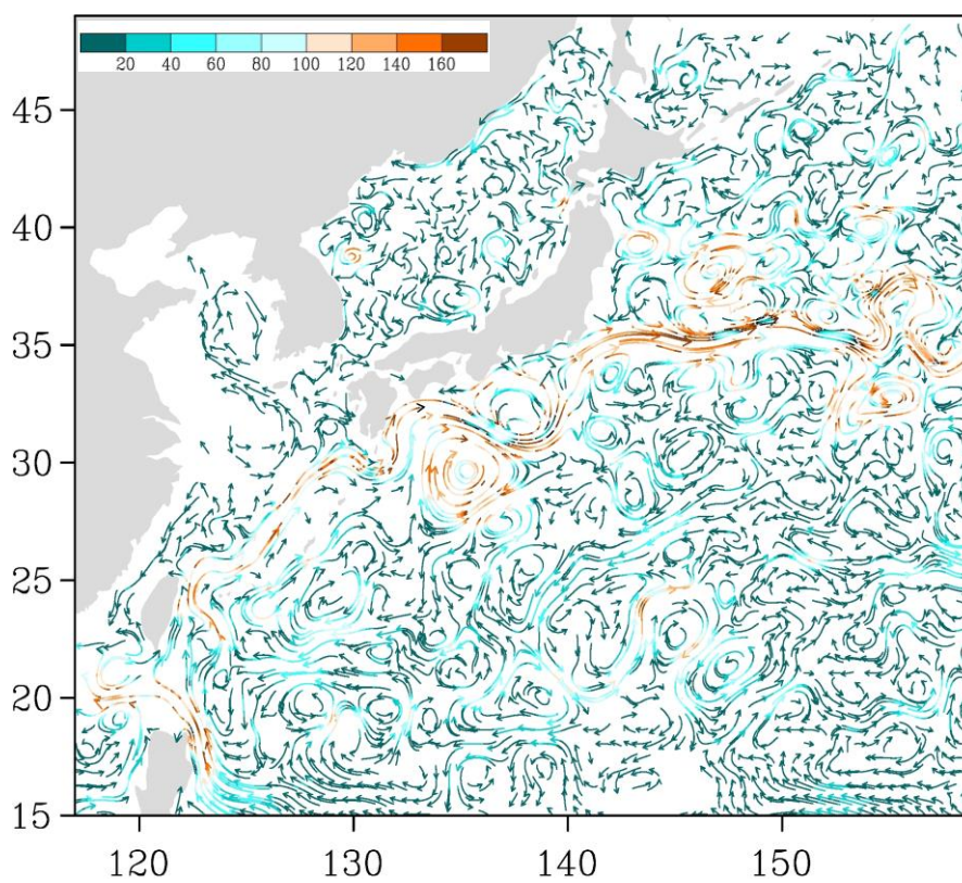
Рис. 3-4 Поверхностные течения западной части Тихого океана, 5 февраля 2018 г.
