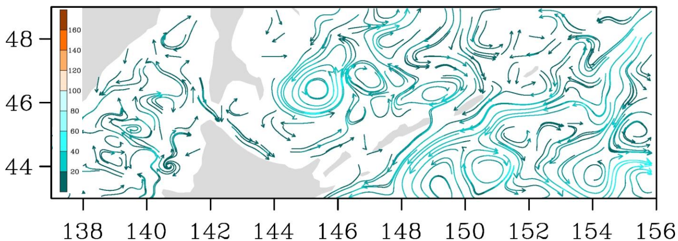
Рис. 3-8 Поверхностные течения, пролив Лаперуза, 15 февраля 2018 г.
