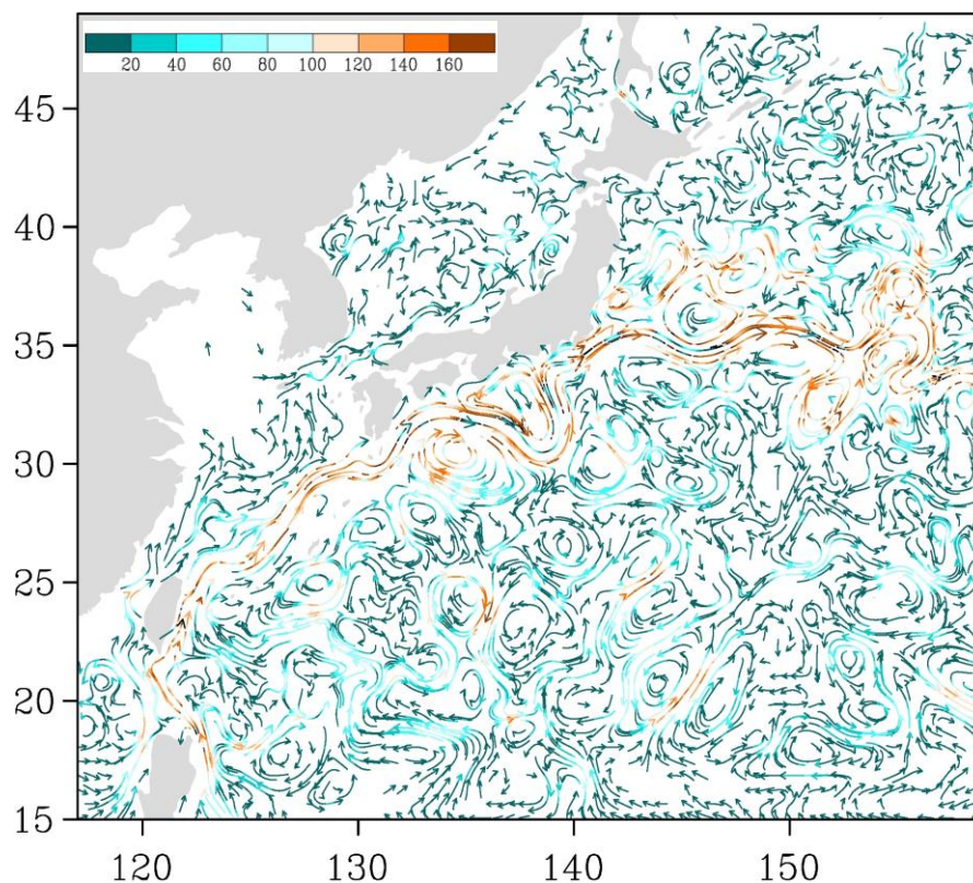
Рис. 3-6 Поверхностные течения западной части Тихого океана, 25 марта 2018 г.
