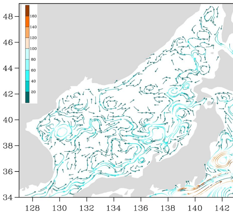
Рис. 3-3 Поверхностные течения Японского моря, 25 марта 2018 г.
