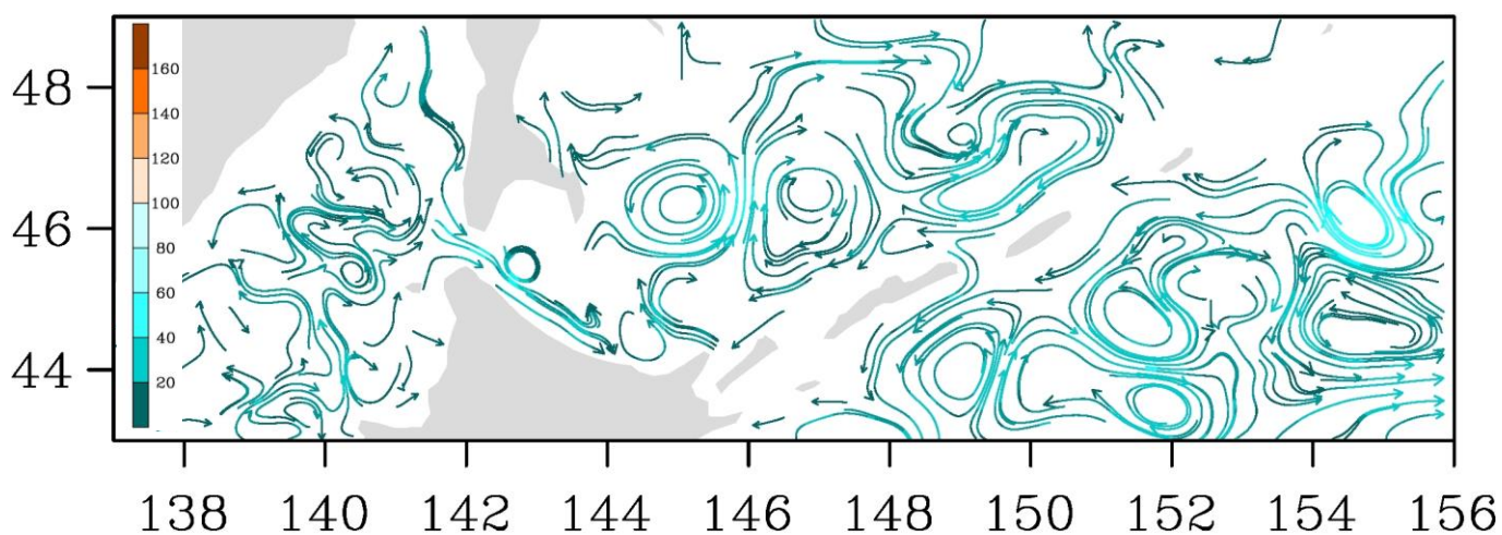
Рис. 3-9 Поверхностные течения, пролив Лаперуза, 25 марта 2018 г.
