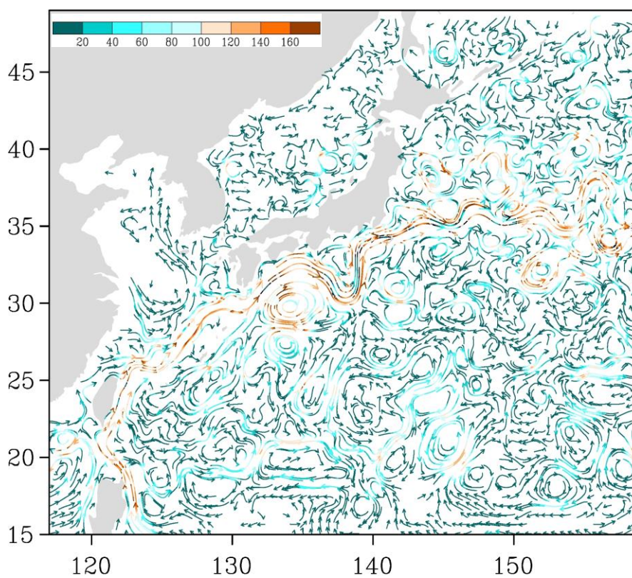
Рис. 3-4 Поверхностные течения западной части Тихого океана, 5 марта 2018 г.
