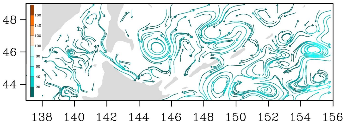
Рис. 3-8 Поверхностные течения, пролив Лаперуза, 15 марта 2018 г.
