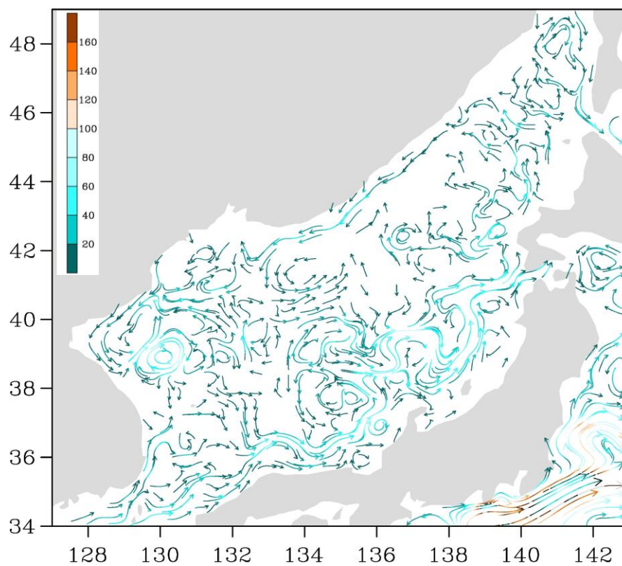
Рис. 3-2 Поверхностные течения Японского моря, 15 марта 2018 г.
