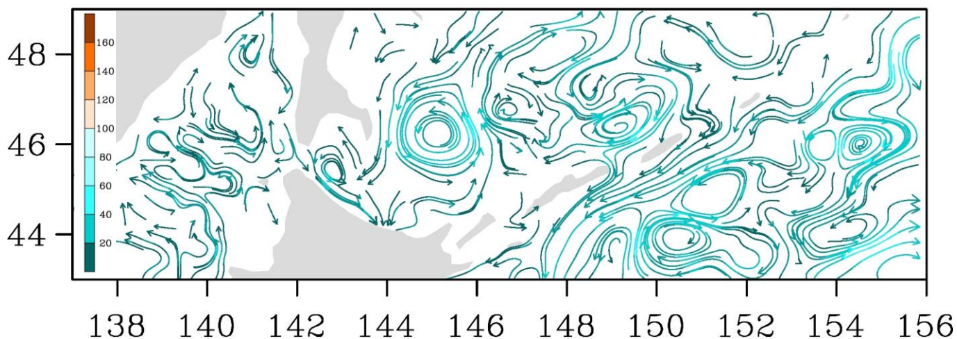
Рис. 3-7 Поверхностные течения, пролив Лаперуза, 5 марта 2018 г.
