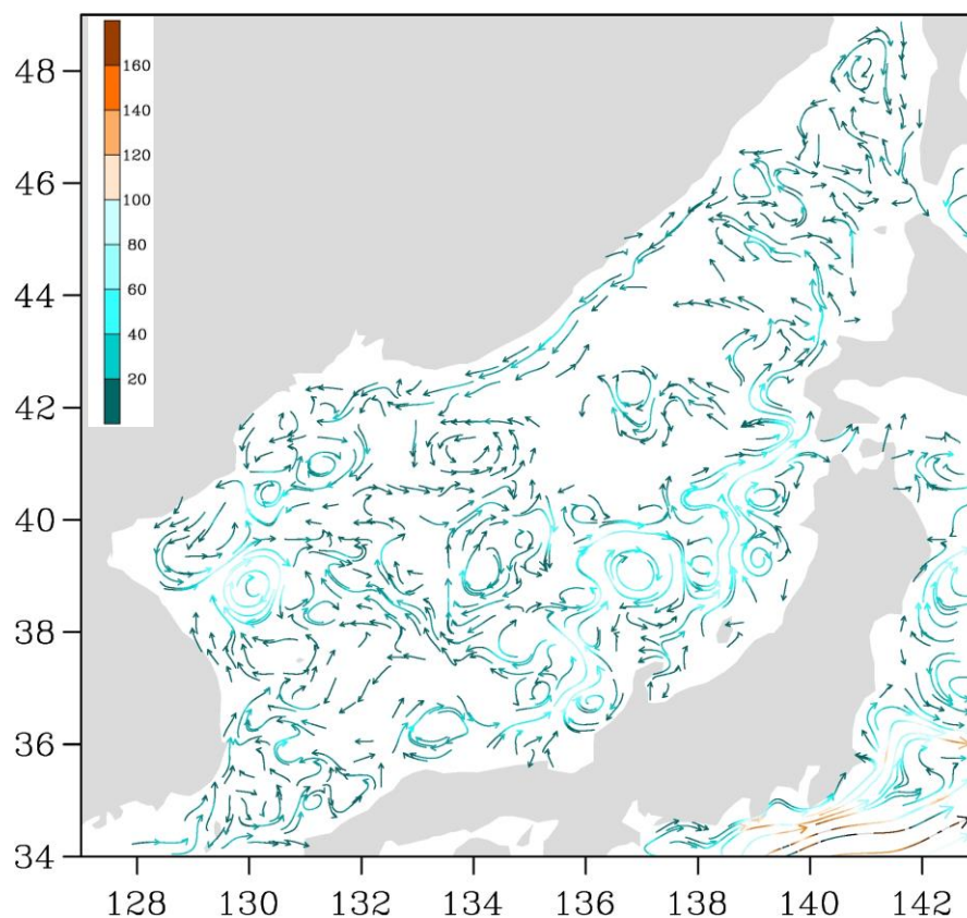
Рис. 3-1 Поверхностные течения Японского моря, 05 марта 2018 г.
