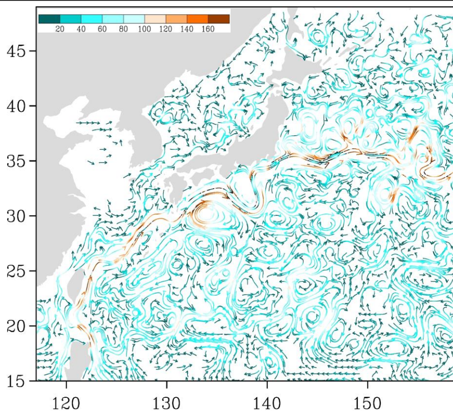
Рис. 3-5 Поверхностные течения западной части Тихого океана, 15 марта 2018 г.
