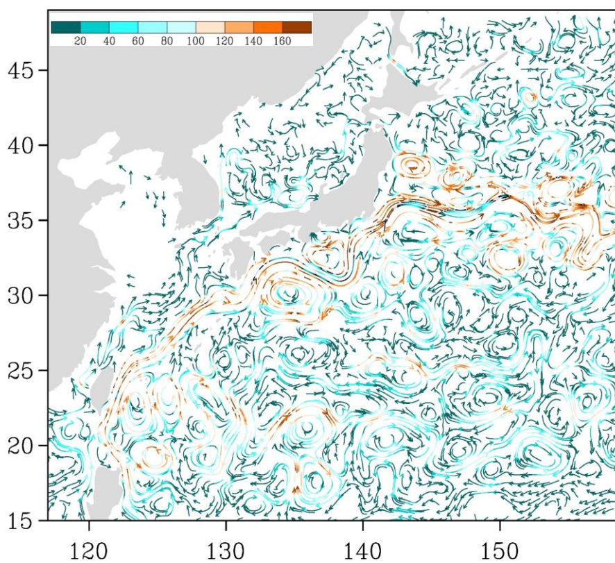
Рис. 3-4 Поверхностные течения западной части Тихого океана, 5 июня 2018 г.
