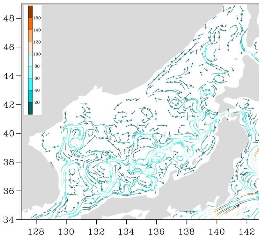
Рис. 3-3 Поверхностные течения Японского моря, 25 июня 2018 г.
