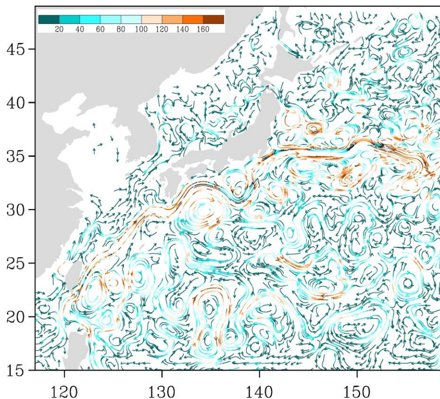
Рис. 3-6 Поверхностные течения западной части Тихого океана, 25 июня 2018 г.
