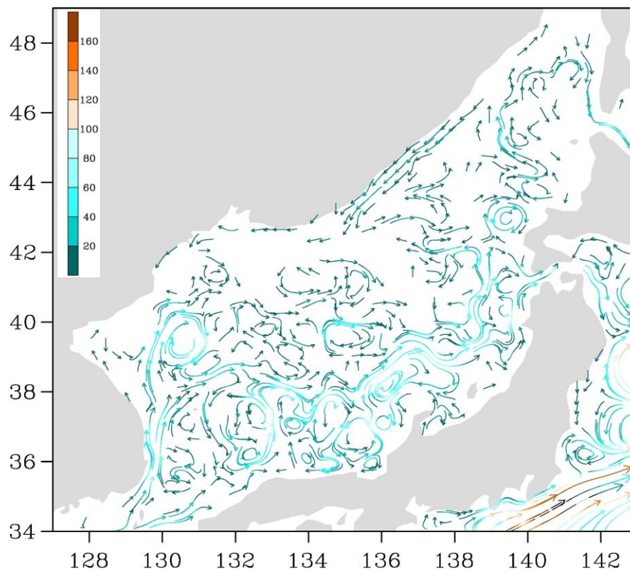
Рис. 3-2 Поверхностные течения Японского моря, 15 июня 2018 г.
