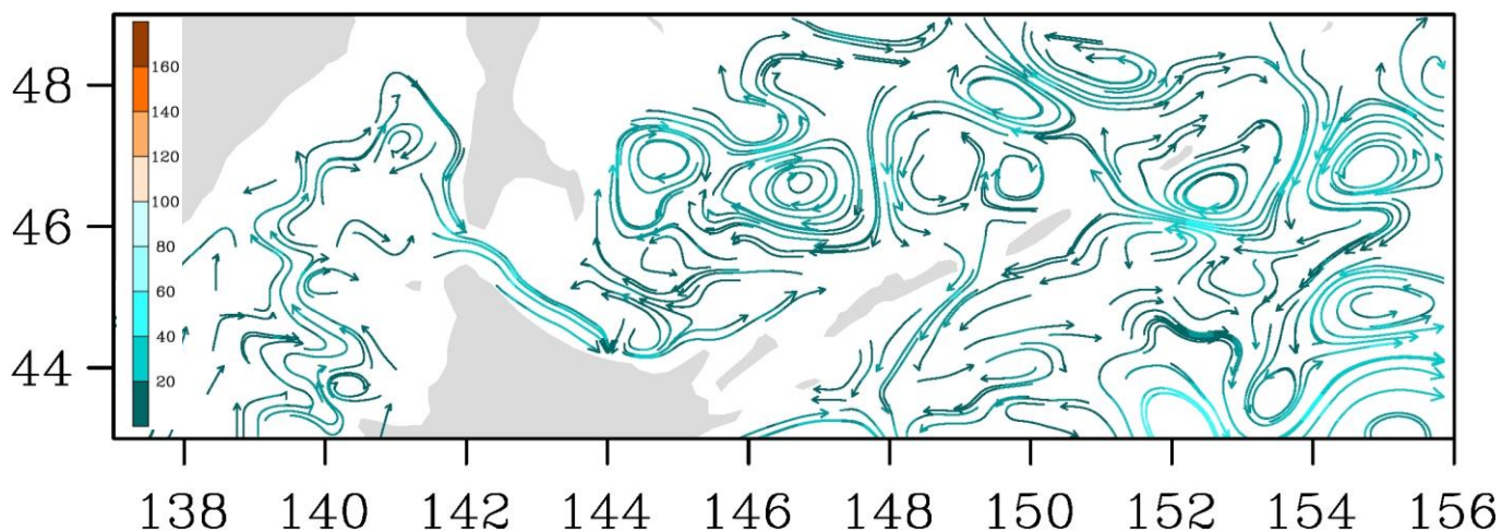
Рис. 3-7 Поверхностные течения, пролив Лаперуза, 5 июня 2018 г.
