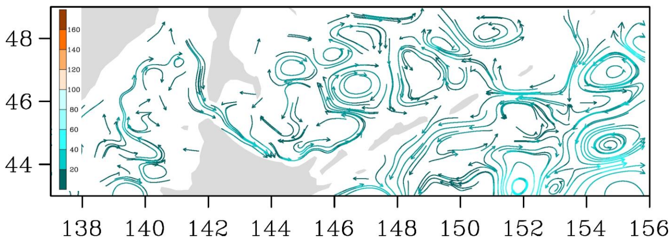
Рис. 3-8 Поверхностные течения, пролив Лаперуза, 15 июня 2018 г.
