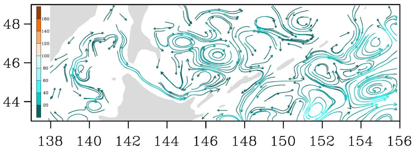
Рис. 3-9 Поверхностные течения, пролив Лаперуза, 25 июня 2018 г.
