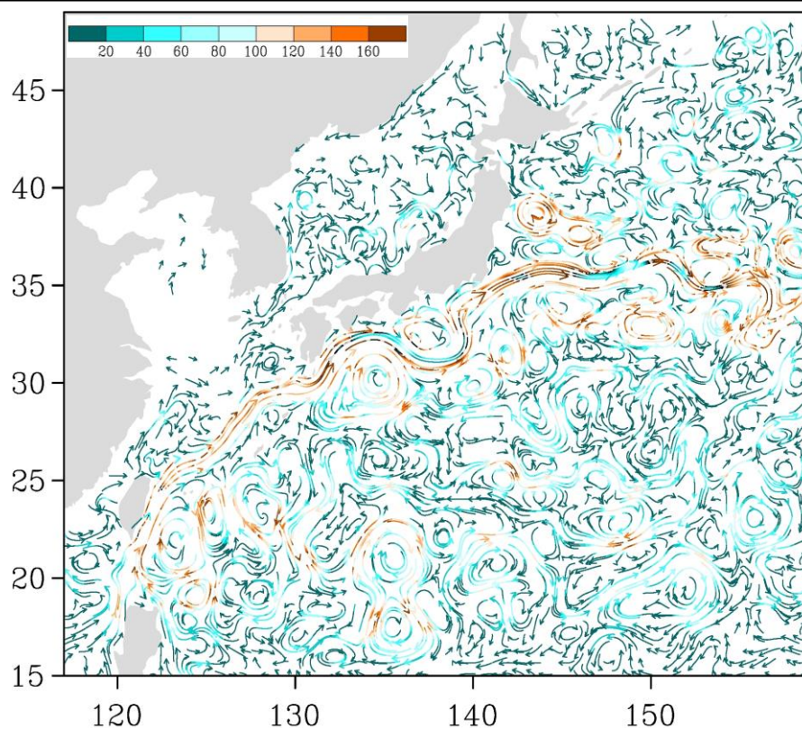
Рис. 3-5 Поверхностные течения западной части Тихого океана, 15 июня 2018 г.
