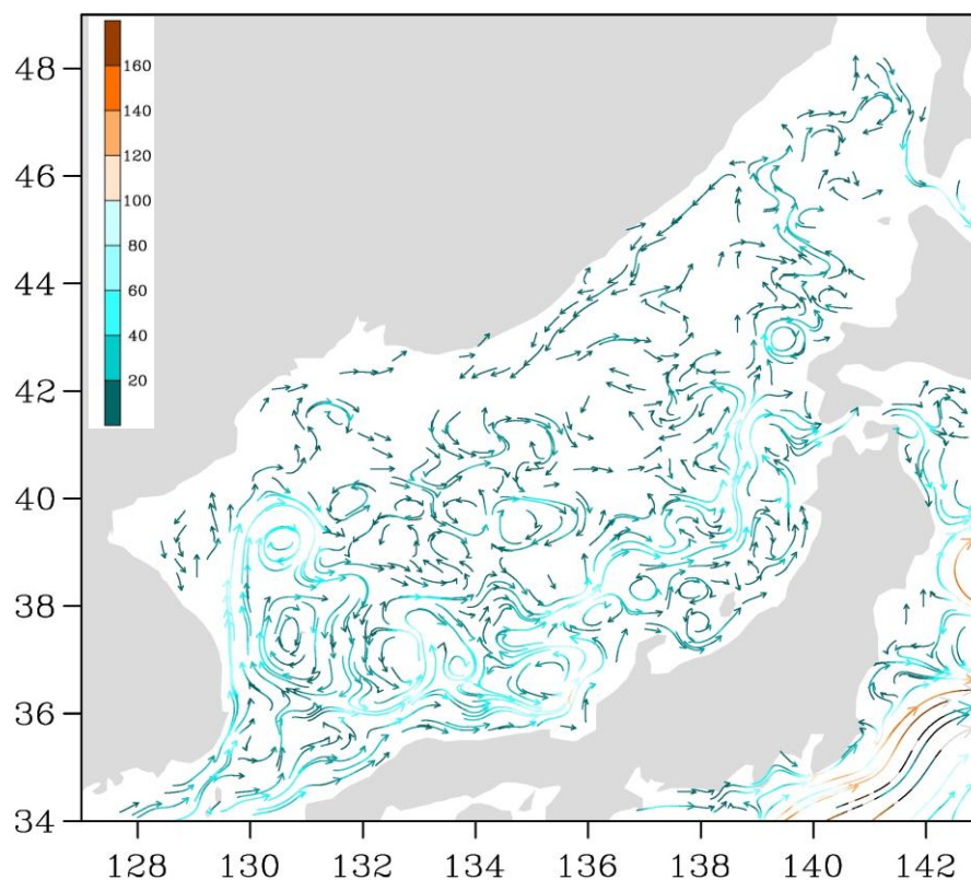
Рис. 3-1 Поверхностные течения Японского моря, 05 июня 2018 г.
