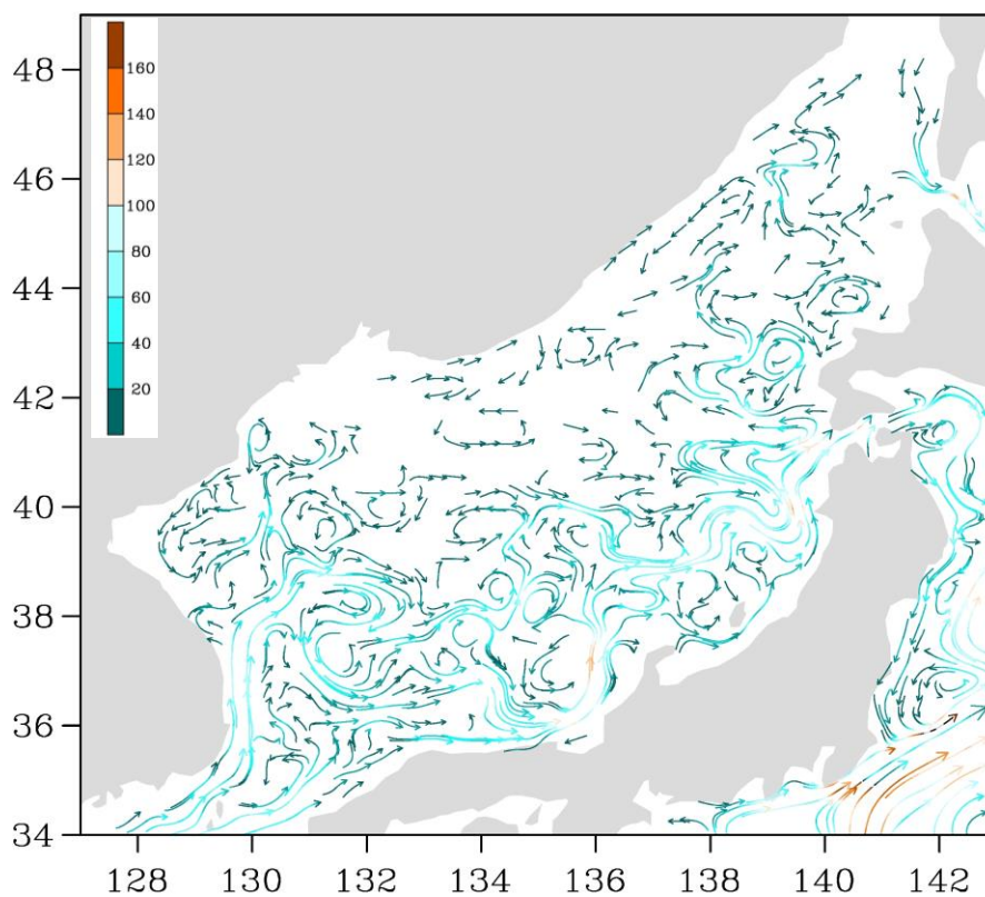
Рис. 3-3 Поверхностные течения Японского моря, 25 июля 2018 г.
