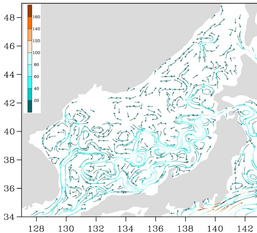
Рис. 3-2 Поверхностные течения Японского моря, 15 июля 2018 г.
