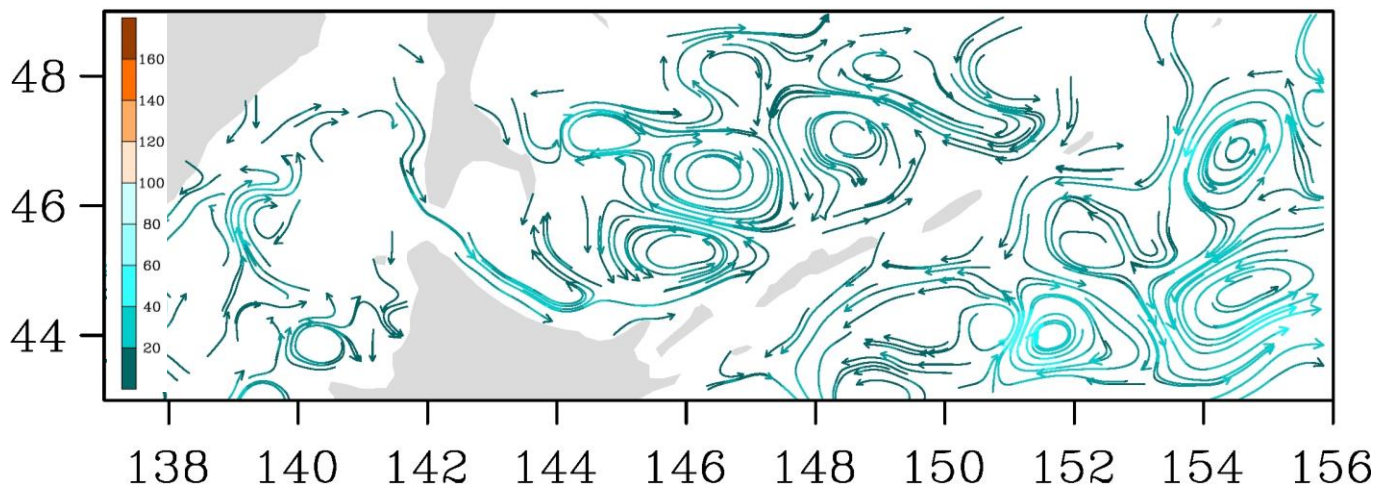
Рис. 3-7 Поверхностные течения, пролив Лаперуза, 5 июля 2018 г.
