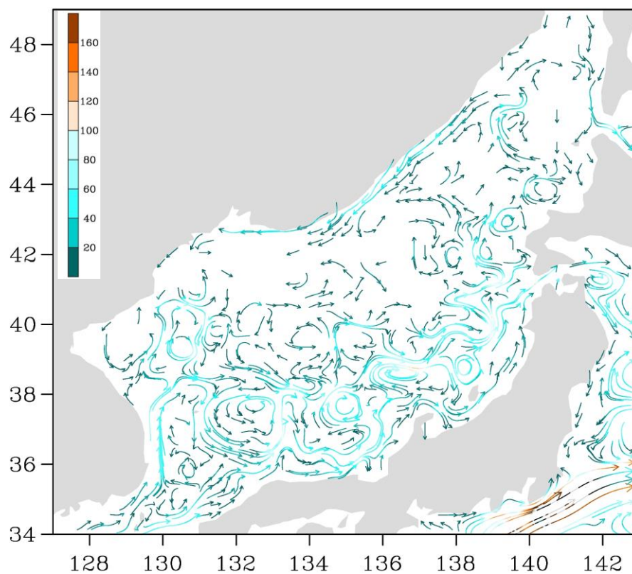
Рис. 3-1 Поверхностные течения Японского моря, 05 июля 2018 г.
