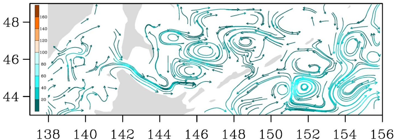
Рис. 3-8 Поверхностные течения, пролив Лаперуза, 15 июля 2018 г.
