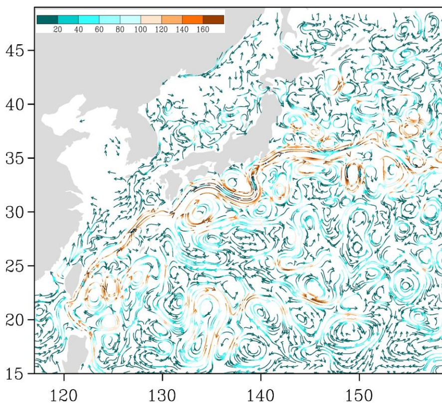
Рис. 3-4 Поверхностные течения западной части Тихого океана, 5 июля 2018 г.
