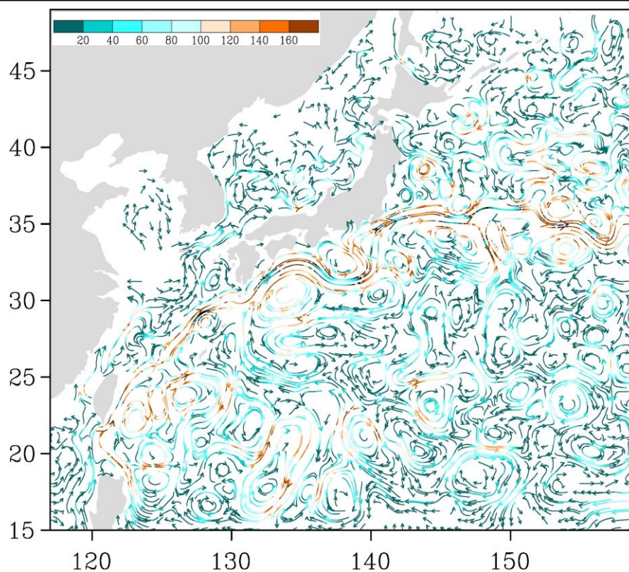
Рис. 3-5 Поверхностные течения западной части Тихого океана, 15 июля 2018 г.
