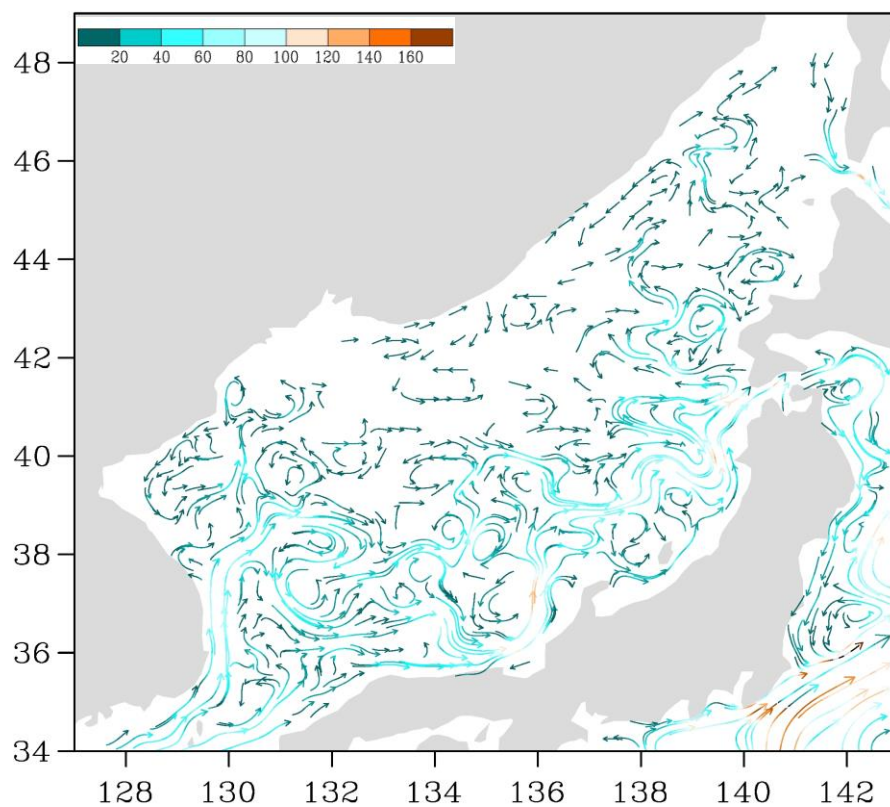
Рис. 3-6 Поверхностные течения западной части Тихого океана, 25 июля 2018 г.
