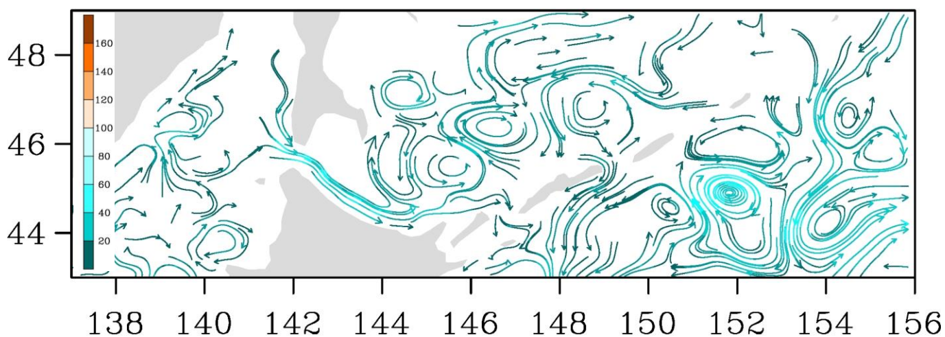
Рис. 3-9 Поверхностные течения, пролив Лаперуза, 25 июля 2018 г.
