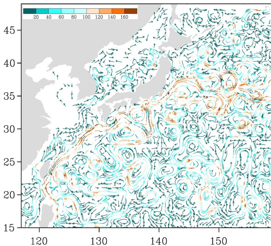
Рис. 3-5 Поверхностные течения западной части Тихого океана, 15 мая 2019 г.
