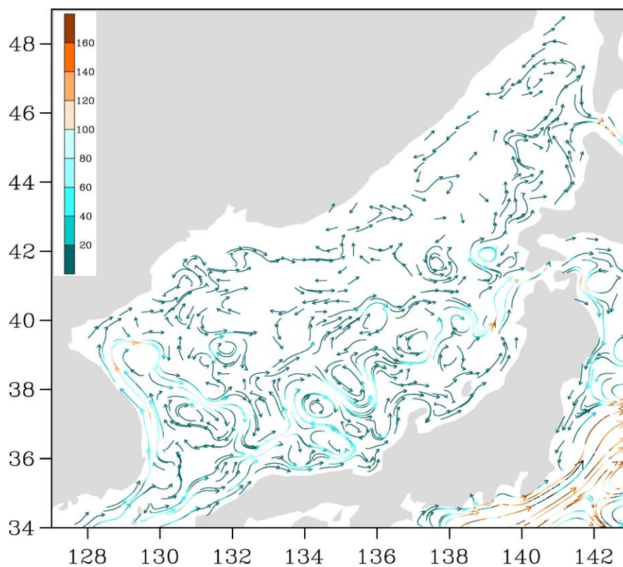
Рис. 3-3 Поверхностные течения Японского моря, 25 мая 2019 г.
