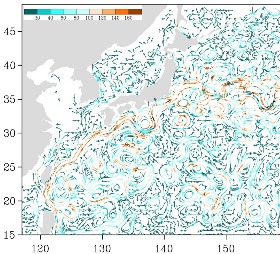
Рис. 3-6 Поверхностные течения западной части Тихого океана, 25 мая 2019 г.
