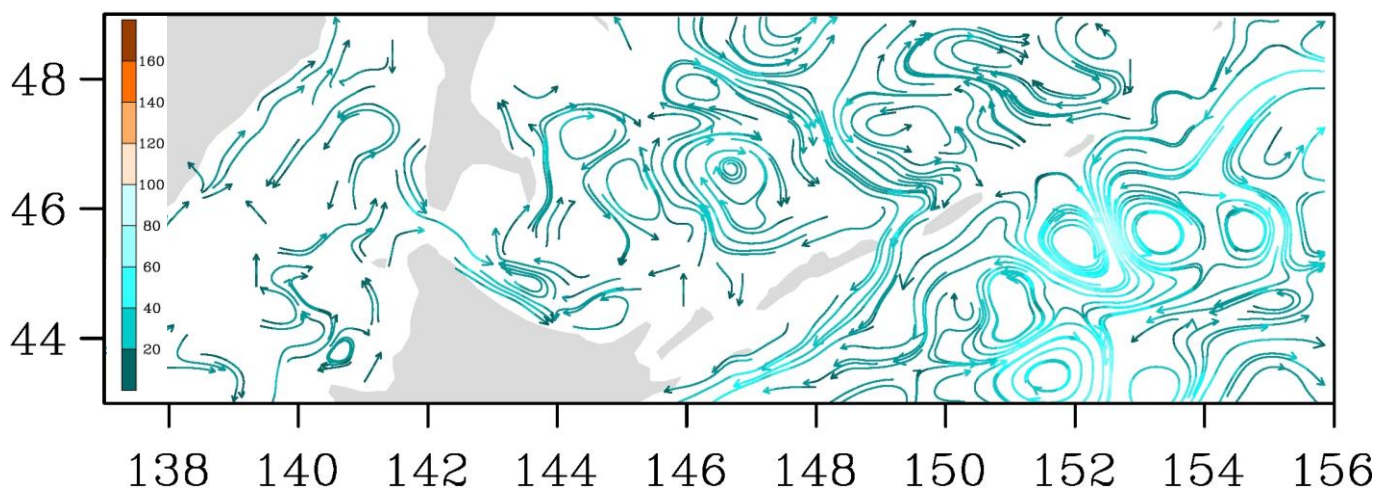
Рис. 3-8 Поверхностные течения, пролив Лаперуза, 15 мая 2019 г.
