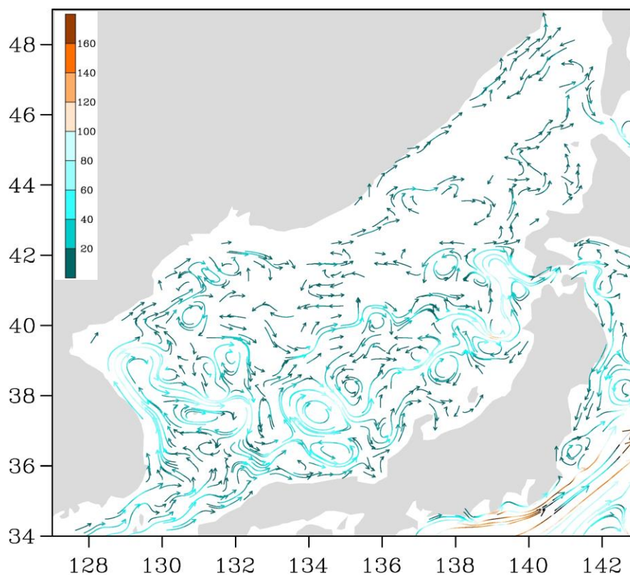
Рис. 3-2 Поверхностные течения Японского моря, 15 мая 2019 г.
