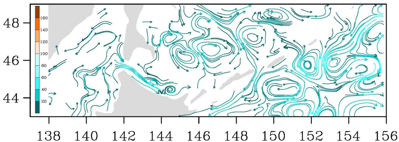
Рис. 3-9 Поверхностные течения, пролив Лаперуза, 25 мая 2019 г.
