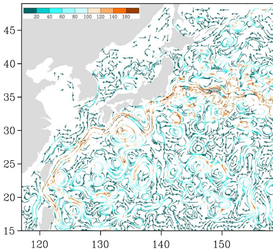
Рис. 3-4 Поверхностные течения западной части Тихого океана, 5 мая 2019 г.
