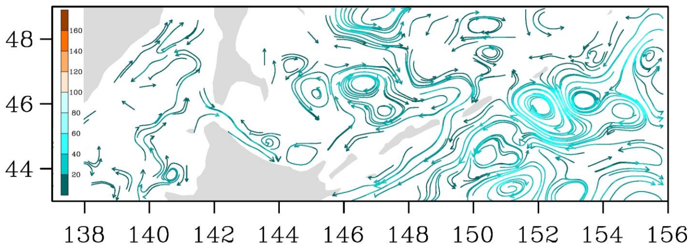
Рис. 3-7 Поверхностные течения, пролив Лаперуза, 5 мая 2019 г.
