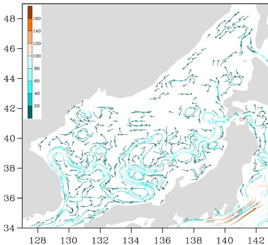
Рис. 3-1 Поверхностные течения Японского моря, 05 мая 2019 г.
