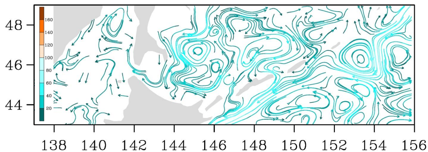
Рис. 3-9 Поверхностные течения, пролив Лаперуза, 25 января 2019 г.
