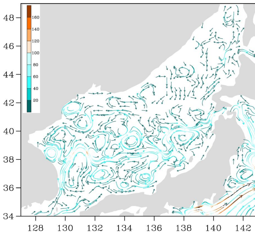
Рис. 3-2 Поверхностные течения Японского моря, 15 января 2019 г.
