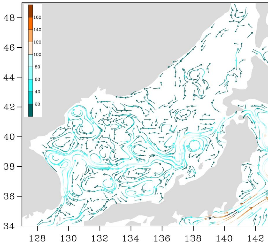
Рис. 3-1 Поверхностные течения Японского моря, 05 января 2019 г.
