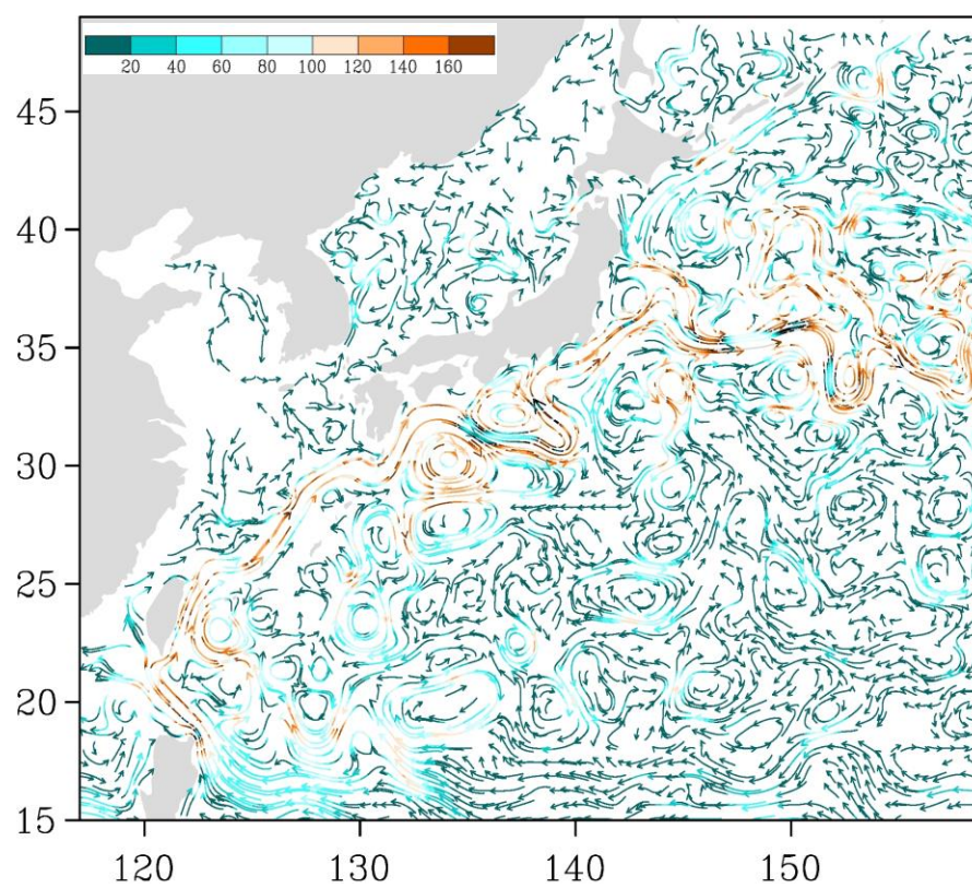
Рис. 3-6 Поверхностные течения западной части Тихого океана, 25 января 2019 г.
