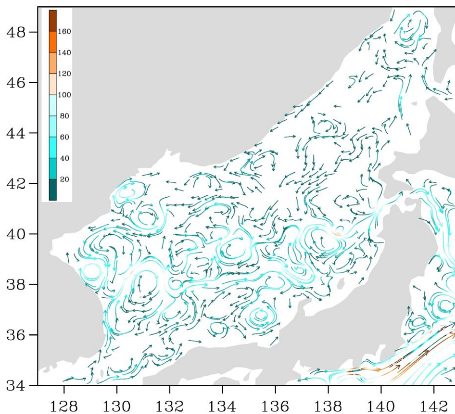
Рис. 3-3 Поверхностные течения Японского моря, 25 января 2019 г.
