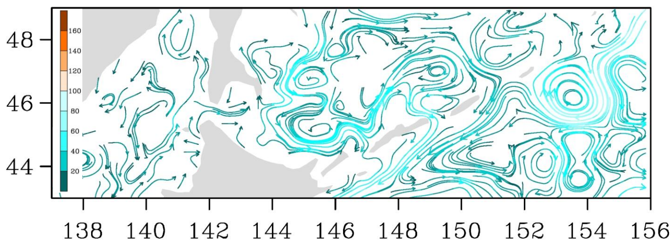
Рис. 3-8 Поверхностные течения, пролив Лаперуза, 15 января 2019 г.
