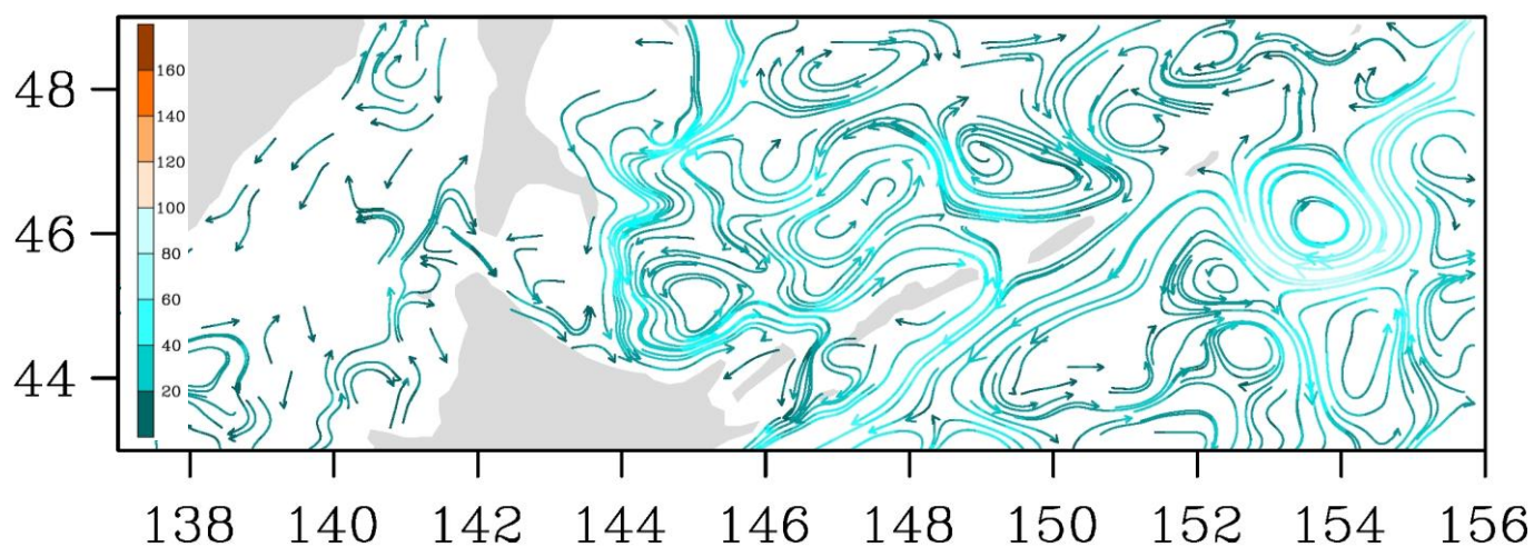
Рис. 3-7 Поверхностные течения, пролив Лаперуза, 5 января 2019 г.
