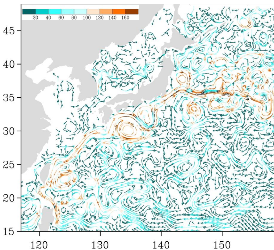
Рис. 3-4 Поверхностные течения западной части Тихого океана, 5 января 2019 г.
