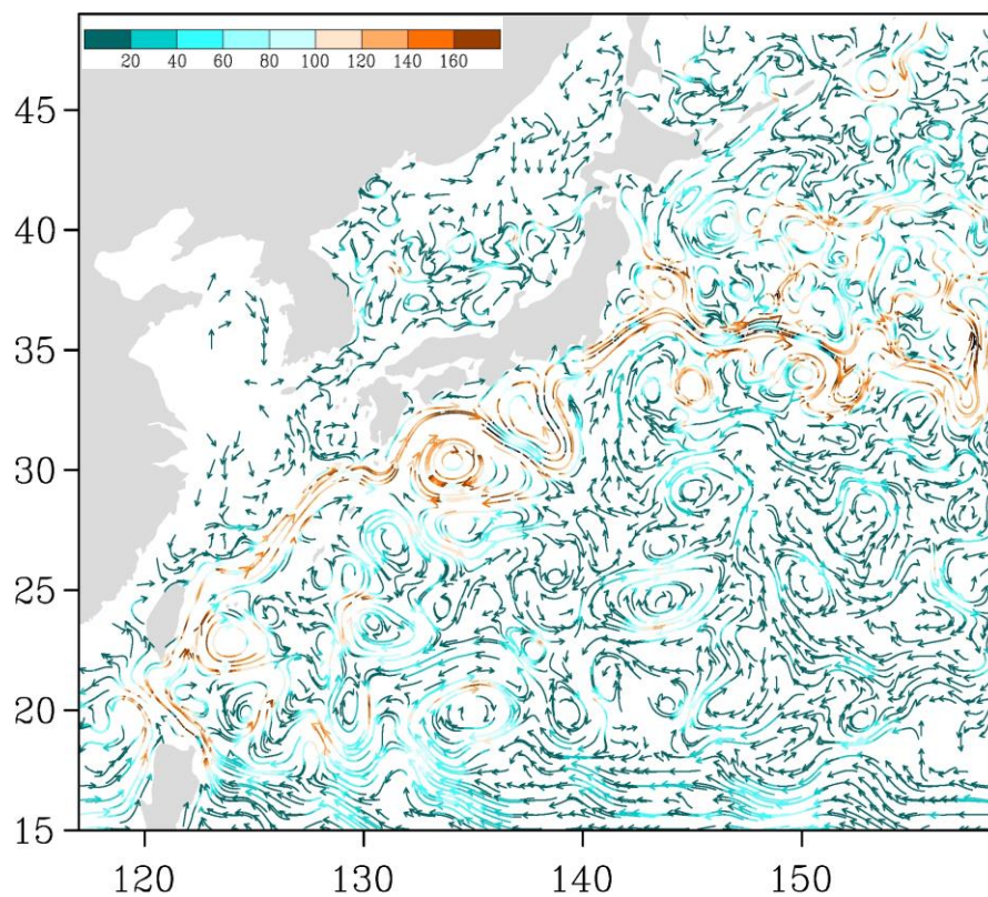
Рис. 3-5 Поверхностные течения западной части Тихого океана, 15 января 2019 г.
