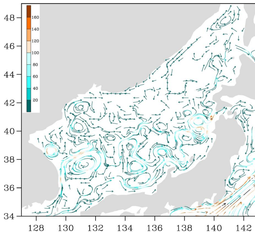
Рис. 3-2 Поверхностные течения Японского моря, 15 марта 2019 г.
