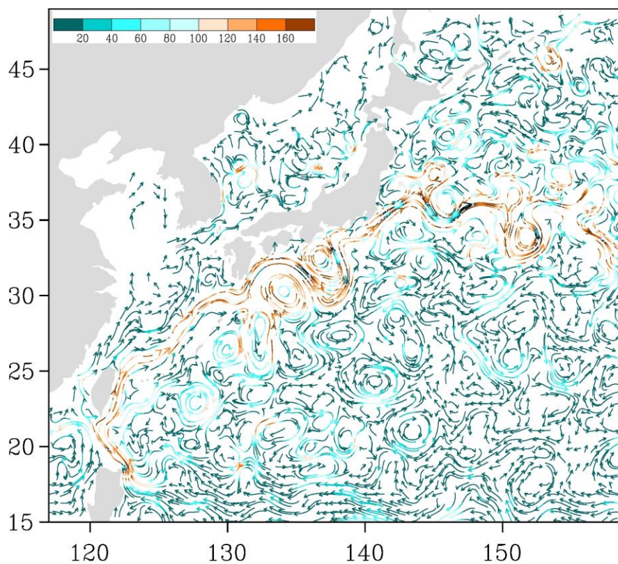
Рис. 3-4 Поверхностные течения западной части Тихого океана, 5 марта 2019 г.
