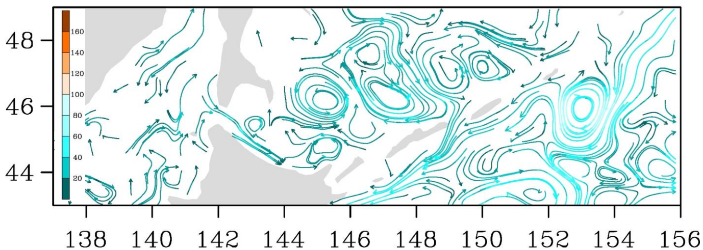
Рис. 3-9 Поверхностные течения, пролив Лаперуза, 25 марта 2019 г.
