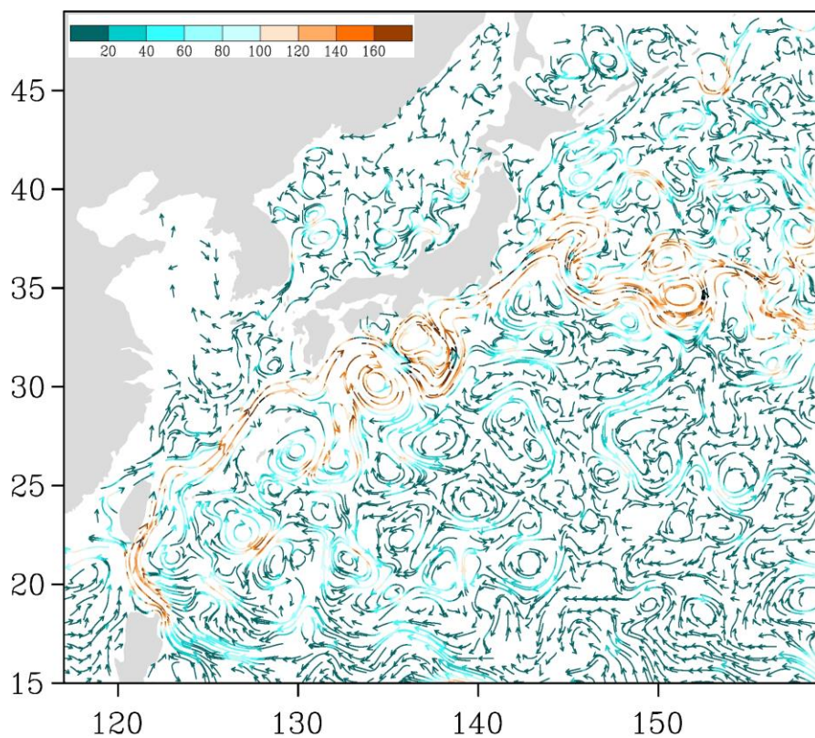
Рис. 3-5 Поверхностные течения западной части Тихого океана, 15 марта 2019 г.
