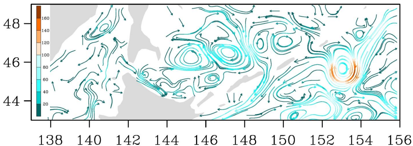
Рис. 3-8 Поверхностные течения, пролив Лаперуза, 15 марта 2019 г.
