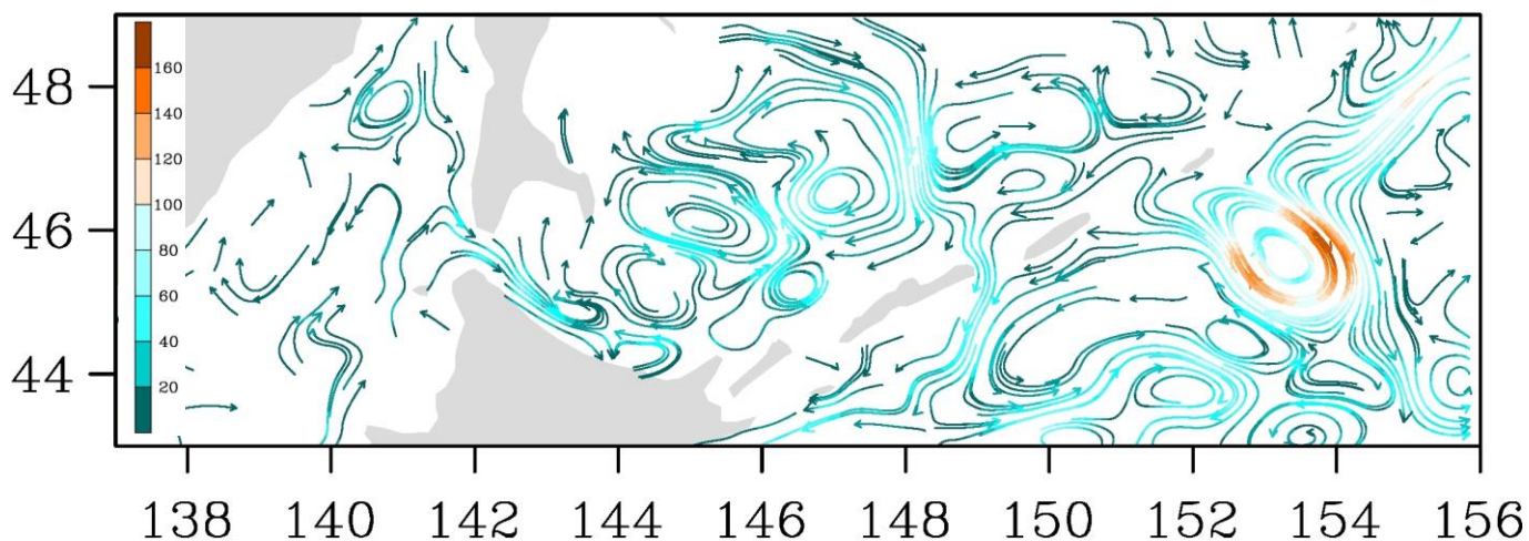
Рис. 3-7 Поверхностные течения, пролив Лаперуза, 5 марта 2019 г.
