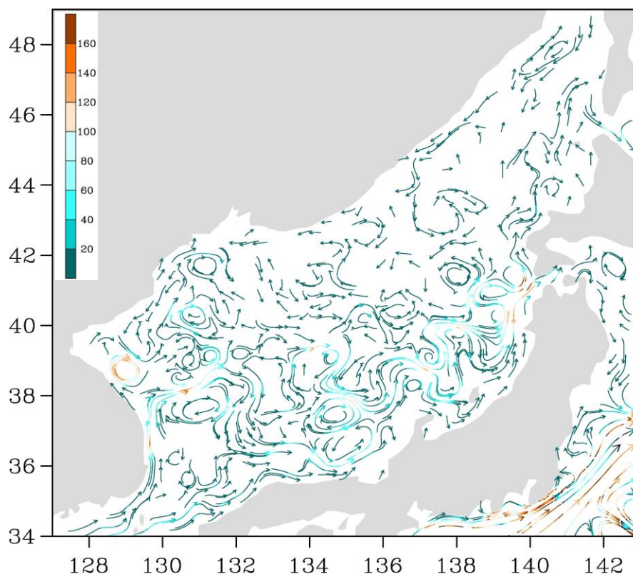
Рис. 3-3 Поверхностные течения Японского моря, 25 марта 2019 г.
