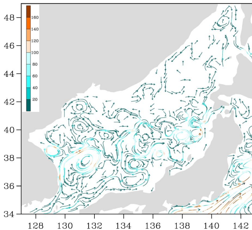
Рис. 3-1 Поверхностные течения Японского моря, 05 марта 2019 г.
