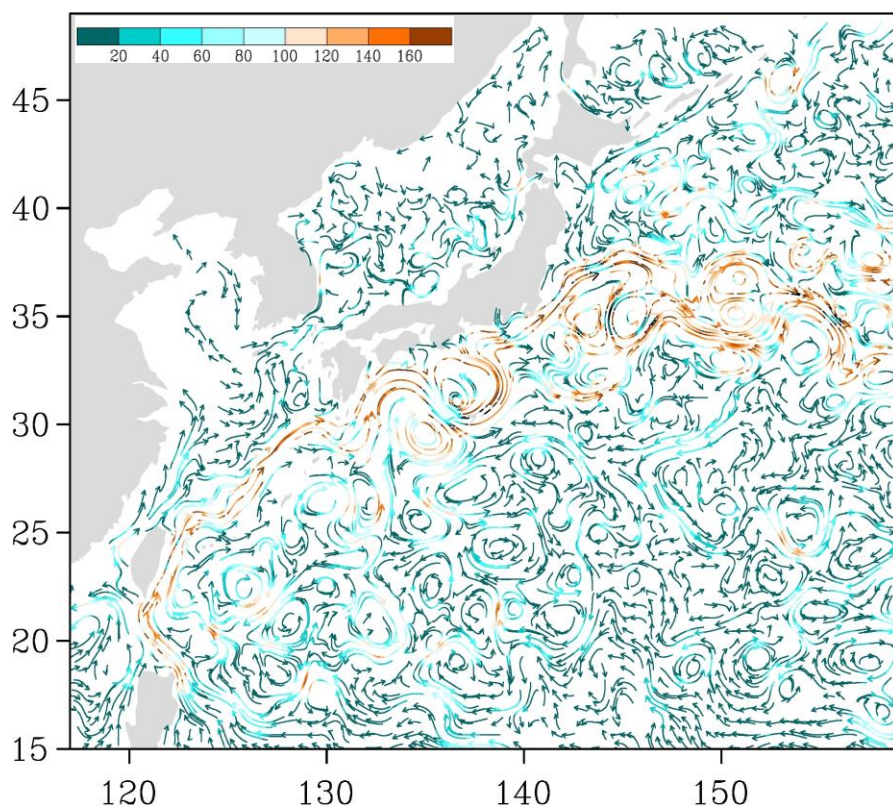
Рис. 3-6 Поверхностные течения западной части Тихого океана, 25 марта 2019 г.
