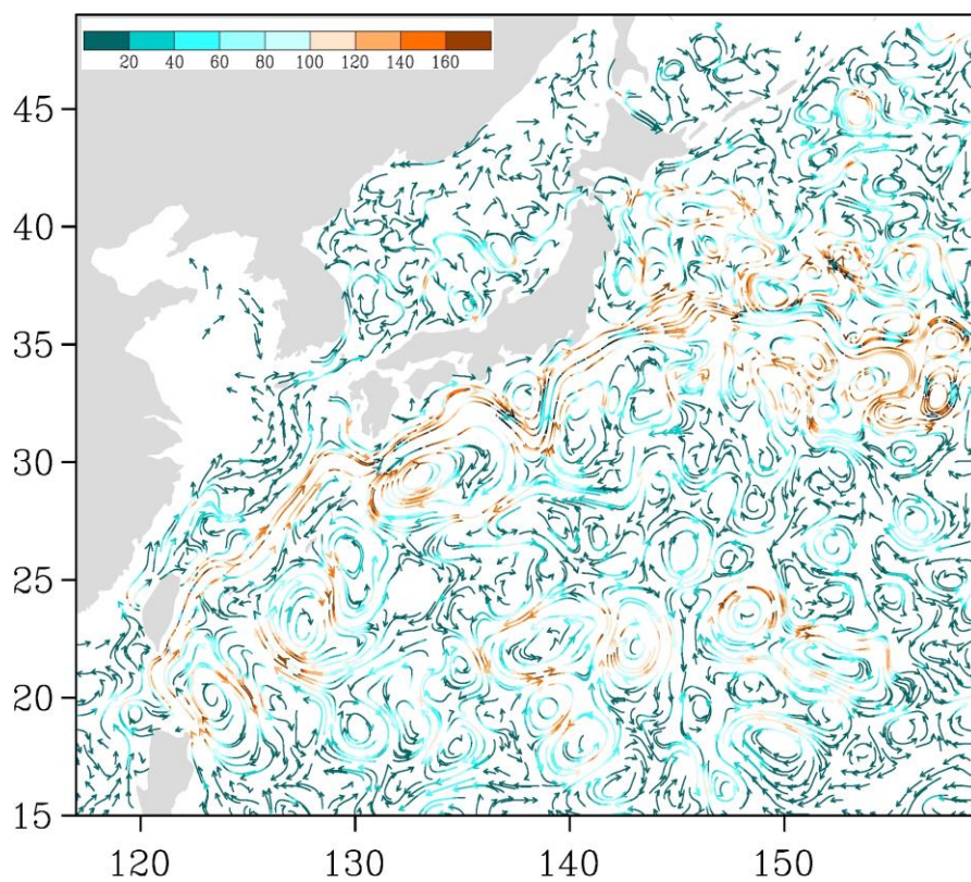
Рис. 3-6 Поверхностные течения западной части Тихого океана, 25 августа 2019 г.
