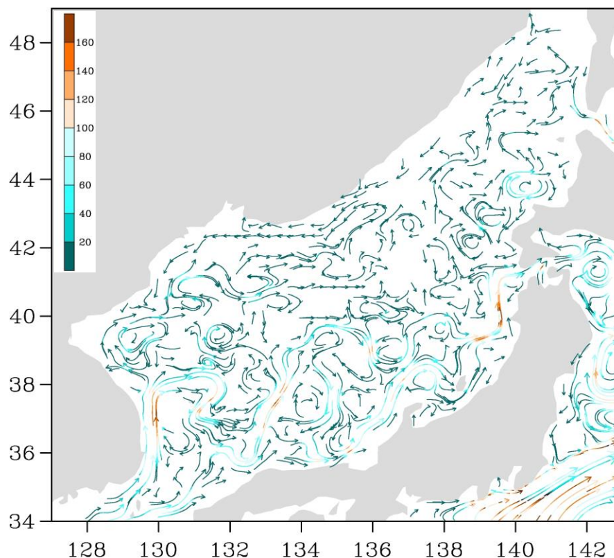
Рис. 3-1 Поверхностные течения Японского моря, 05 августа 2019 г.
