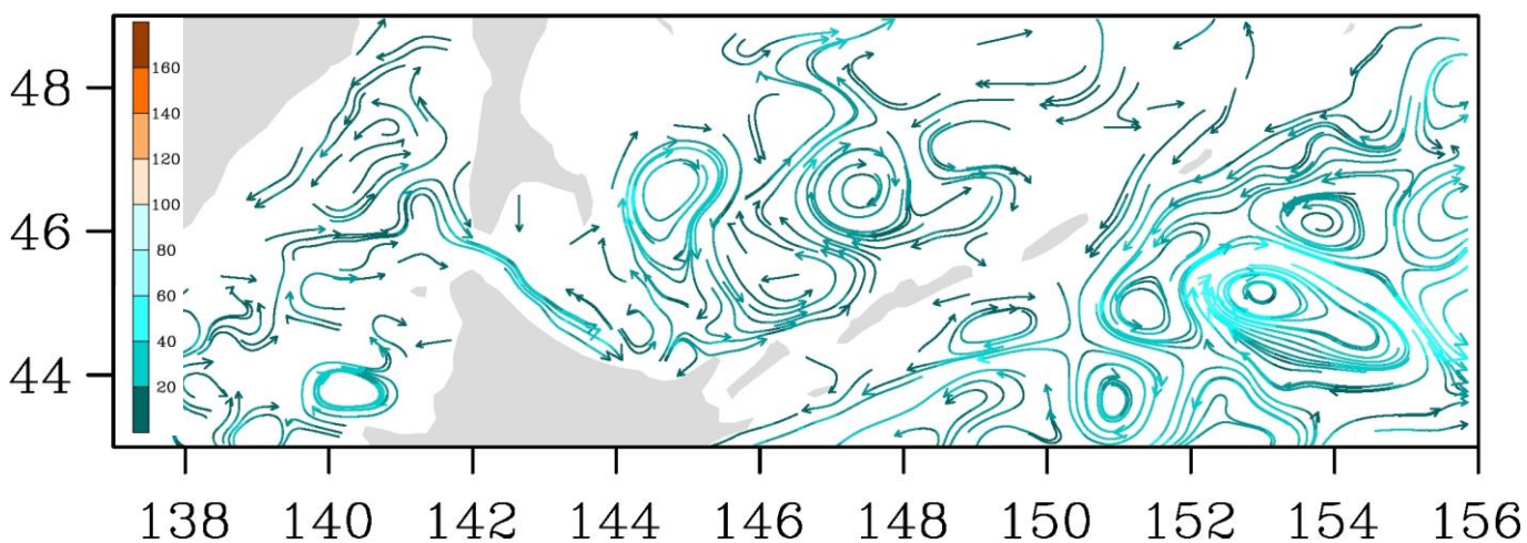
Рис. 3-8 Поверхностные течения, пролив Лаперуза, 15 августа 2019 г.
