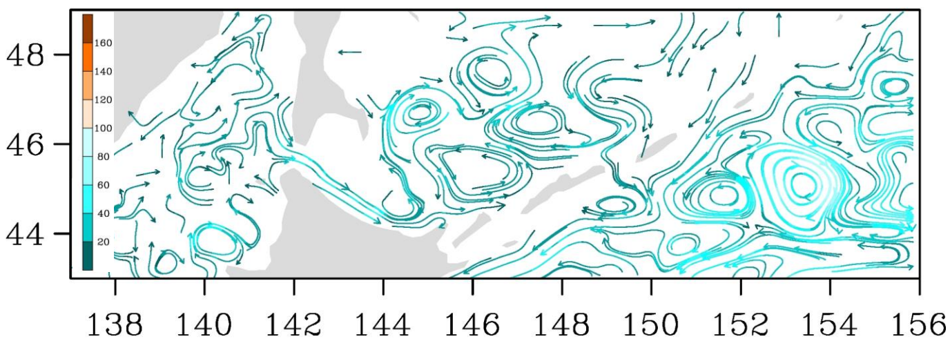
Рис. 3-9 Поверхностные течения, пролив Лаперуза, 25 августа 2019 г.
