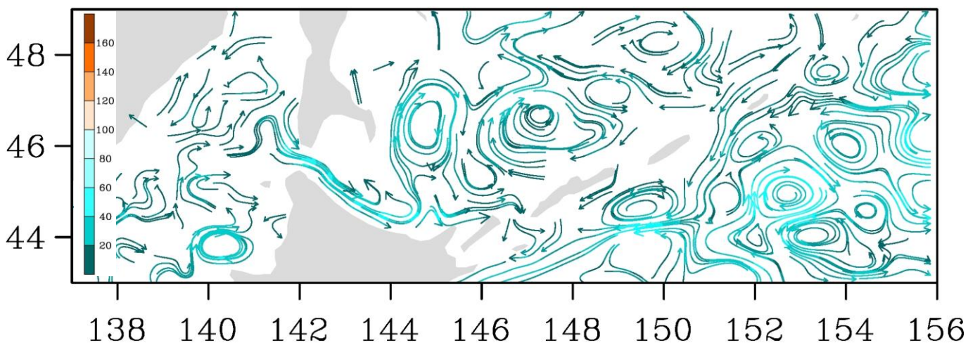
Рис. 3-7 Поверхностные течения, пролив Лаперуза, 5 августа 2019 г.
