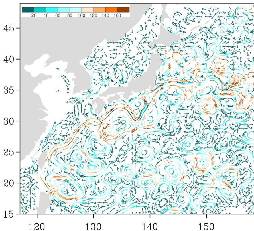
Рис. 3-4 Поверхностные течения западной части Тихого океана, 5 августа 2019 г.
