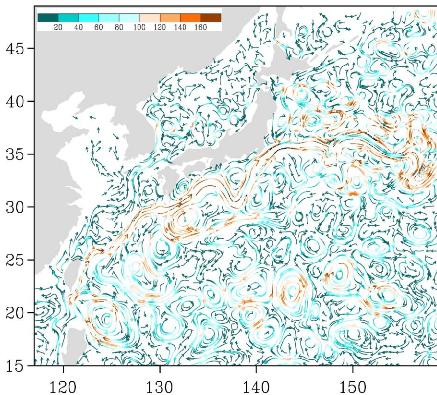
Рис. 3-5 Поверхностные течения западной части Тихого океана, 15 августа 2019 г.
