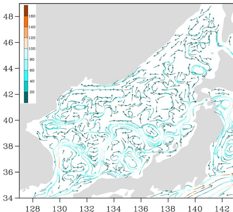
Рис. 3-3 Поверхностные течения Японского моря, 25 августа 2019 г.
