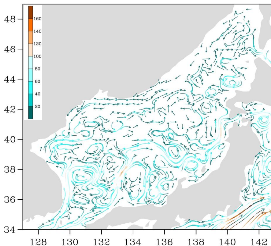
Рис. 3-2 Поверхностные течения Японского моря, 15 августа 2019 г.
