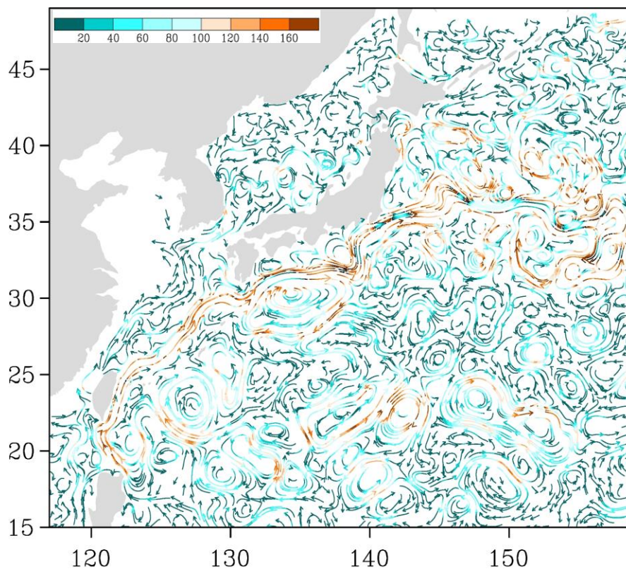
Рис. 3-4 Поверхностные течения западной части Тихого океана, 5 сентября 2019 г.
