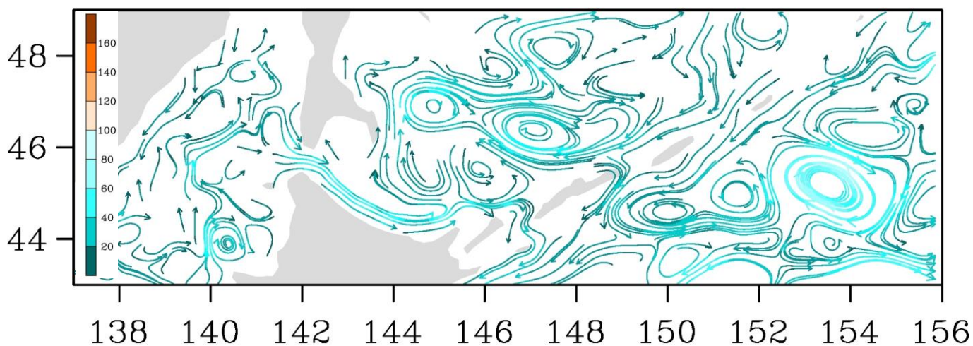
Рис. 3-8 Поверхностные течения, пролив Лаперуза, 15 сентября 2019 г.
