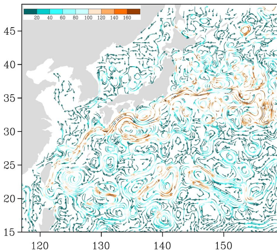
Рис. 3-6 Поверхностные течения западной части Тихого океана, 25 сентября 2019 г.
