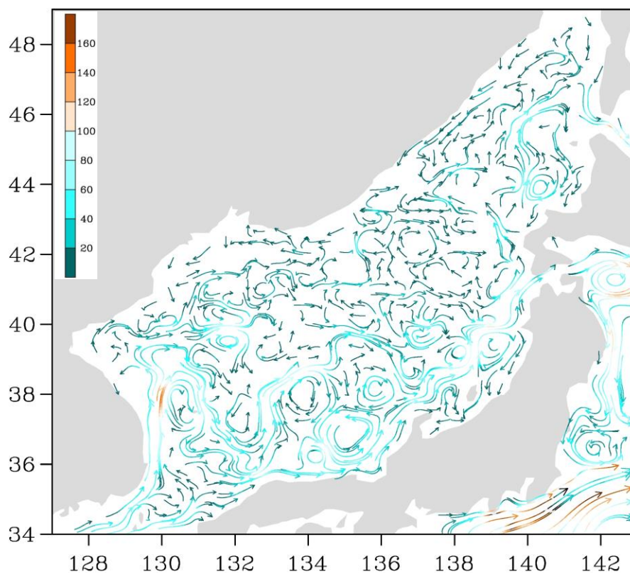
Рис. 3-3 Поверхностные течения Японского моря, 25 сентября 2019 г.
