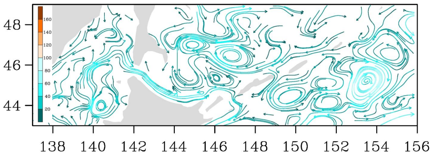
Рис. 3-9 Поверхностные течения, пролив Лаперуза, 25 сентября 2019 г.
