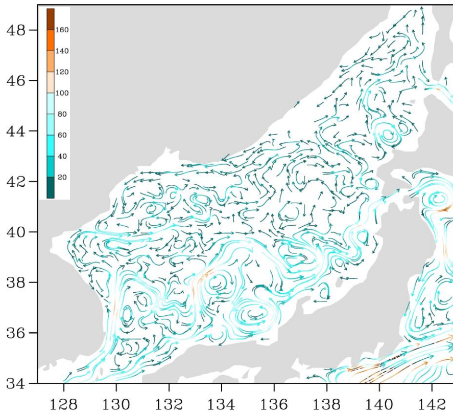
Рис. 3-1 Поверхностные течения Японского моря, 05 сентября 2019 г.
