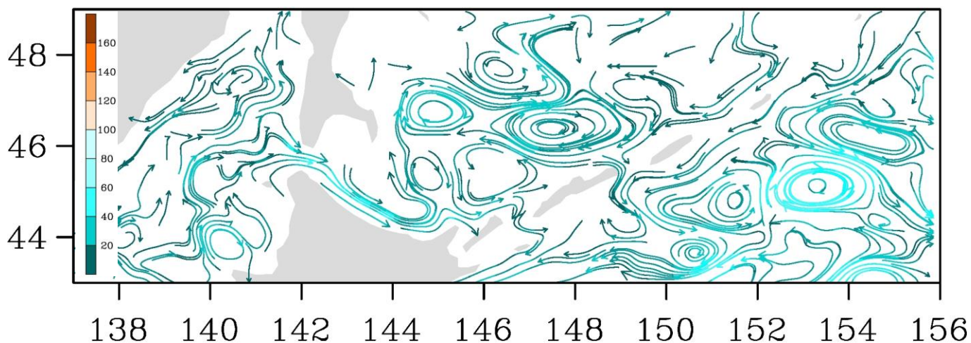
Рис. 3-7 Поверхностные течения, пролив Лаперуза, 5 сентября 2019 г.
