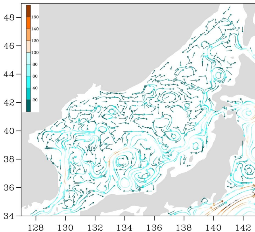
Рис. 3-2 Поверхностные течения Японского моря, 15 сентября 2019 г.
