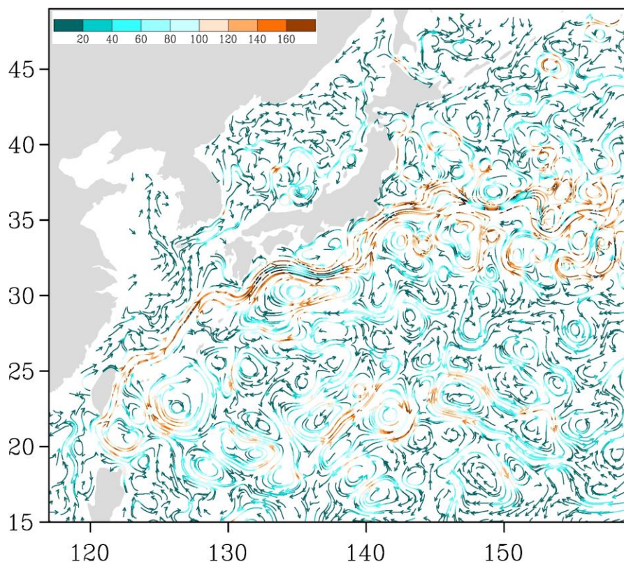
Рис. 3-5 Поверхностные течения западной части Тихого океана, 15 сентября 2019 г.
