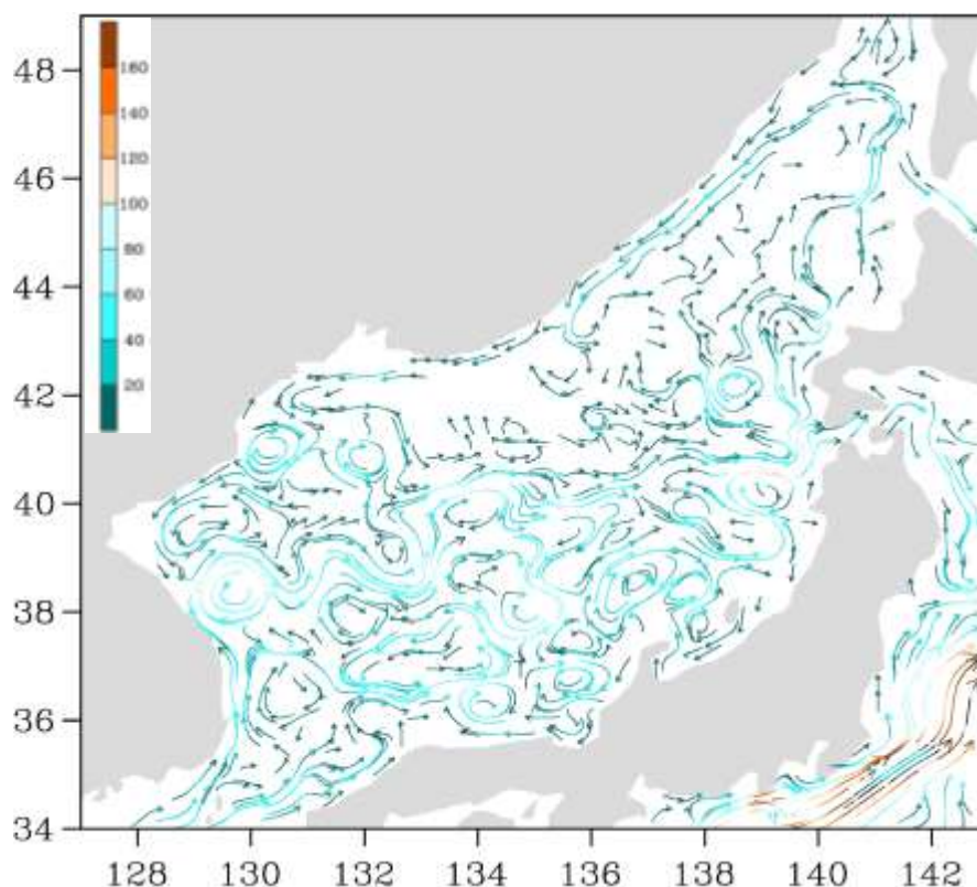
Рис. 3-3 Поверхностные течения Японского моря, 25 января 2021 г.
