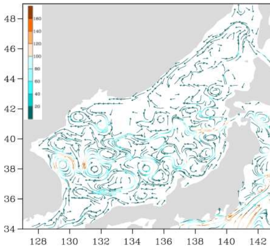
Рис. 3-1 Поверхностные течения Японского моря, 05 января 2021 г.
