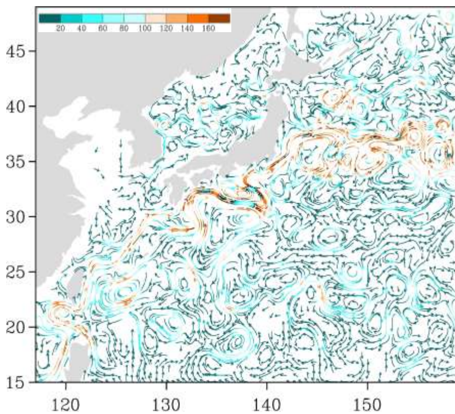
Рис. 3-6 Поверхностные течения западной части Тихого океана, 25 января 2021 г.
