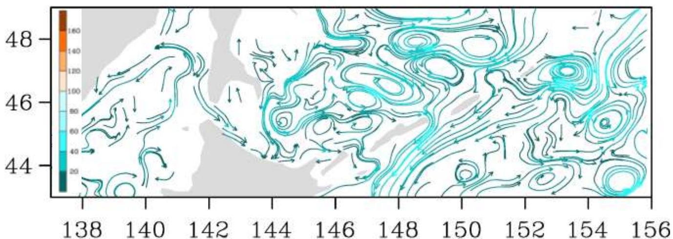
Рис. 3-7 Поверхностные течения, пролив Лаперуза, 5 января 2021 г.
