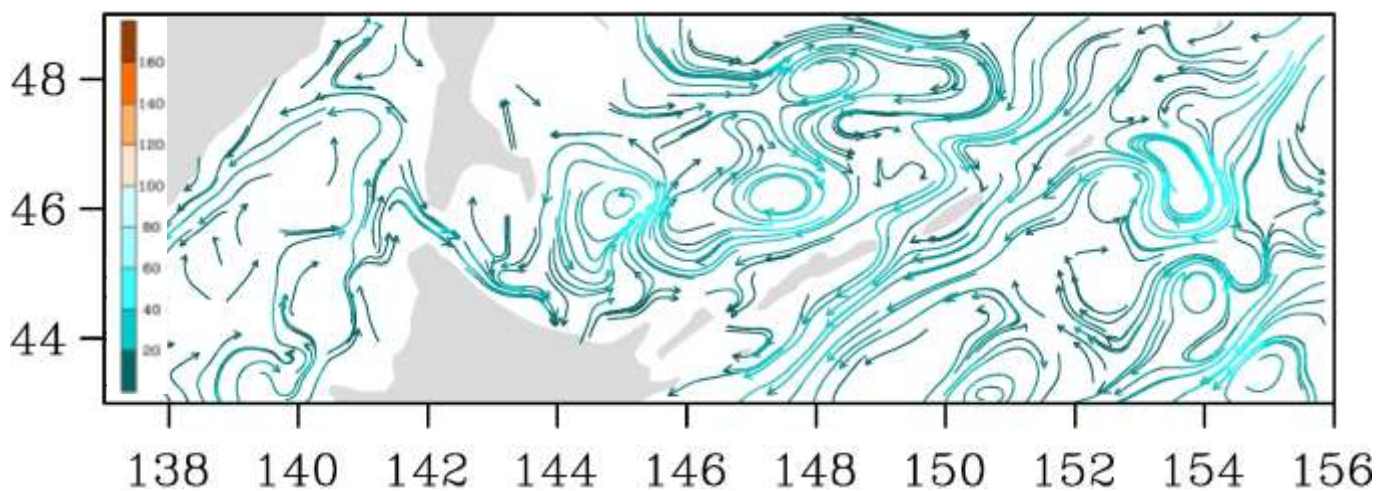
Рис. 3-9 Поверхностные течения, пролив Лаперуза, 25 января 2021 г.
