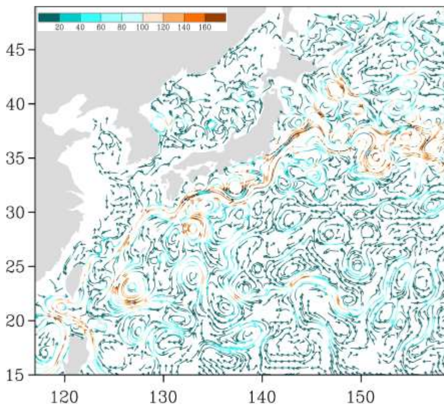
Рис. 3-4 Поверхностные течения западной части Тихого океана, 5 января 2021 г.
