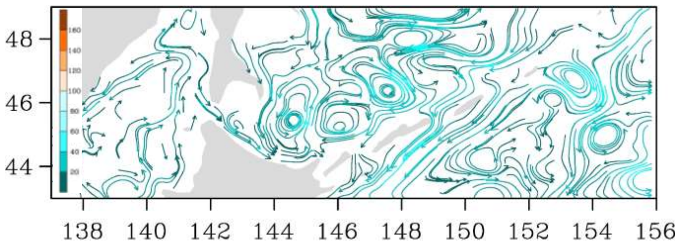
Рис. 3-8 Поверхностные течения, пролив Лаперуза, 15 января 2021 г.
