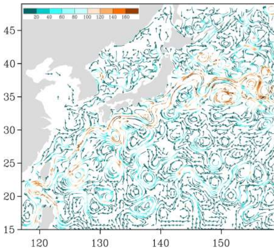
Рис. 3-5 Поверхностные течения западной части Тихого океана, 15 января 2021 г.
