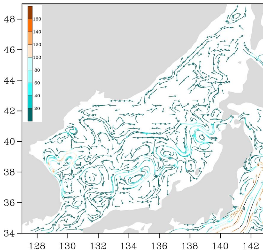
Рис. 3-1 Поверхностные течения Японского моря, 05 апреля 2021 г.
