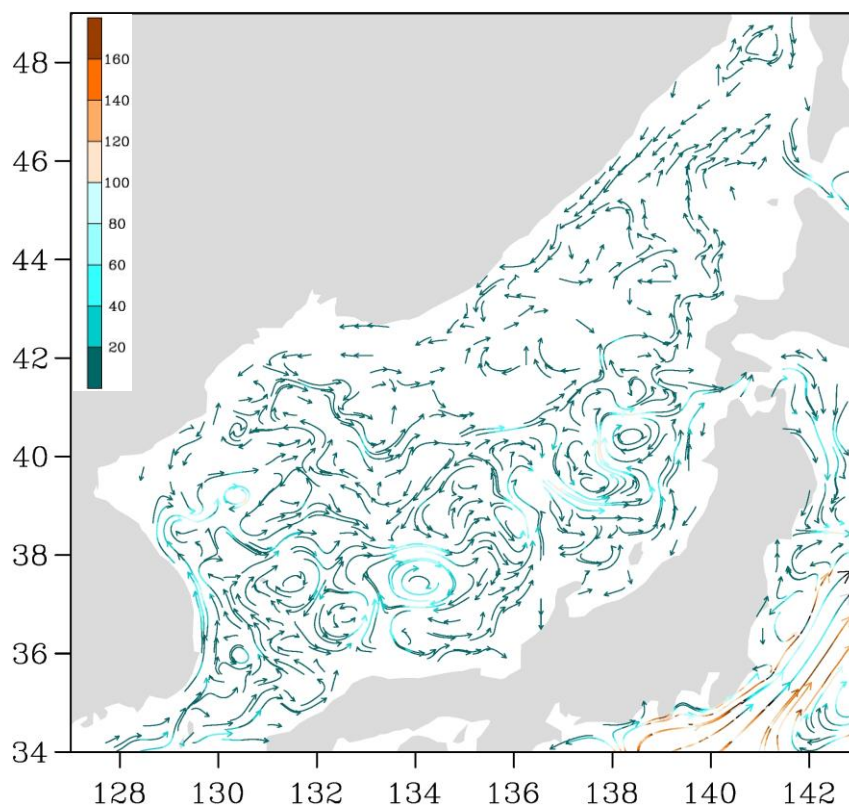
Рис. 3-3 Поверхностные течения Японского моря, 25 апреля 2021 г.
