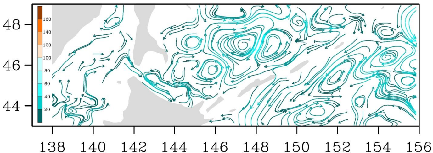
Рис. 3-7 Поверхностные течения, южная часть Охотского моря, 5 апреля 2021 г.
