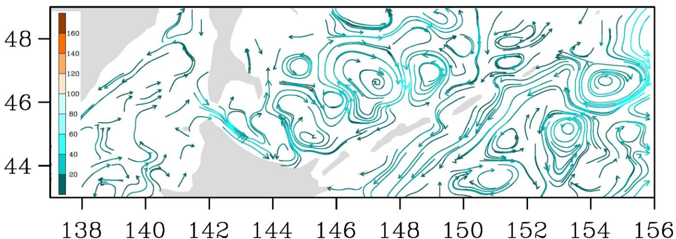
Рис. 3-8 Поверхностные течения, южная часть Охотского моря, 15 апреля 2021 г.
