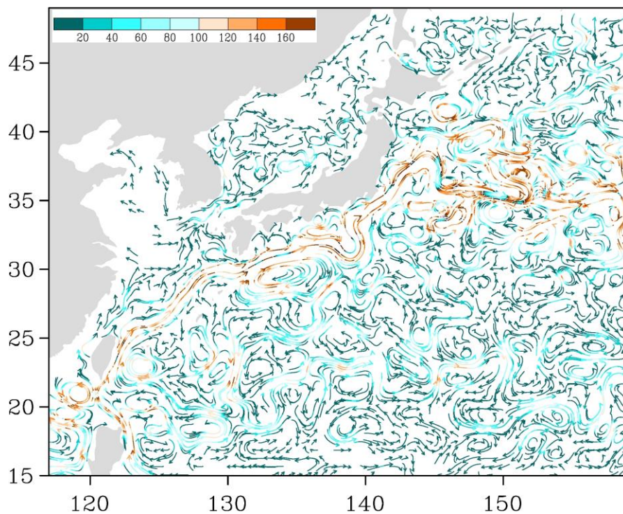
Рис. 3-5 Поверхностные течения западной части Тихого океана, 15 апреля 2021 г.
