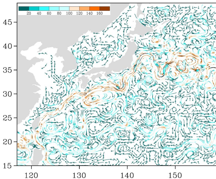
Рис. 3-4 Поверхностные течения западной части Тихого океана, 5 апреля 2021 г.
