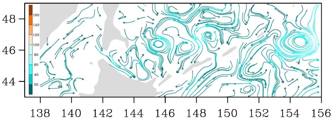
Рис. 3-9 Поверхностные течения, южная часть Охотского моря, 25 апреля 2021 г.
