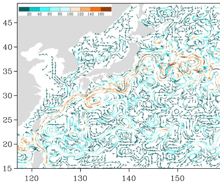
Рис. 3-6 Поверхностные течения западной части Тихого океана, 25 апреля 2021 г.
