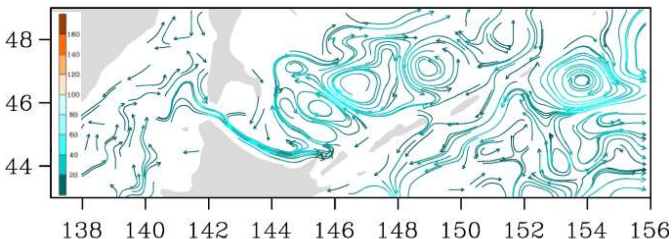
Рис. 3-8 Поверхностные течения, южная часть Охотского моря, 15 июня 2021 г.
