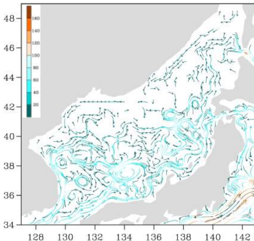
Рис. 3-1 Поверхностные течения Японского моря, 05 июня 2021 г.
