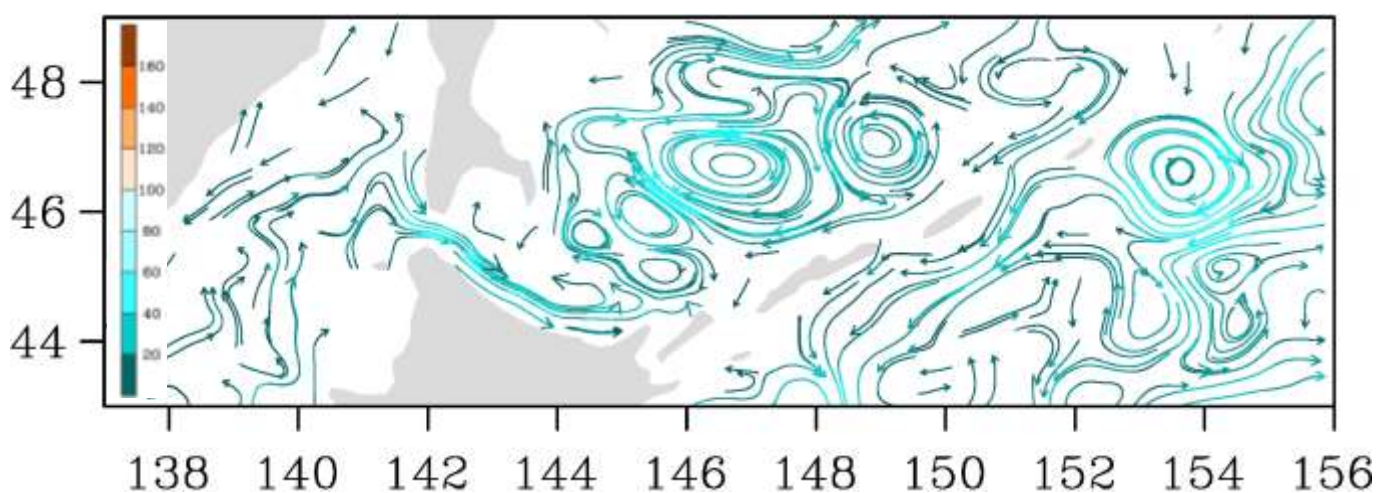
Рис. 3-9 Поверхностные течения, южная часть Охотского моря, 25 июня 2021 г.
