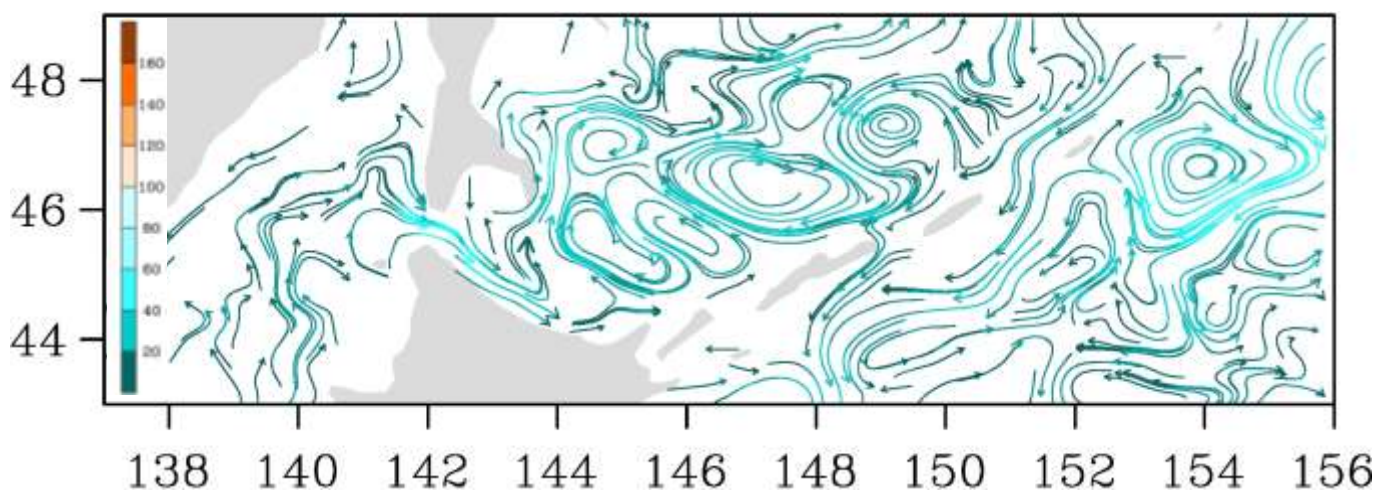
Рис. 3-7 Поверхностные течения, южная часть Охотского моря, 5 июня 2021 г.
