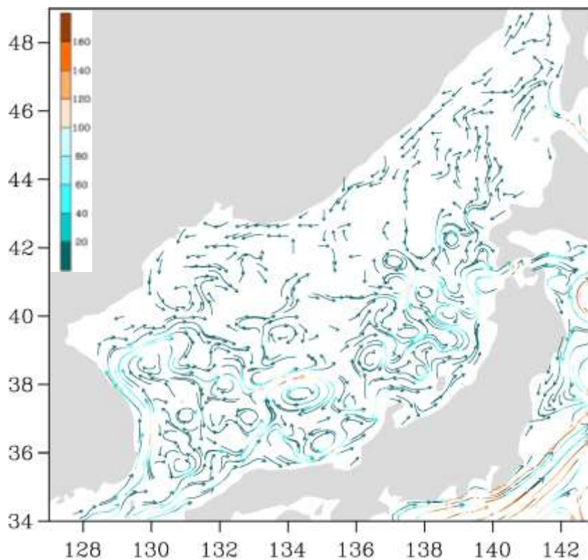
Рис. 3-2 Поверхностные течения Японского моря, 15 июня 2021 г.
