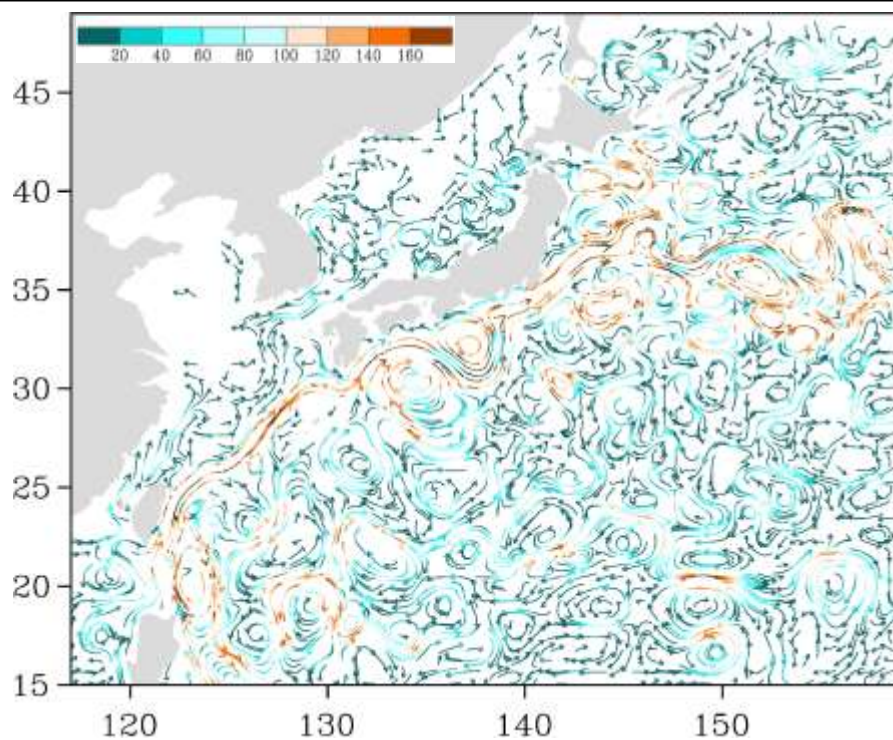
Рис. 3-5 Поверхностные течения западной части Тихого океана, 15 июня 2021 г.
