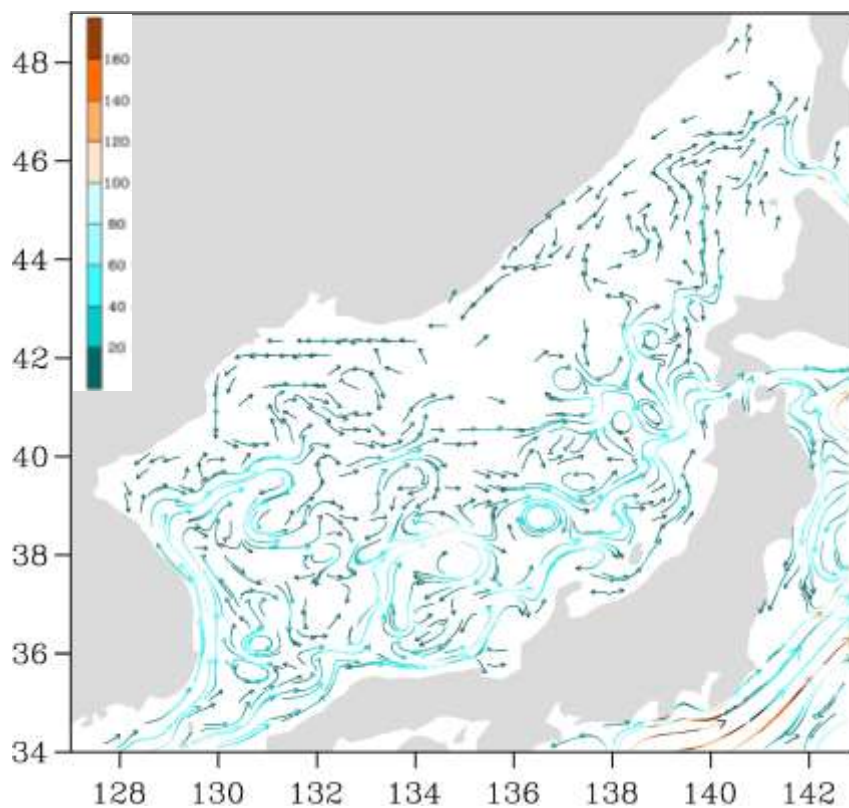
Рис. 3-3 Поверхностные течения Японского моря, 25 июня 2021 г.
