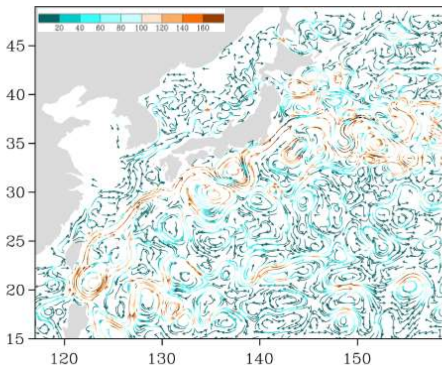
Рис. 3-6 Поверхностные течения западной части Тихого океана, 25 июня 2021 г.
