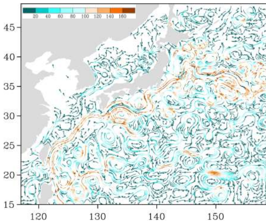
Рис. 3-4 Поверхностные течения западной части Тихого океана, 5 июня 2021 г.
