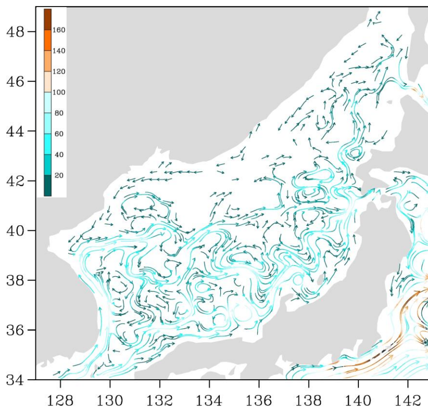
Рис. 3-3 Поверхностные течения Японского моря, 25 июля 2021 г.
