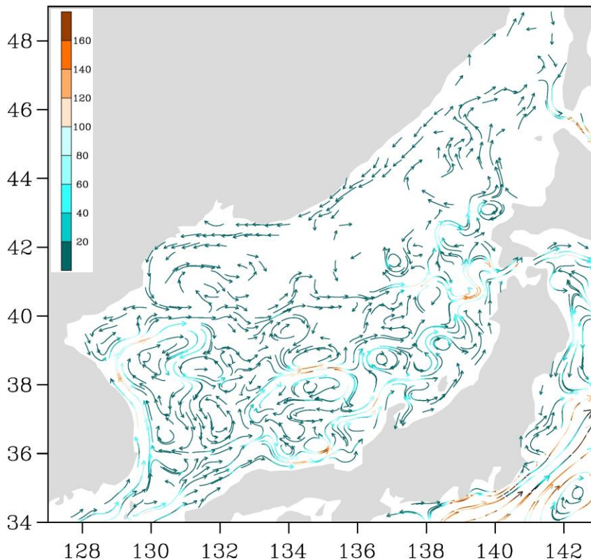
Рис. 3-1 Поверхностные течения Японского моря, 05 июля 2021 г.
