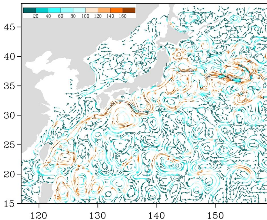
Рис. 3-5 Поверхностные течения западной части Тихого океана, 15 июля 2021 г.
