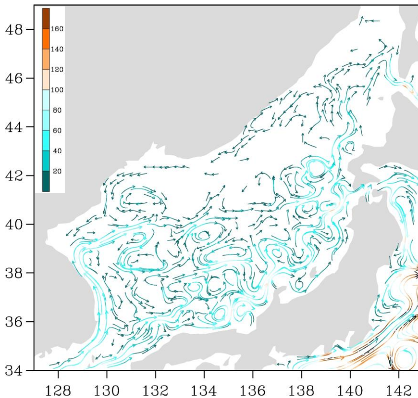
Рис. 3-2 Поверхностные течения Японского моря, 15 июля 2021 г.
