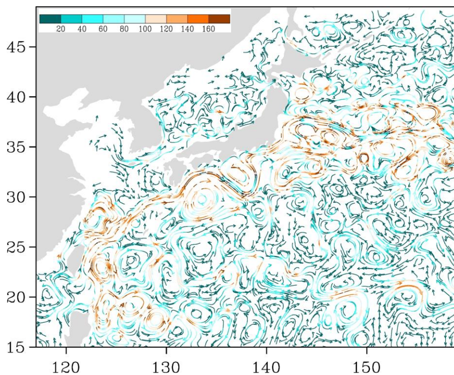
Рис. 3-6 Поверхностные течения западной части Тихого океана, 25 июля 2021 г.
