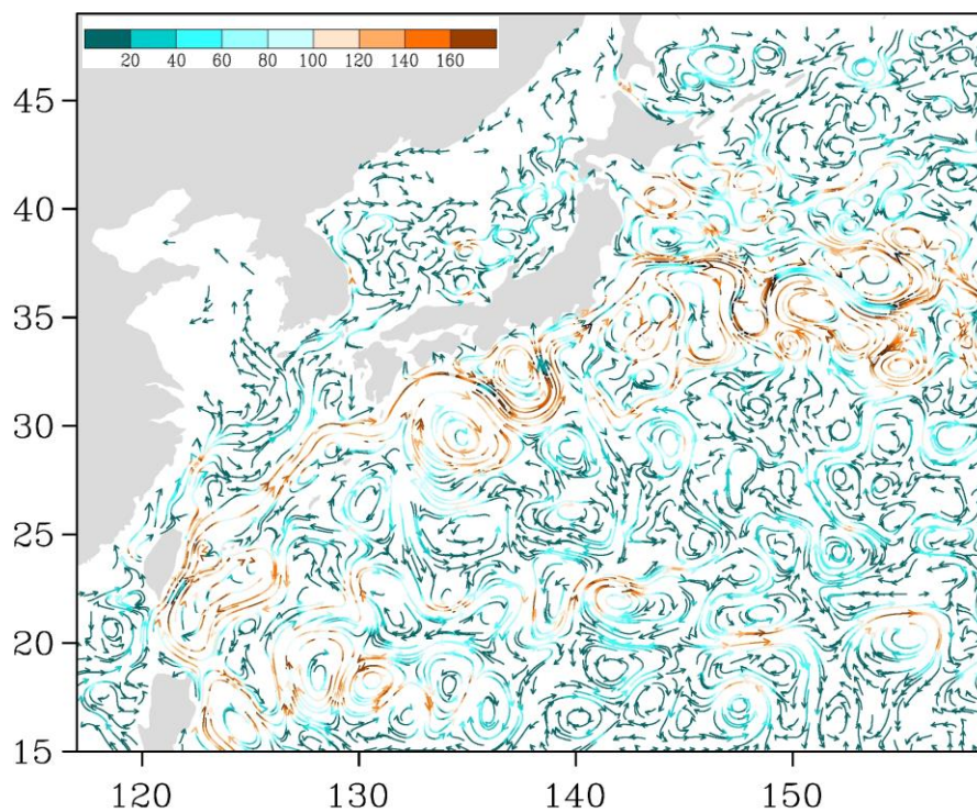
Рис. 3-4 Поверхностные течения западной части Тихого океана, 5 июля 2021 г.
