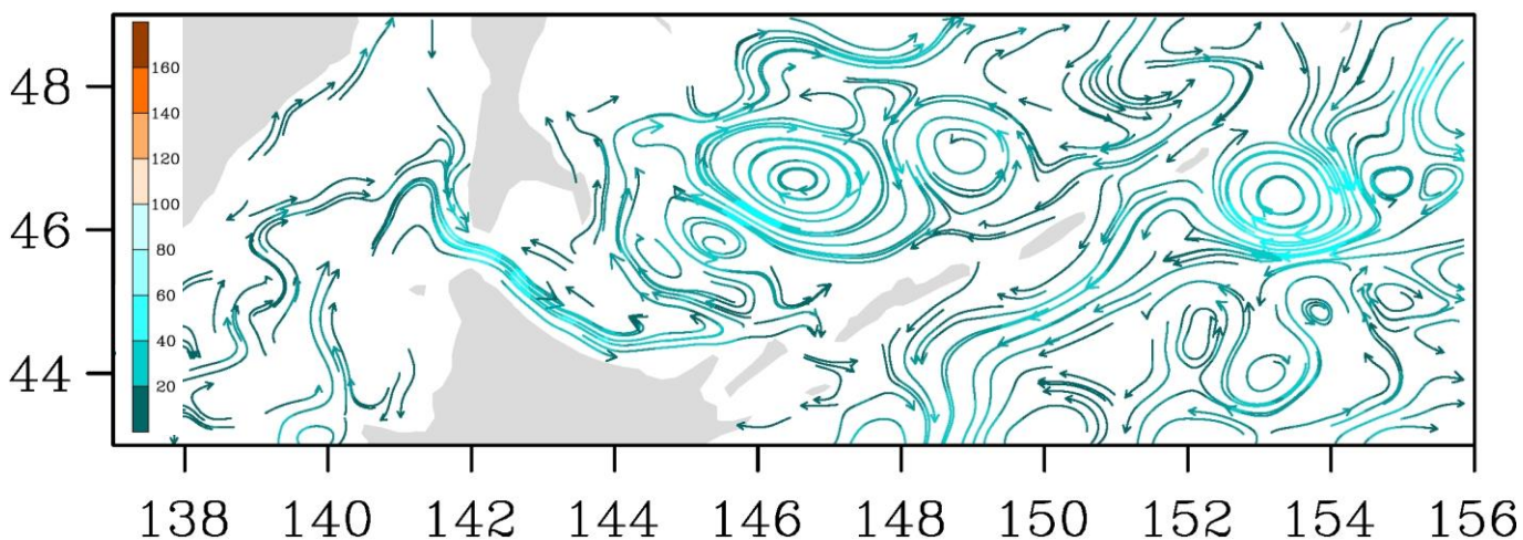
Рис. 3-7 Поверхностные течения, южная часть Охотского моря, 5 июля 2021 г.
