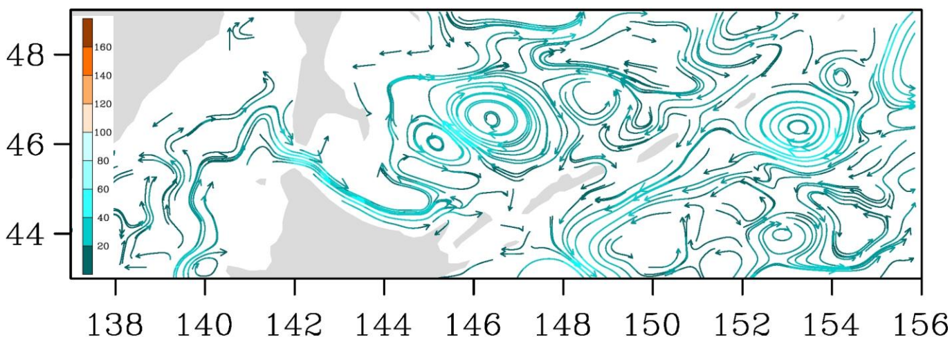
Рис. 3-8 Поверхностные течения, южная часть Охотского моря, 15 июля 2021 г.
