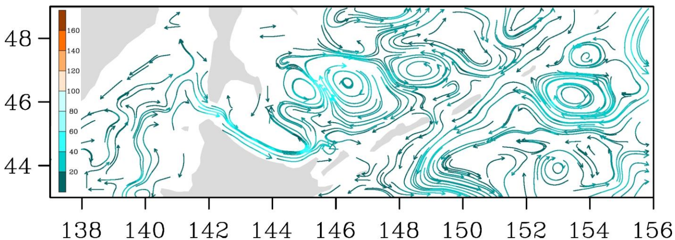
Рис. 3-9 Поверхностные течения, южная часть Охотского моря, 25 июля 2021 г.
