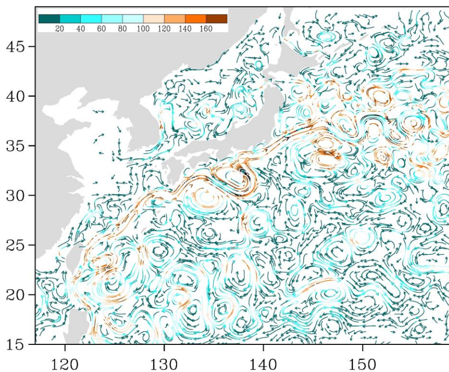
Рис. 3-6 Поверхностные течения западной части Тихого океана, 25 сентября 2021 г.
