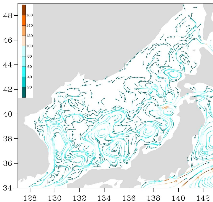
Рис. 3-2 Поверхностные течения Японского моря, 15 сентября 2021 г.
