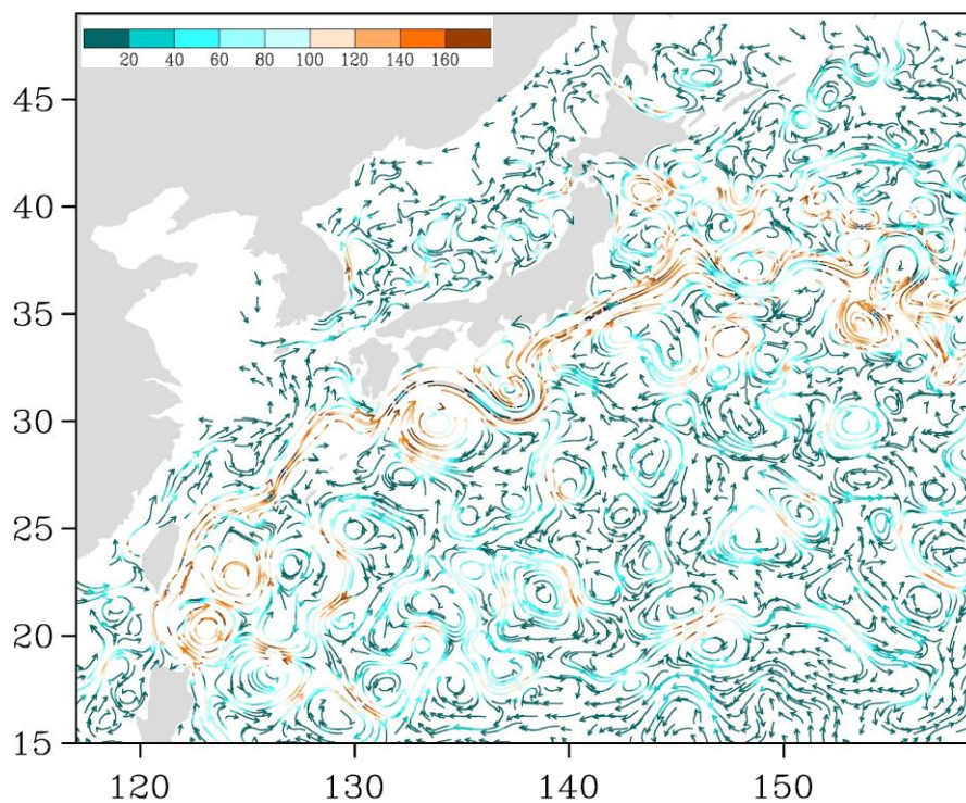
Рис. 3-4 Поверхностные течения западной части Тихого океана, 5 сентября 2021 г.
