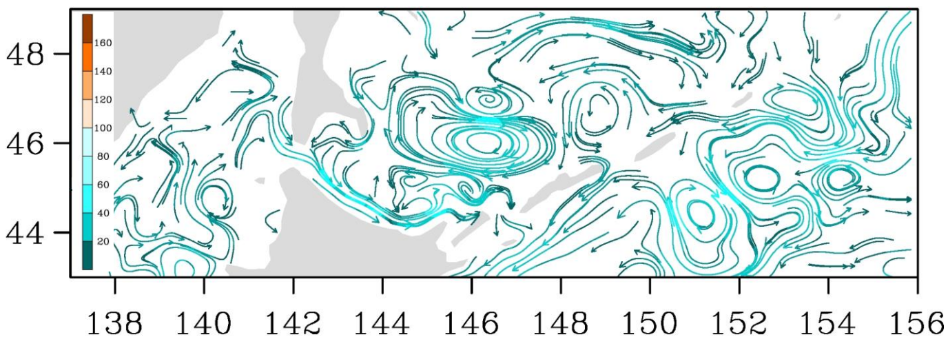
Рис. 3-9 Поверхностные течения, южная часть Охотского моря, 25 сентября 2021 г.
