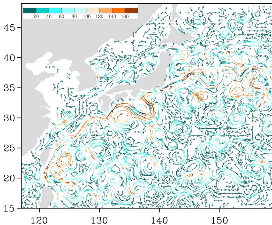
Рис. 3-5 Поверхностные течения западной части Тихого океана, 15 сентября 2021 г.
