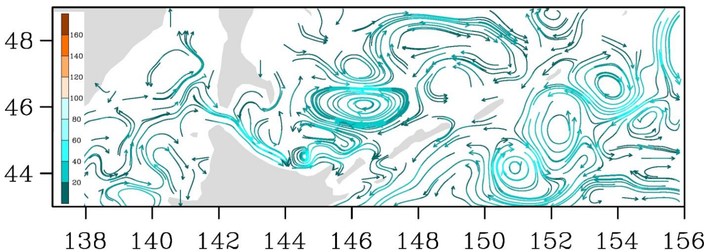
Рис. 3-8 Поверхностные течения, южная часть Охотского моря, 15 сентября 2021 г.
