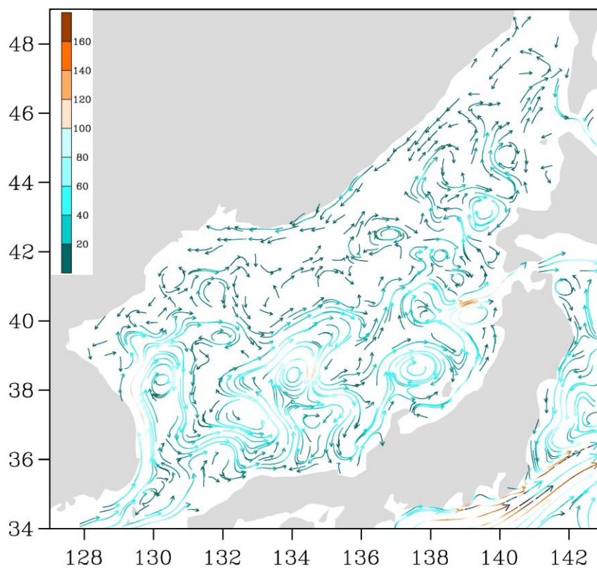
Рис. 3-3 Поверхностные течения Японского моря, 25 сентября 2021 г.
