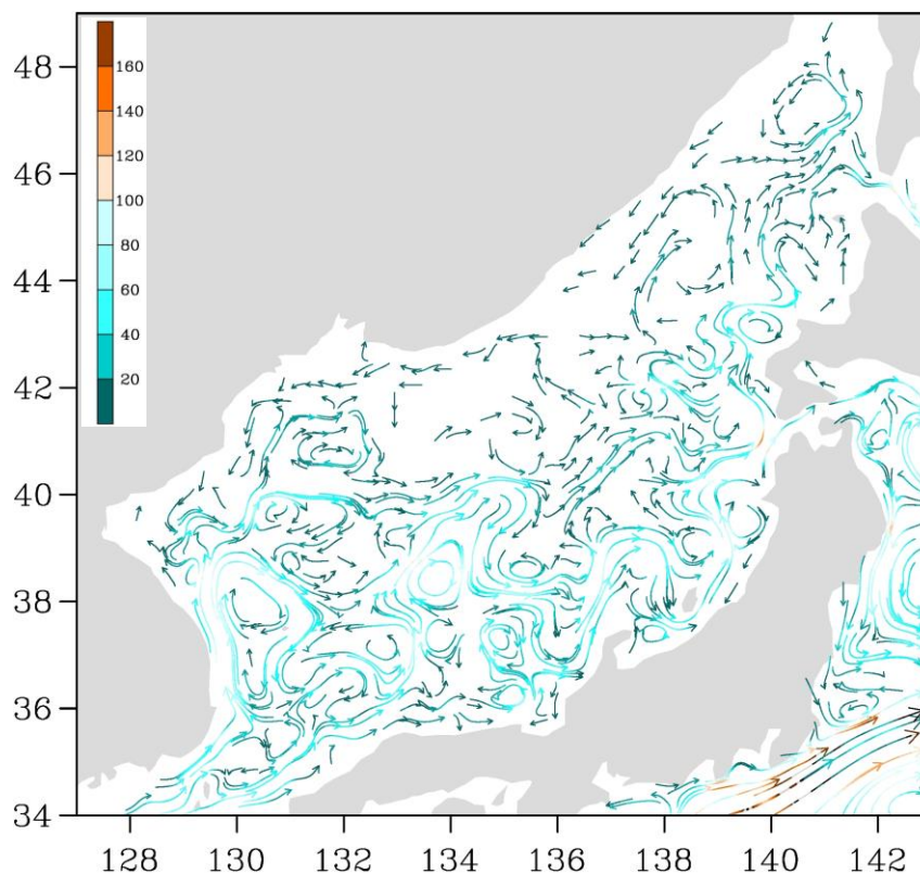
Рис. 3-1 Поверхностные течения Японского моря, 05 сентября 2021 г.
