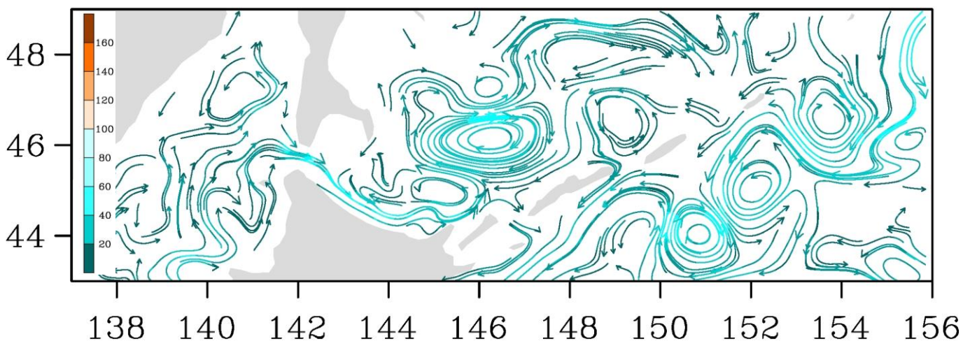
Рис. 3-7 Поверхностные течения, южная часть Охотского моря, 5 сентября 2021 г.
