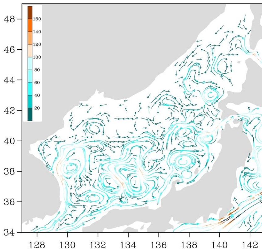
Рис. 3-1 Поверхностные течения Японского моря, 05 октября 2021 г.
