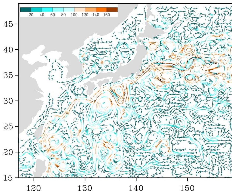
Рис. 3-6 Поверхностные течения западной части Тихого океана, 25 октября 2021 г.
