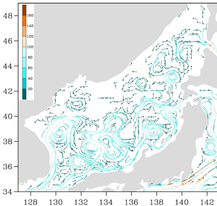
Рис. 3-2 Поверхностные течения Японского моря, 15 октября 2021 г.
