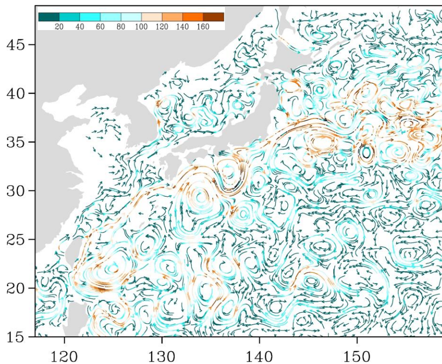
Рис. 3-5 Поверхностные течения западной части Тихого океана, 15 октября 2021 г.
