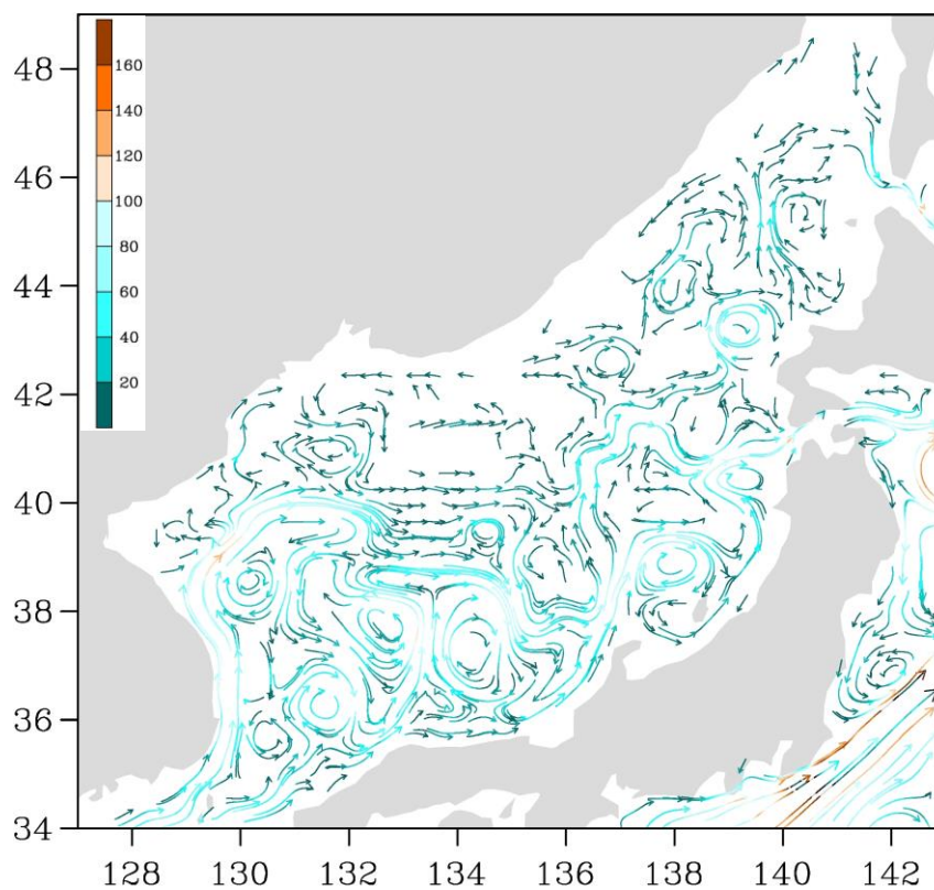
Рис. 3-3 Поверхностные течения Японского моря, 25 октября 2021 г.
