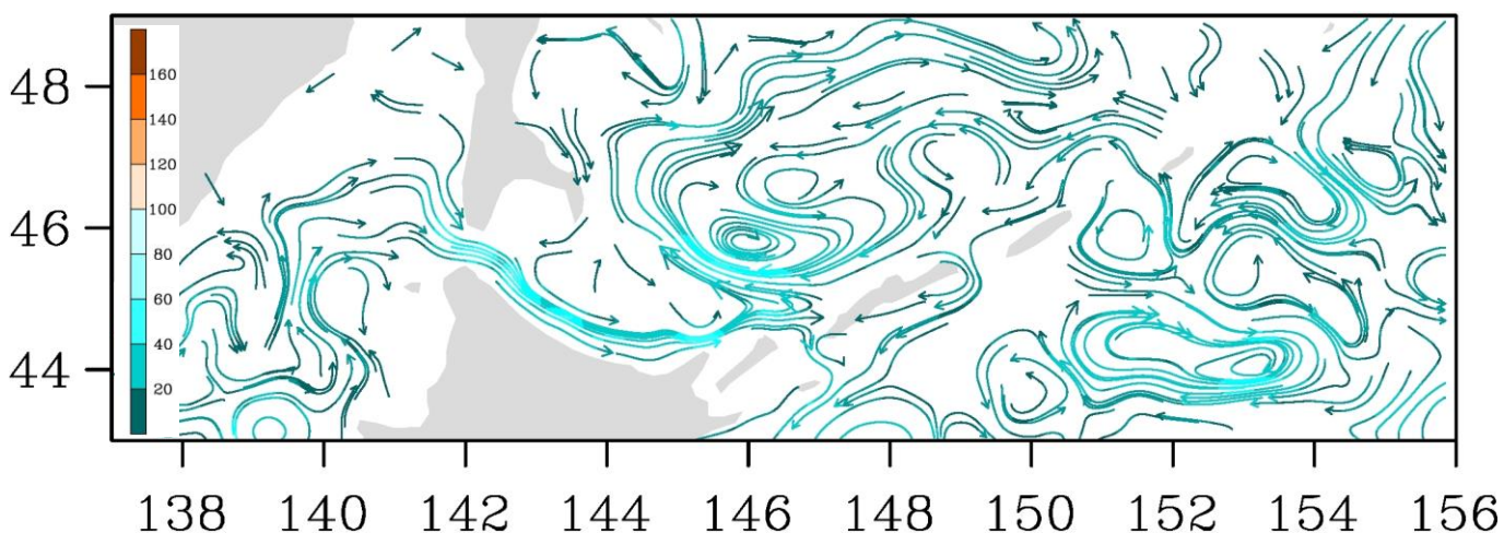
Рис. 3-8 Поверхностные течения, южная часть Охотского моря, 15 октября 2021 г.
