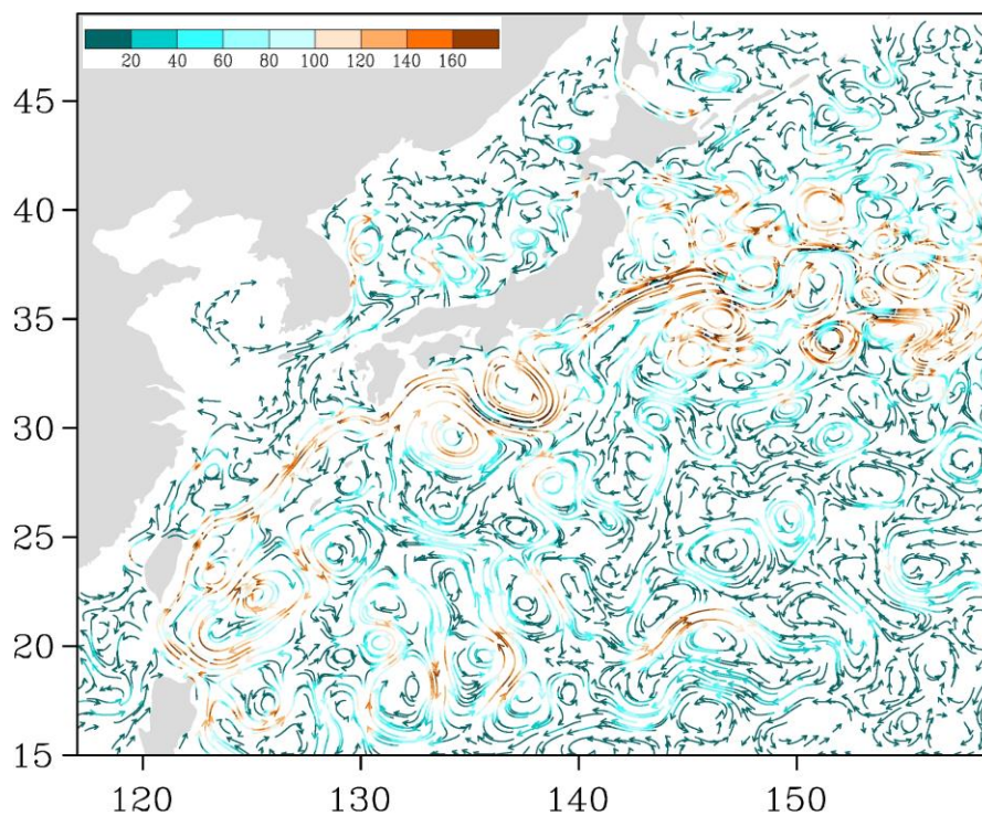
Рис. 3-4 Поверхностные течения западной части Тихого океана, 5 октября 2021 г.
