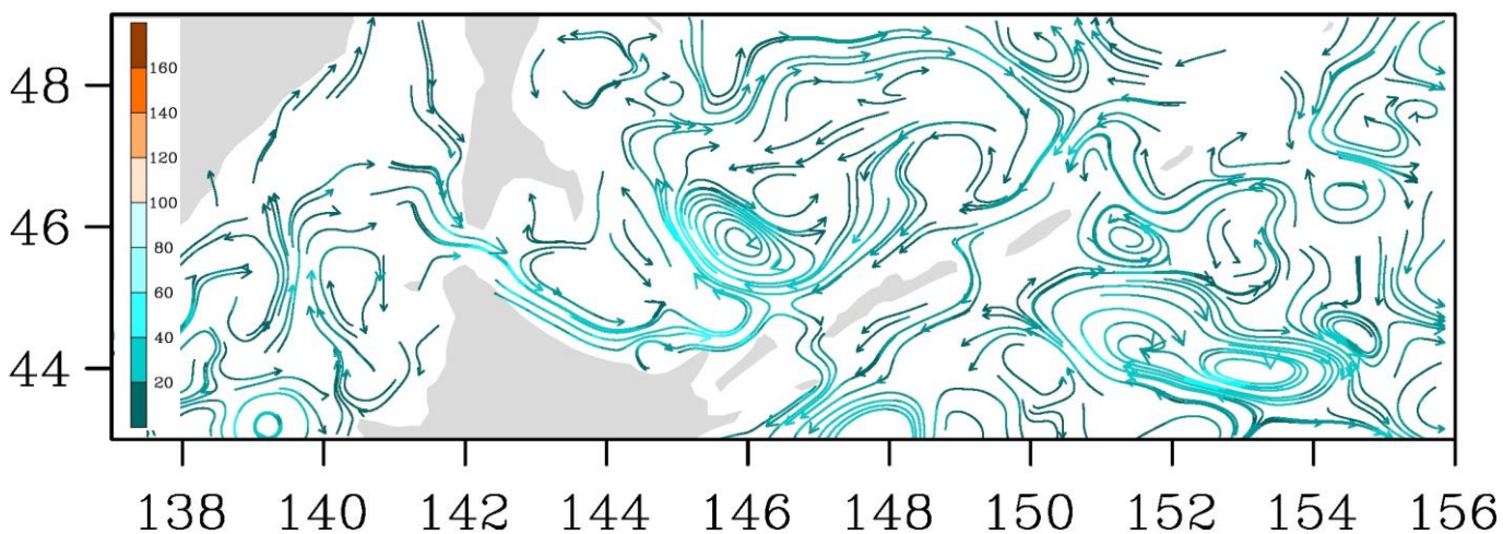
Рис. 3-9 Поверхностные течения, южная часть Охотского моря, 25 октября 2021 г.
