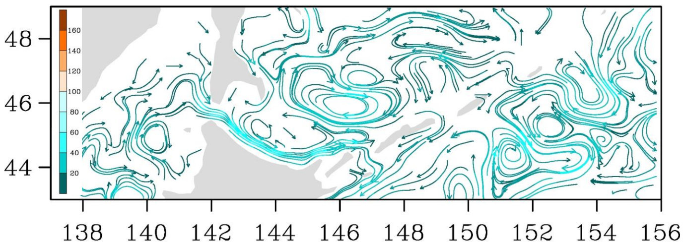
Рис. 3-7 Поверхностные течения, южная часть Охотского моря, 5 октября 2021 г.
