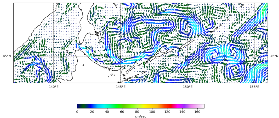
Рис. 3-9 Поверхностные течения, южная часть Охотского моря, 25 января 2025 г.
