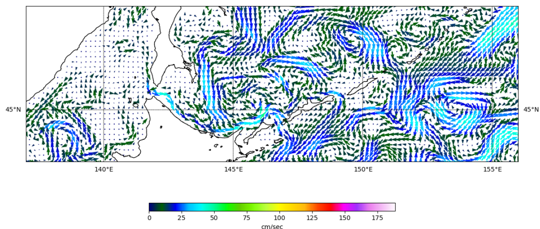
Рис. 3-7 Поверхностные течения, южная часть Охотского моря, 5 января 2025 г.
