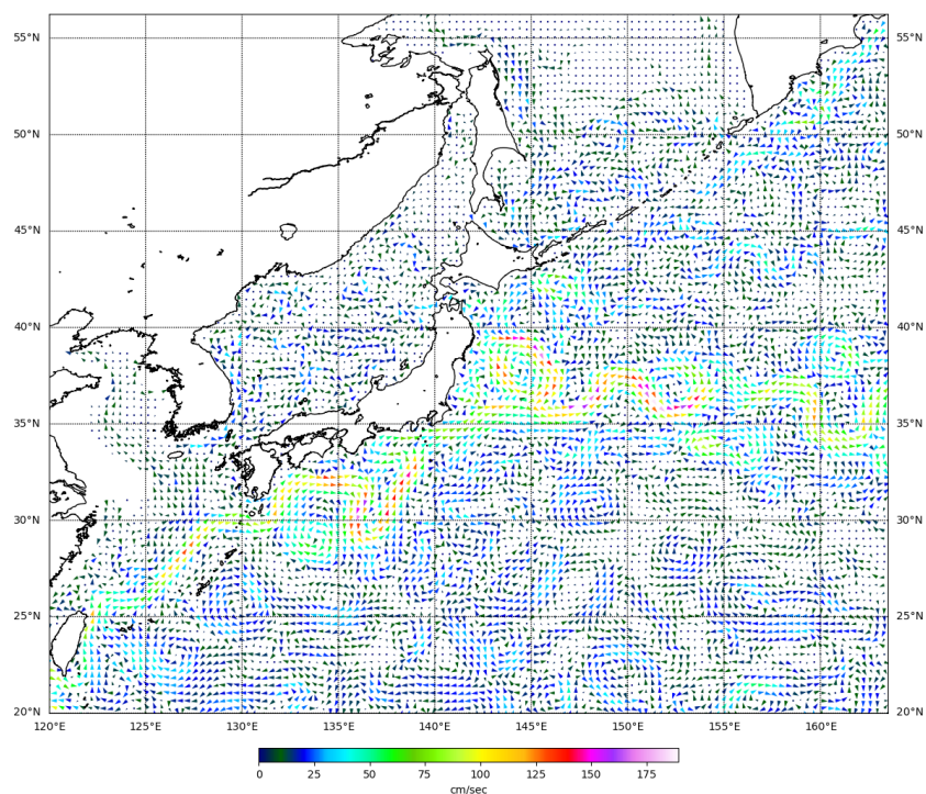
Рис. 3-5 Поверхностные течения западной части Тихого океана, 15 января 2025 г.
