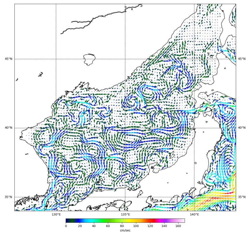
Рис. 3-3 Поверхностные течения Японского моря, 25 января 2025 г.
