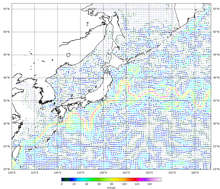
Рис. 3-6 Поверхностные течения западной части Тихого океана, 25 января 2025 г.
