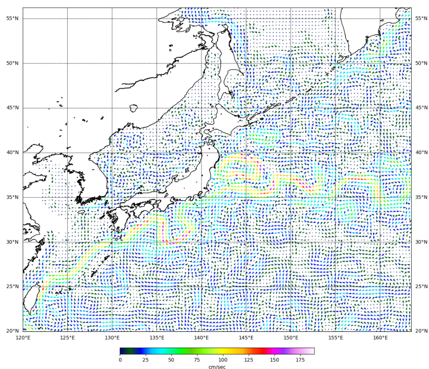
Рис. 3-4 Поверхностные течения западной части Тихого океана, 5 января 2025 г.
