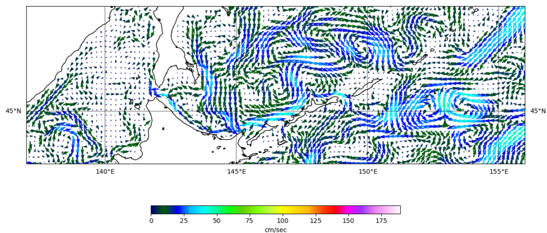
Рис. 3-8 Поверхностные течения, южная часть Охотского моря, 15 января 2025 г.
