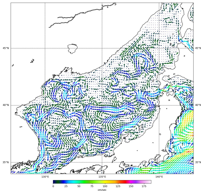
Рис. 3-1 Поверхностные течения Японского моря, 05 января 2025 г.
