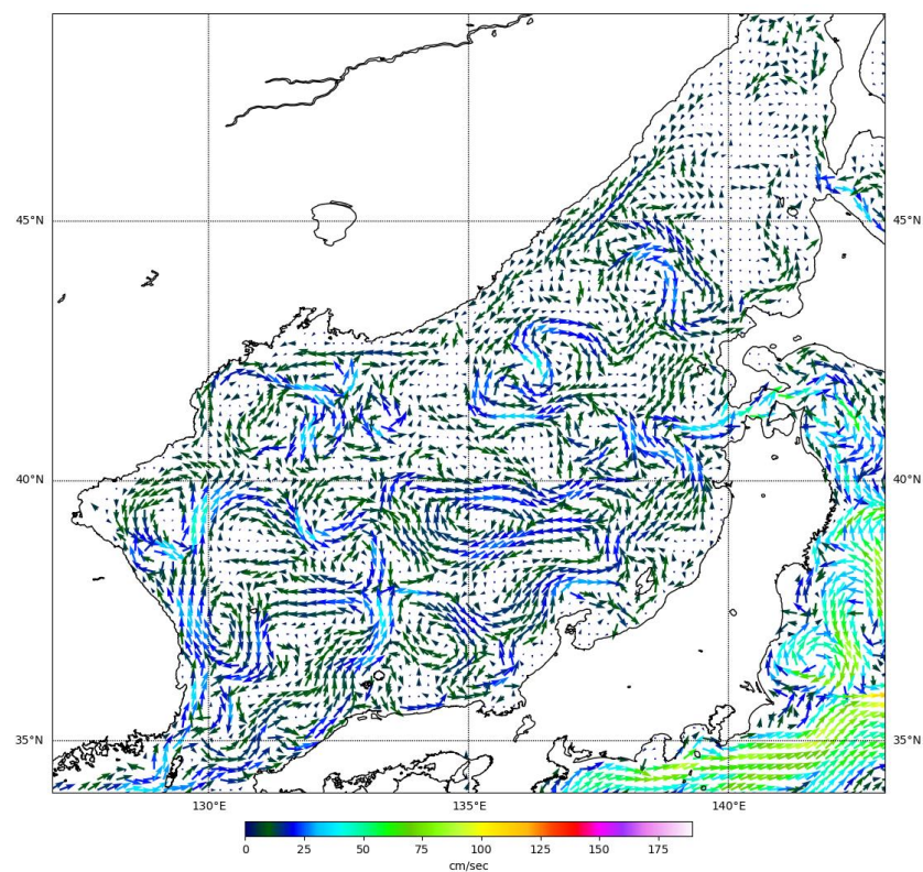
Рис. 3-2 Поверхностные течения Японского моря, 15 января 2025 г.
